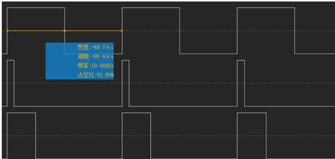
图 3.4.1 4 路独立输出波形
