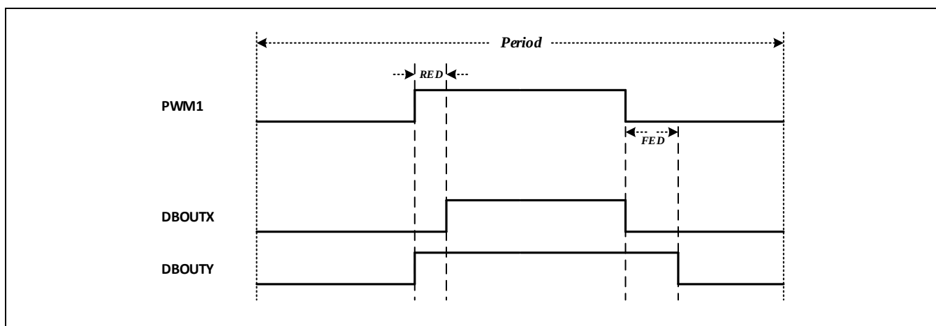
Figure 13-29 模式4: 高低电平有效死区输出举例
