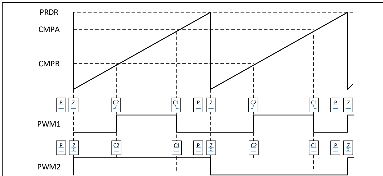
Figure 12-20 递增，脉冲定位非对称波形输出
