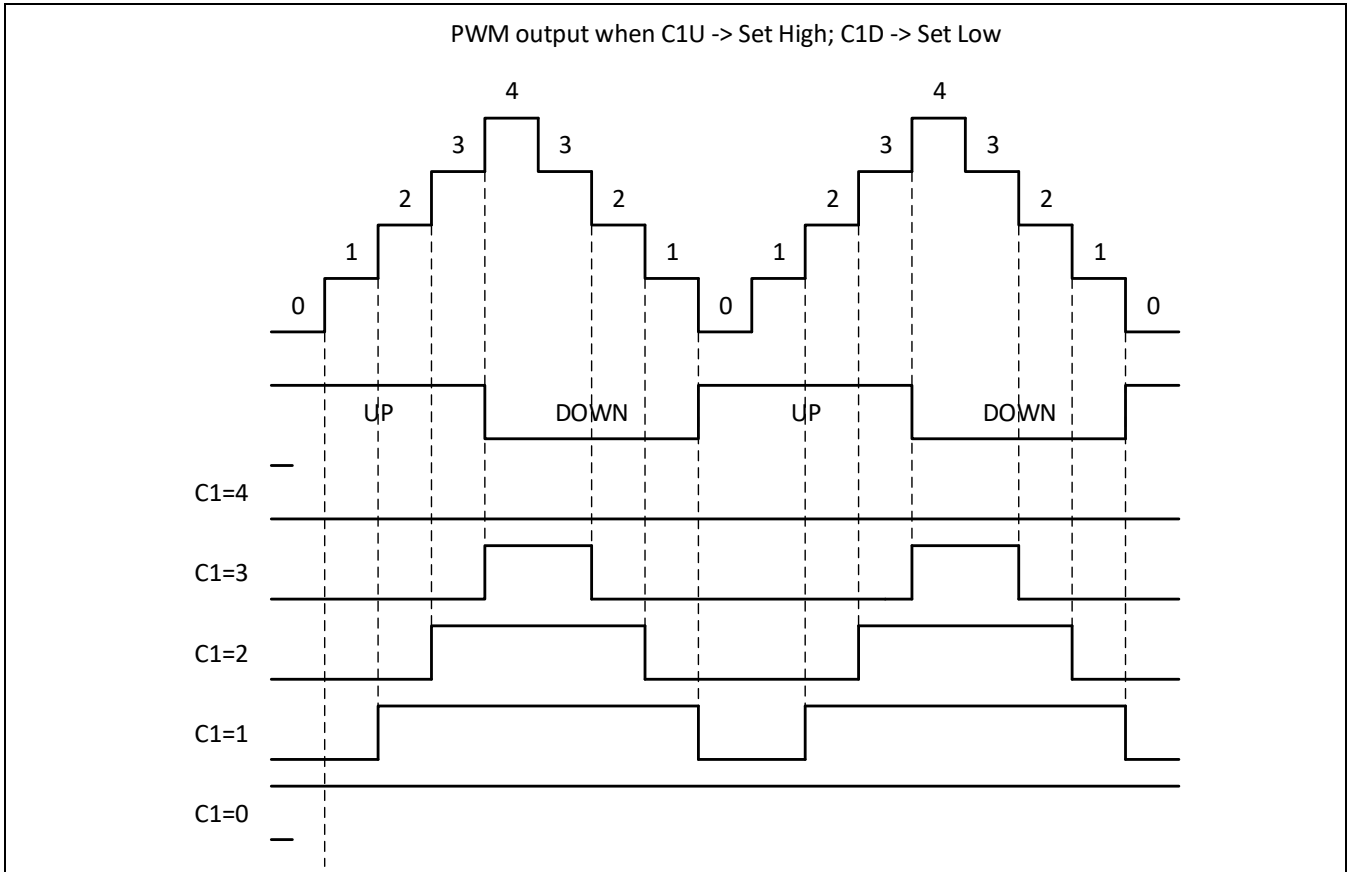
Figure 12-18 递增递减单比较值时，对称波形输出
