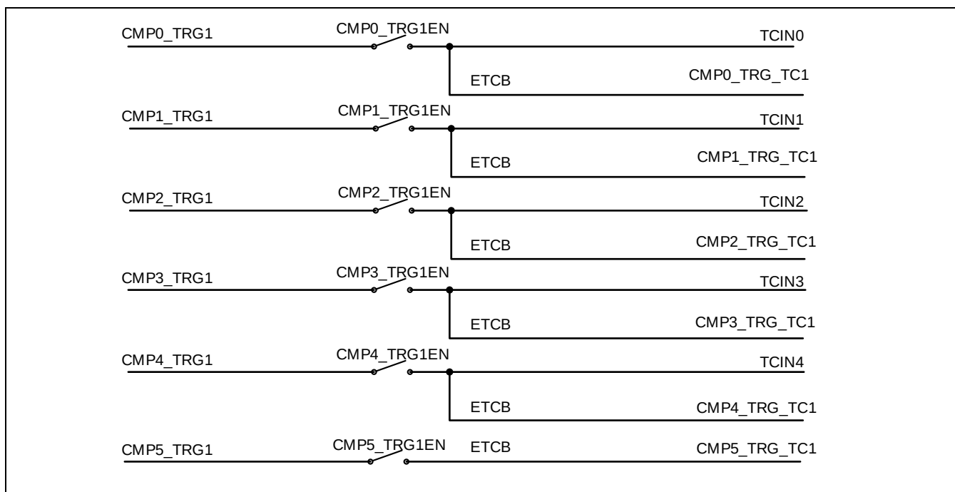
Figure 18-10 CMP 触发 TC1 的 Capture/CLK 输入及产生相关 ETCB 触发信号
