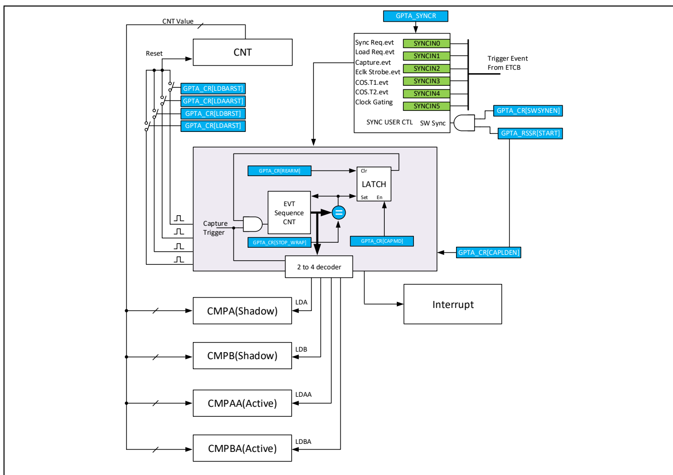
Figure 12-23 捕获模式结构框图
