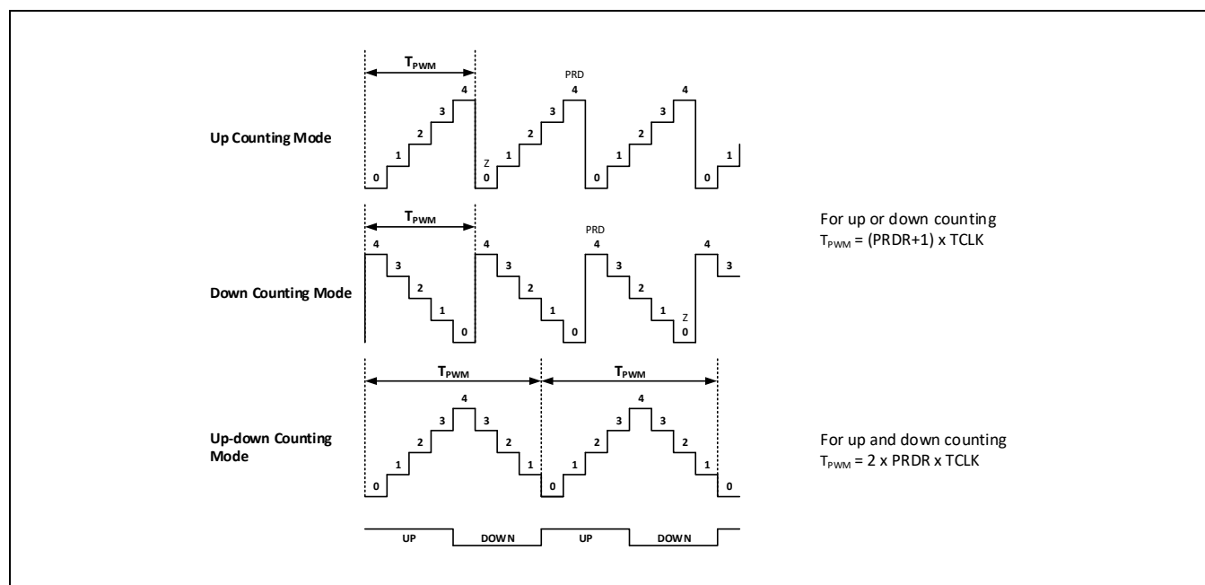
Figure 13-6 计数器工作模式
