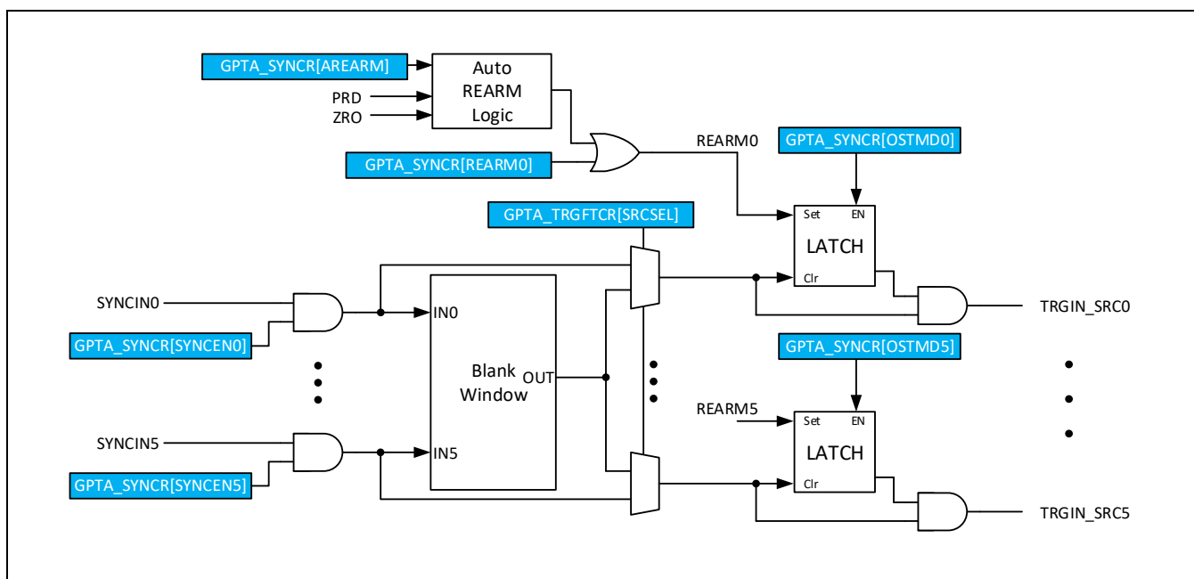
Figure 12-27 同步触发输入
