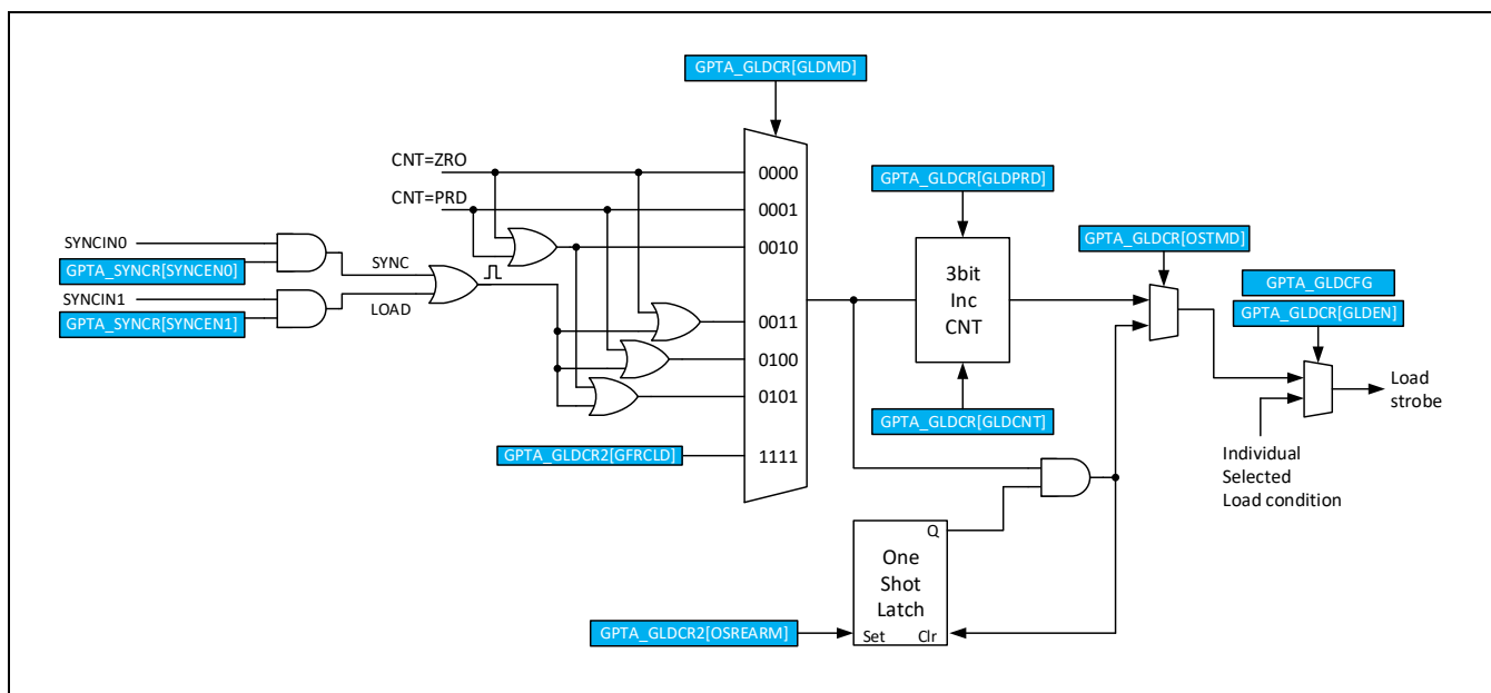
Figure 12-10 全局载入控制
