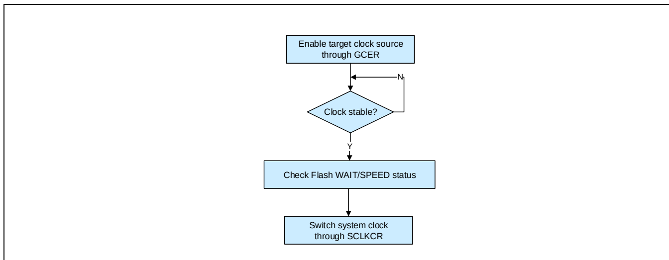
Figure 7-2 时钟源切换示意图
