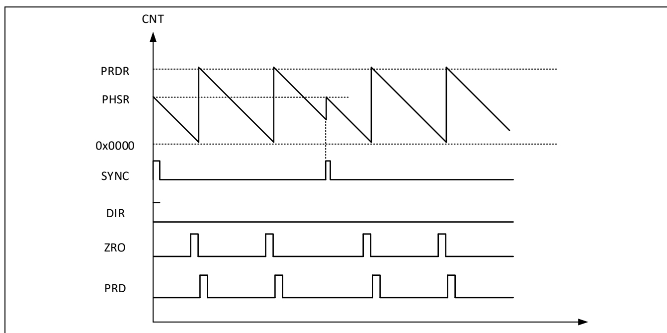
Figure 12-8 递减工作模式
