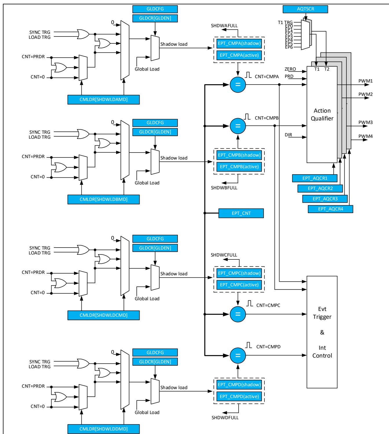
Figure 13-11 计数器值比较控制
