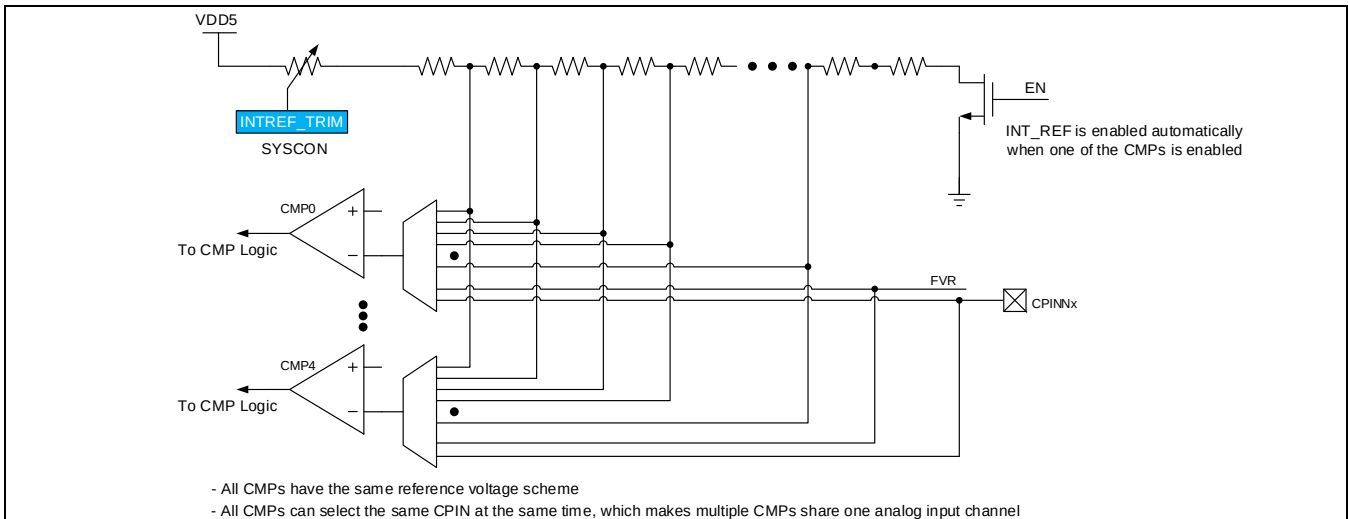
Figure 18-4 比较器内部参考电压
