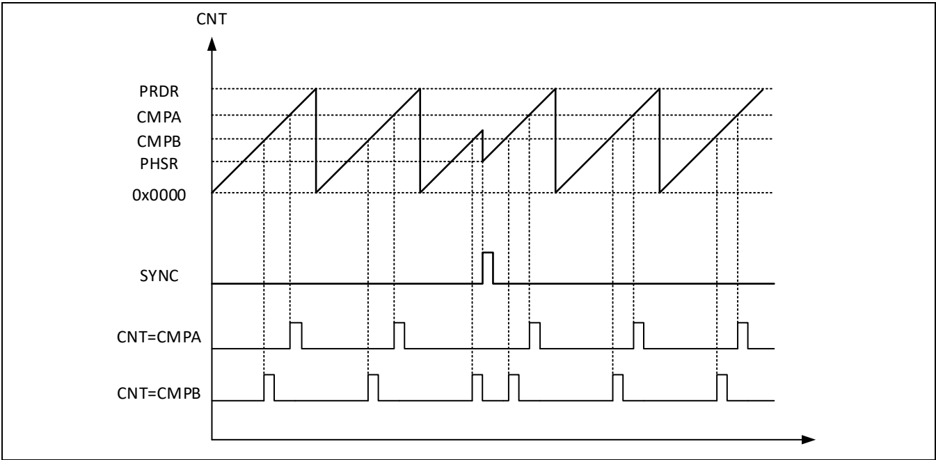
Figure 12-12 递增模式下比较事件产生时序
