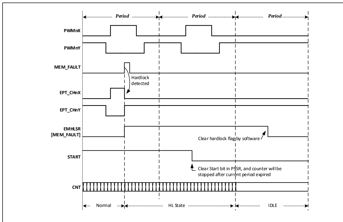
Figure 13-37 硬锁止模式
