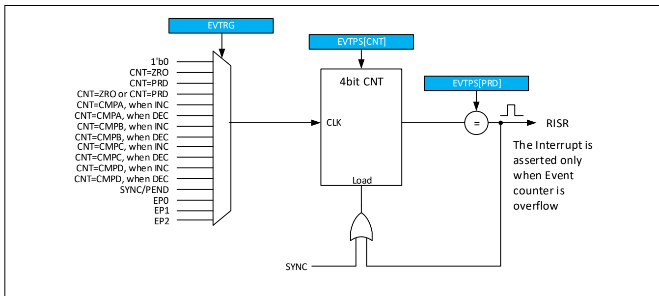
Figure 13-45 事件计数器
