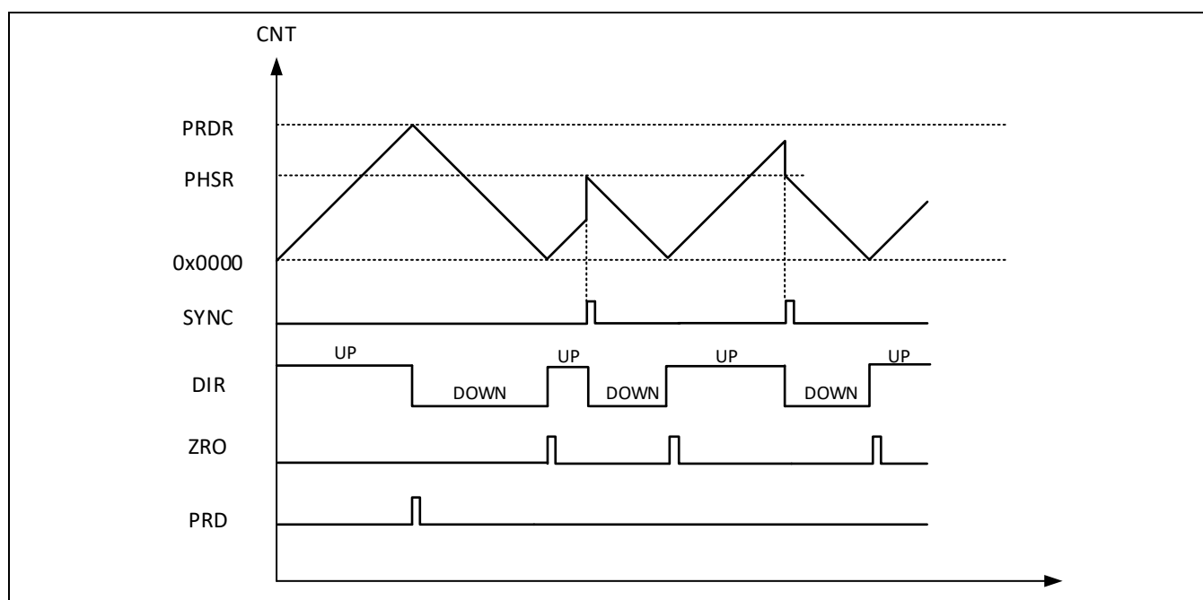
Figure 12-9 递增递减工作模式
