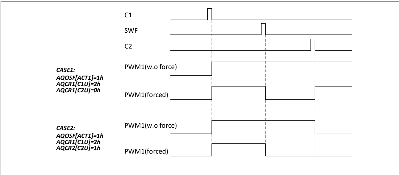
Figure 13-20 一次性软件强制输出
