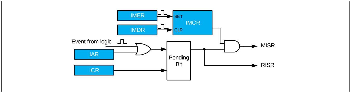
Figure 7-11 SYSCON 通用中断的控制逻辑
