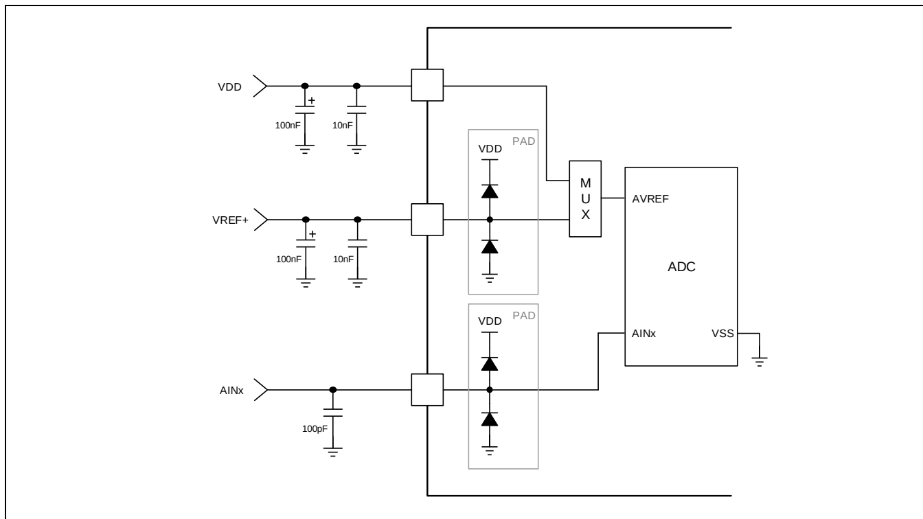
Figure 9-2 参考电路
