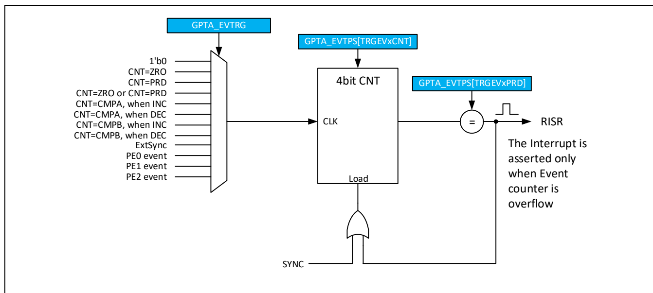
Figure 12-31 事件计数器
