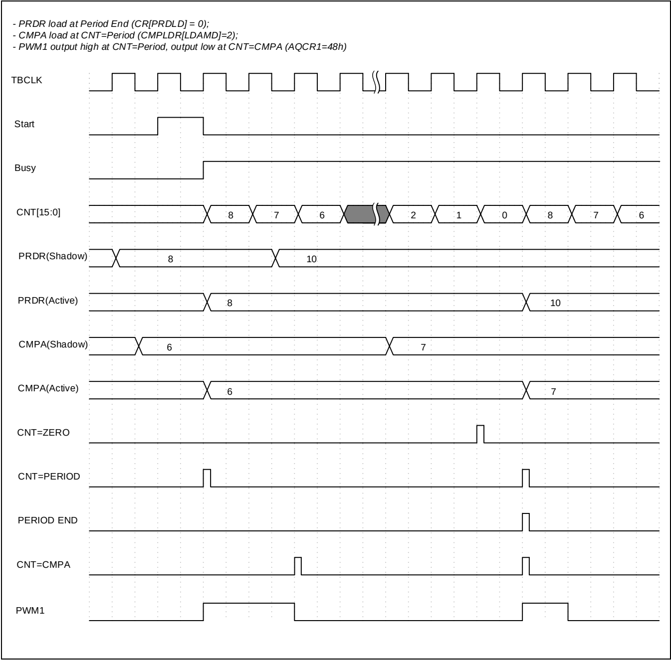
Figure 13-23 递减单比较值时，非对称波形输出
