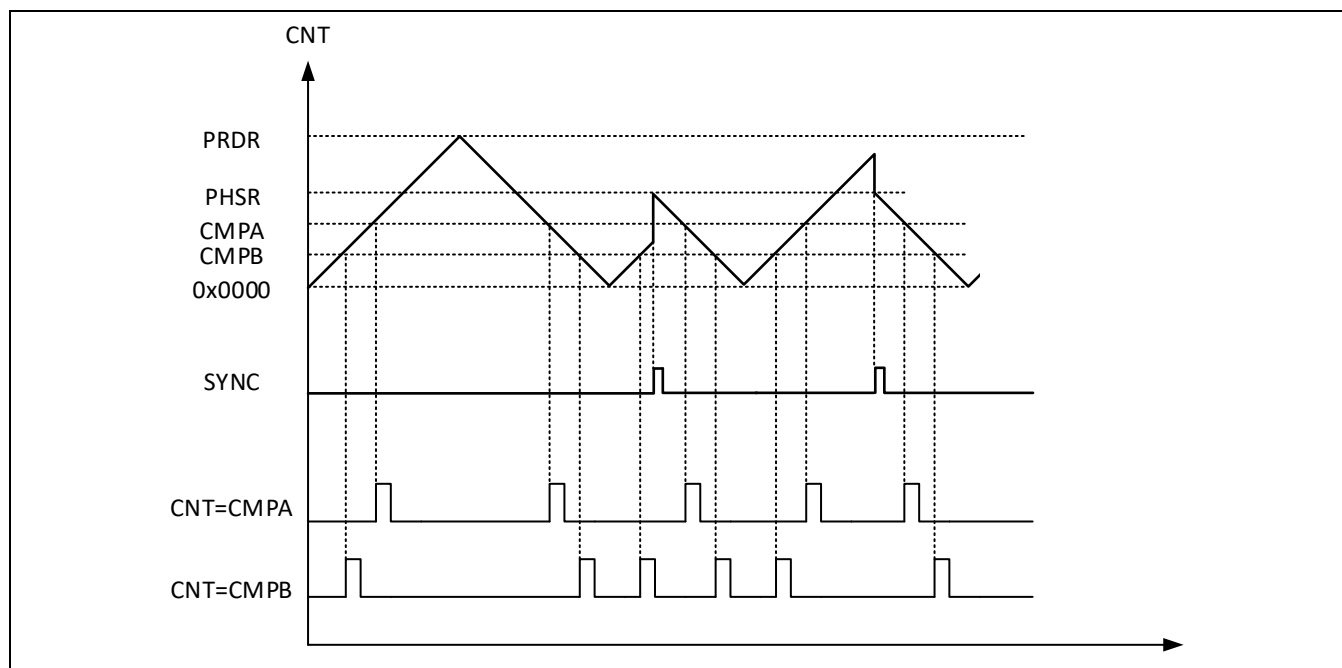
Figure 12-14 递增递减模式下比较事件产生时序
