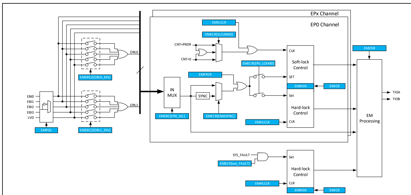
Figure 13-35 紧急模式控制模块
