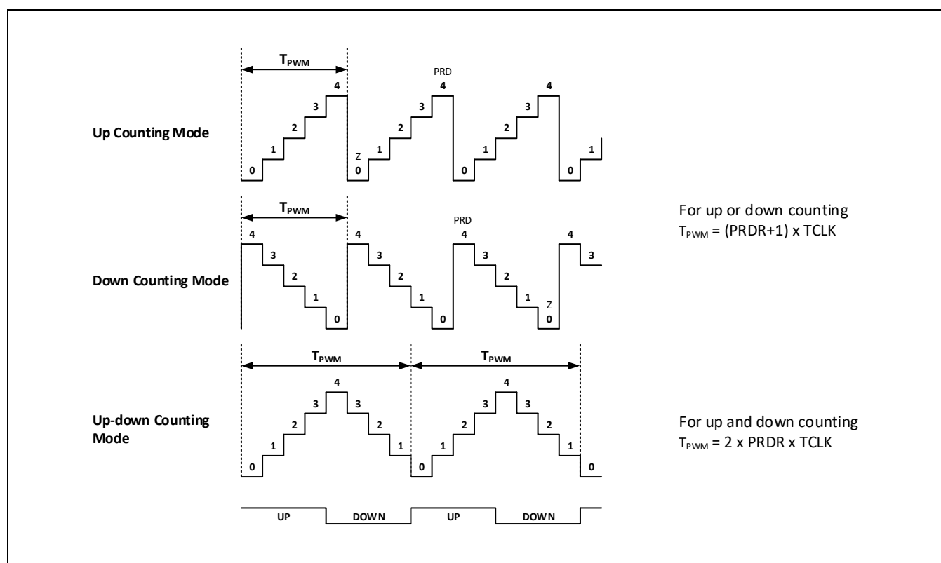
Figure 12-6 计数器工作模式
