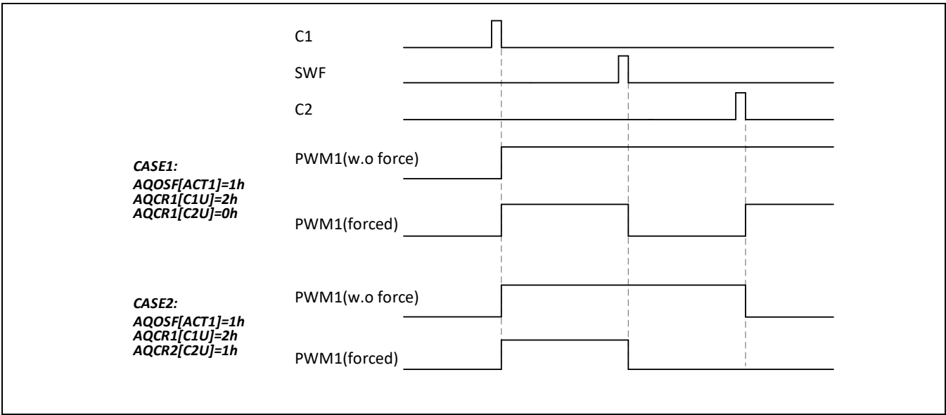
Figure 12-16 一次性软件强制输出
