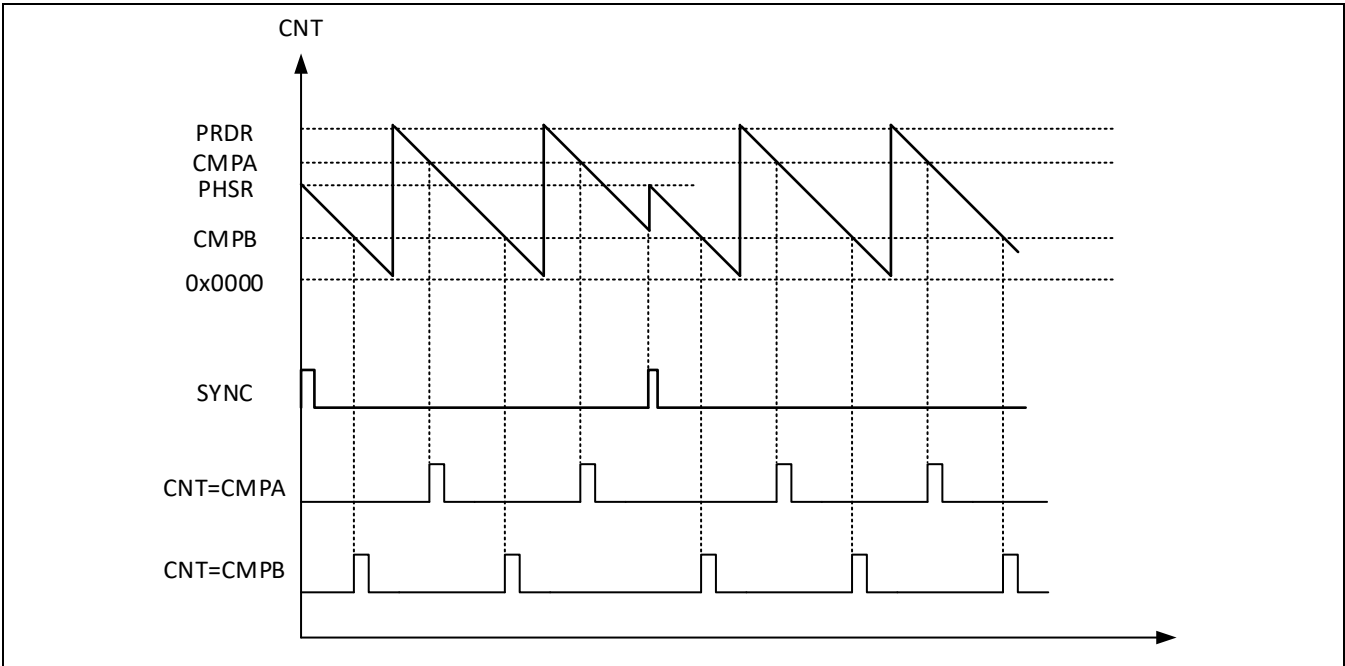
Figure 12-13 递减模式下比较事件产生时序
