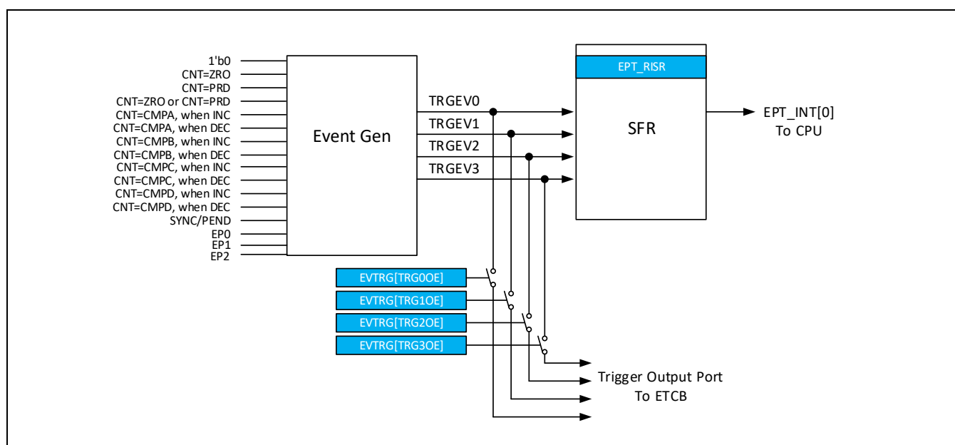
Figure 13-44 同步触发输出
