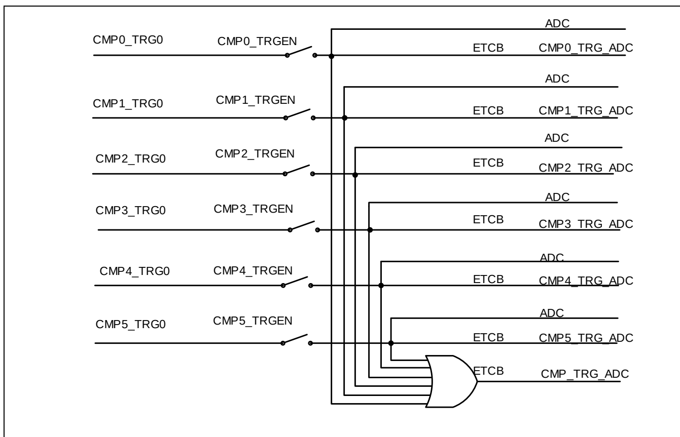
Figure 18-9 CMP 触发 ADC 及产生相关 ETCB 触发信号
