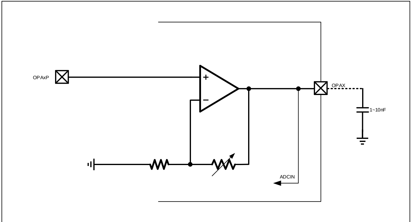
Figure 14-2 运算放大器作为 ADC 输入
