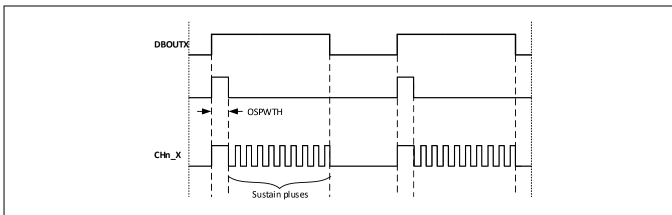
Figure 13-33 首脉冲扩展后的波形
