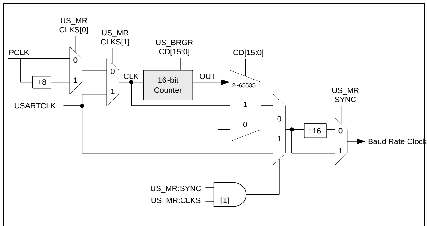
Figure 17-2 USART波特率发生器模块框图
