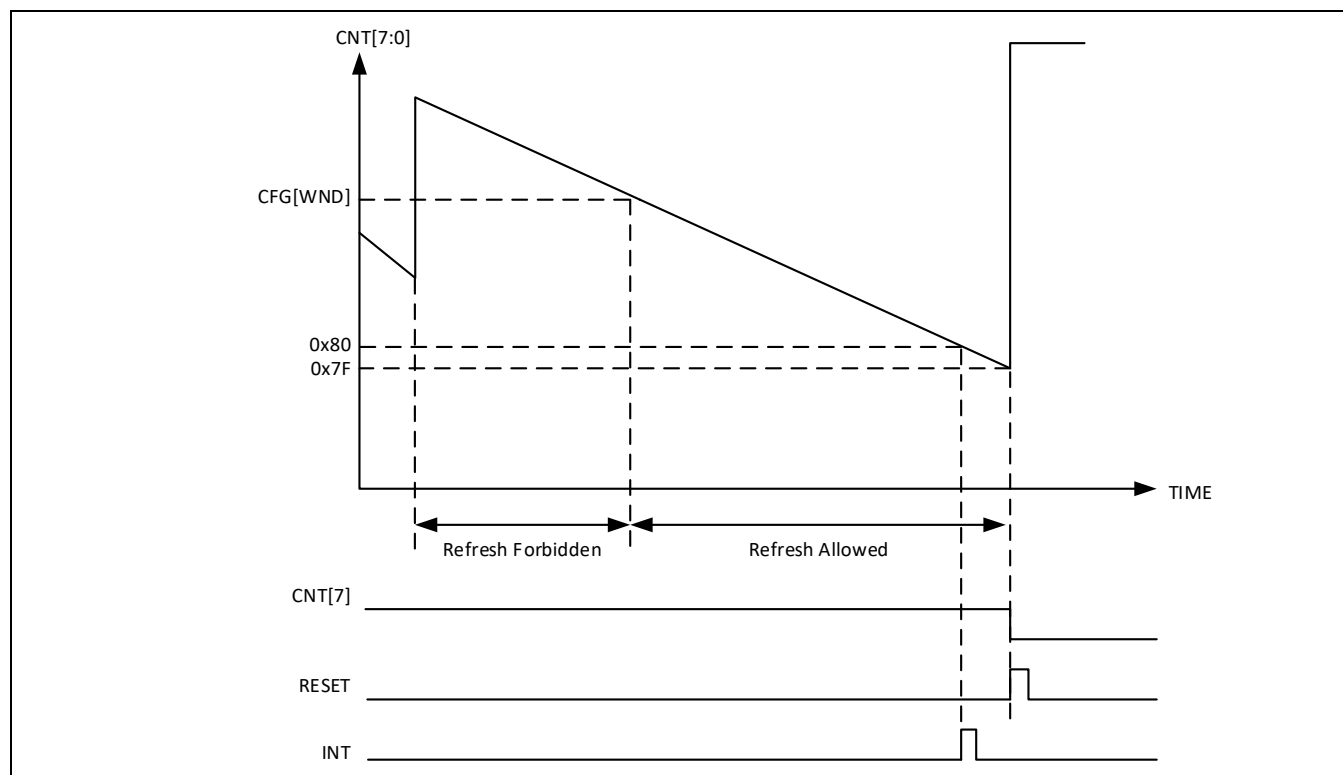
Figure 15-2 计数器工作示例
