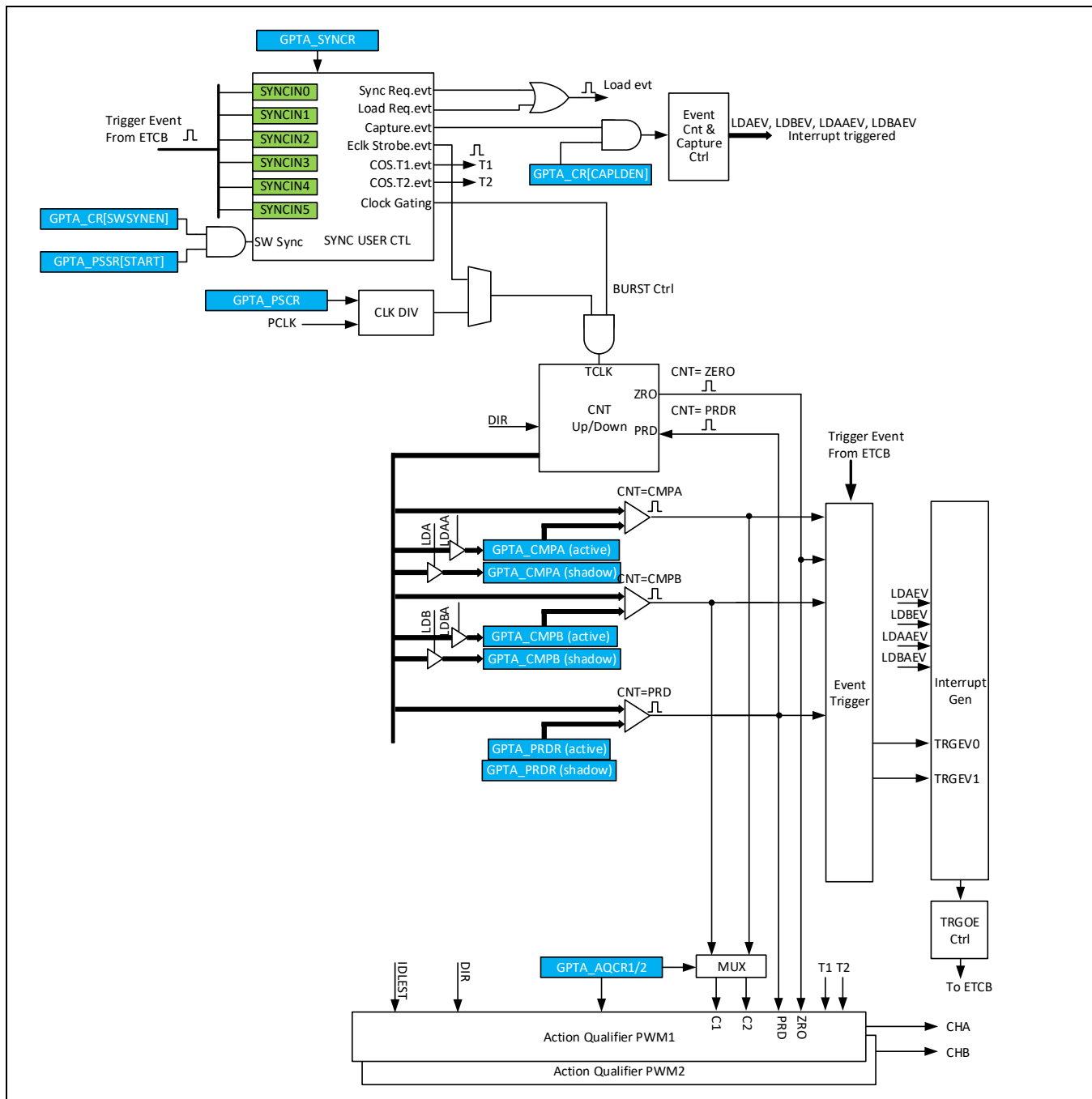
Figure 12-1 模块结构示意图
