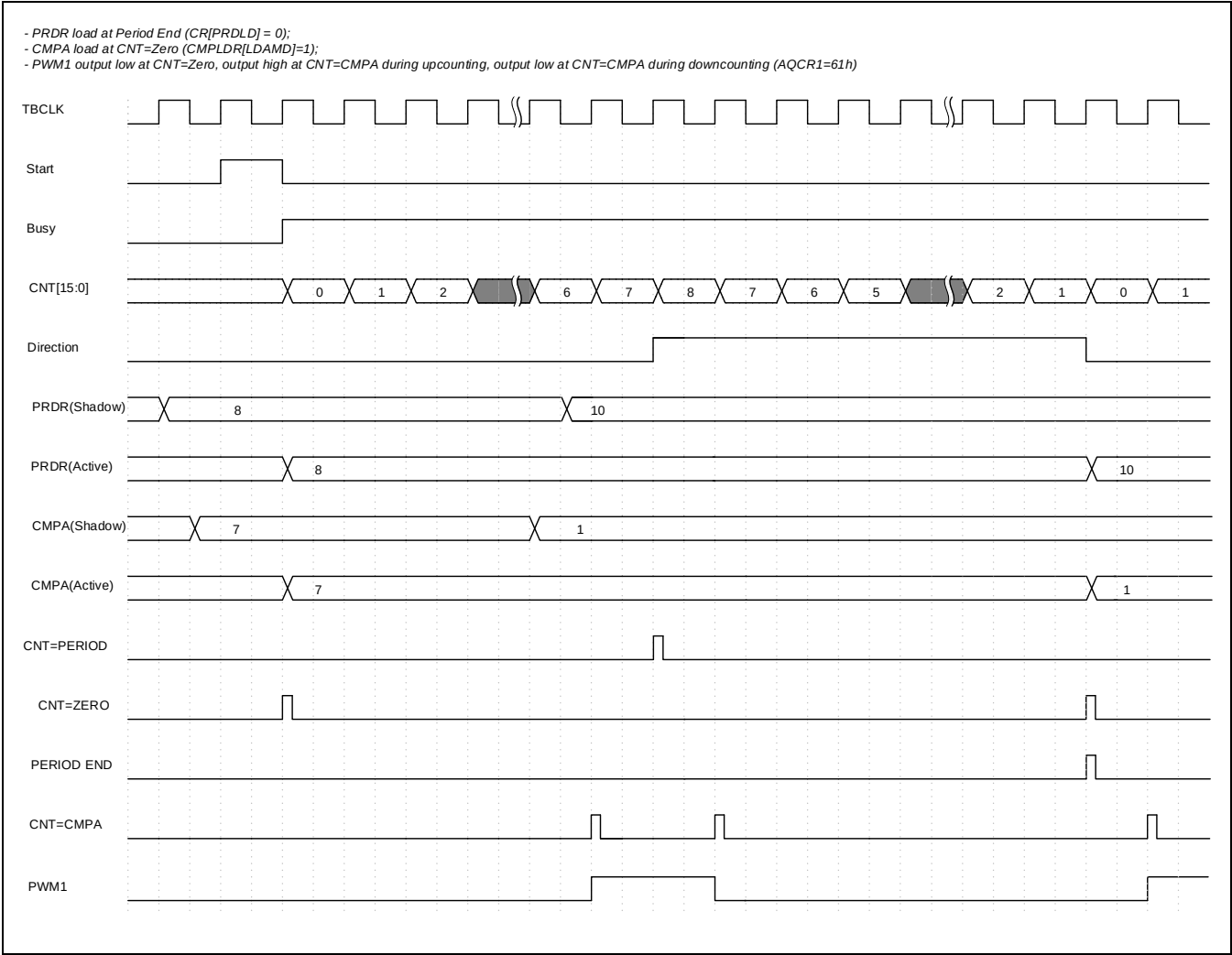
Figure 13-24 递增递减单比较值时，对称波形输出
