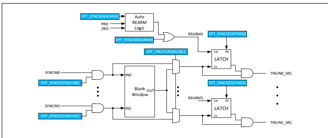
Figure 13-41 同步触发输入
