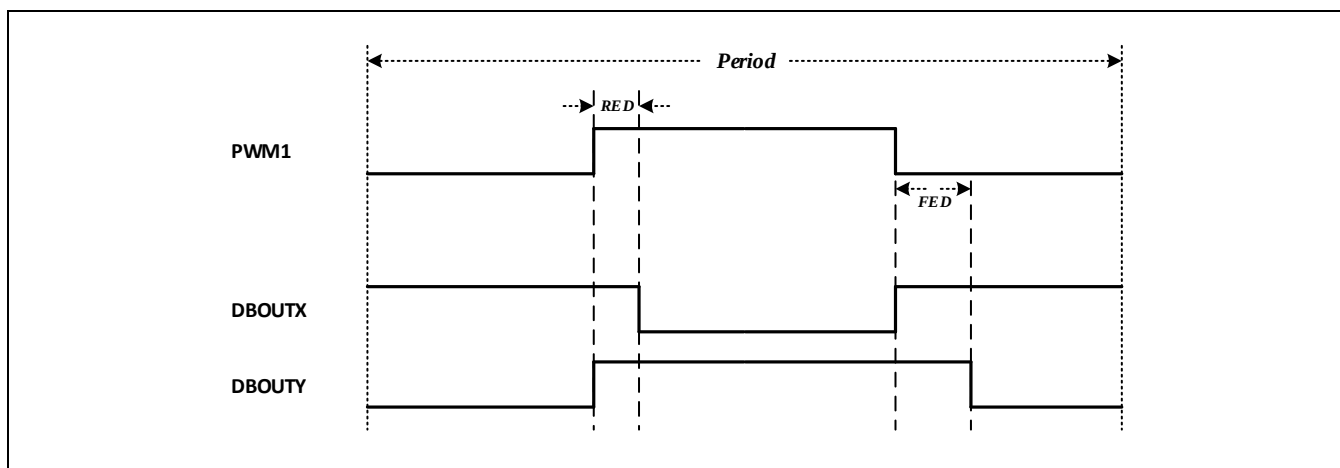
Figure 13-28 模式3: 低电平有效的死区互补输出举例
