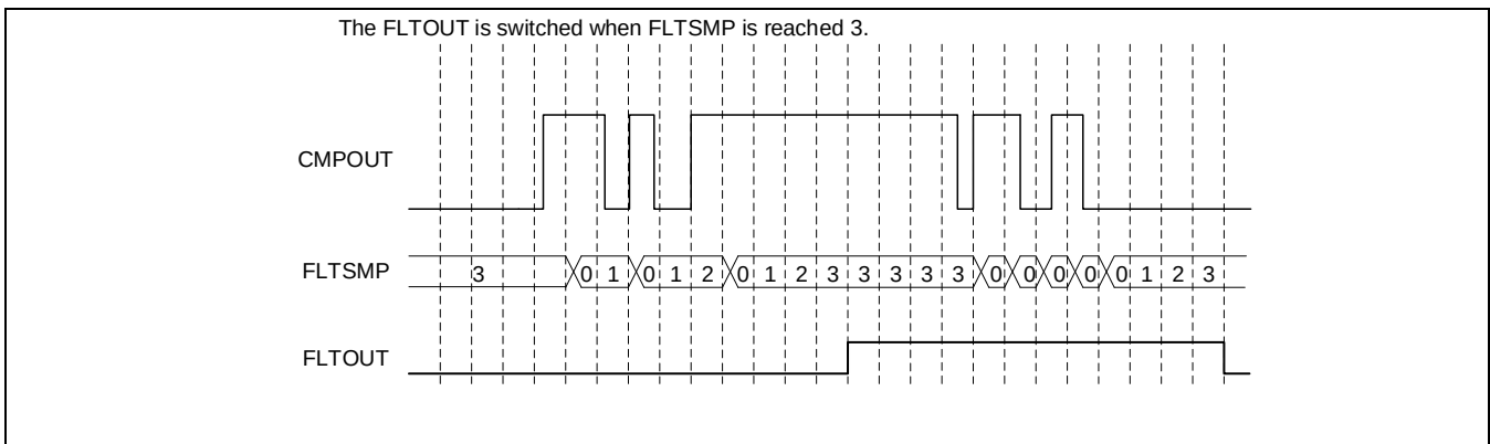
Figure 18-5 数字滤波机制
