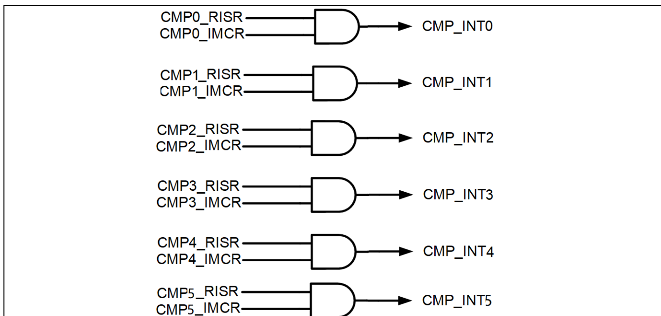
Figure 18-7 中断分配
