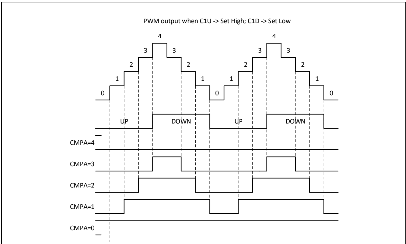
Figure 13-25 递增递减单比较值时，对称波形输出
