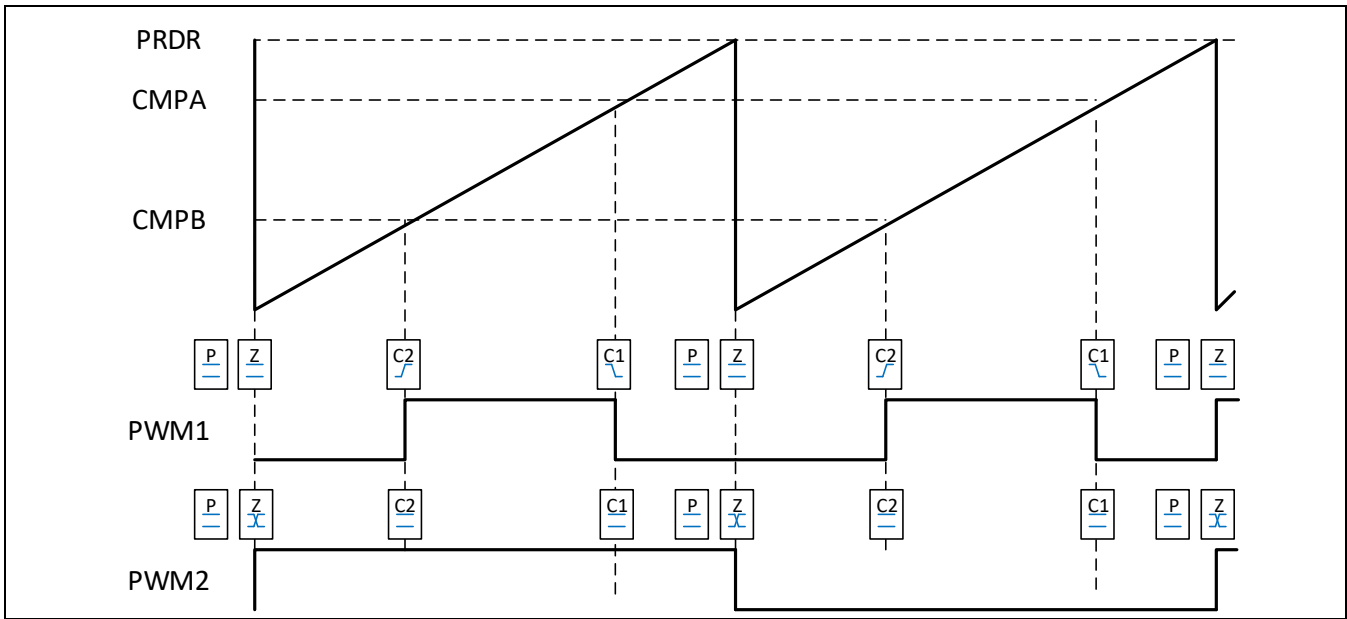
Figure 13-17 递增，脉冲定位非对称波形输出
