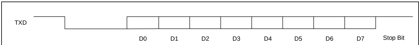
Figure 16-4 数据发送
