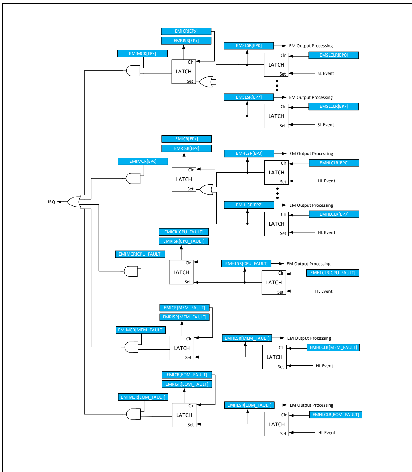
Figure 13-38 紧急模式中断
