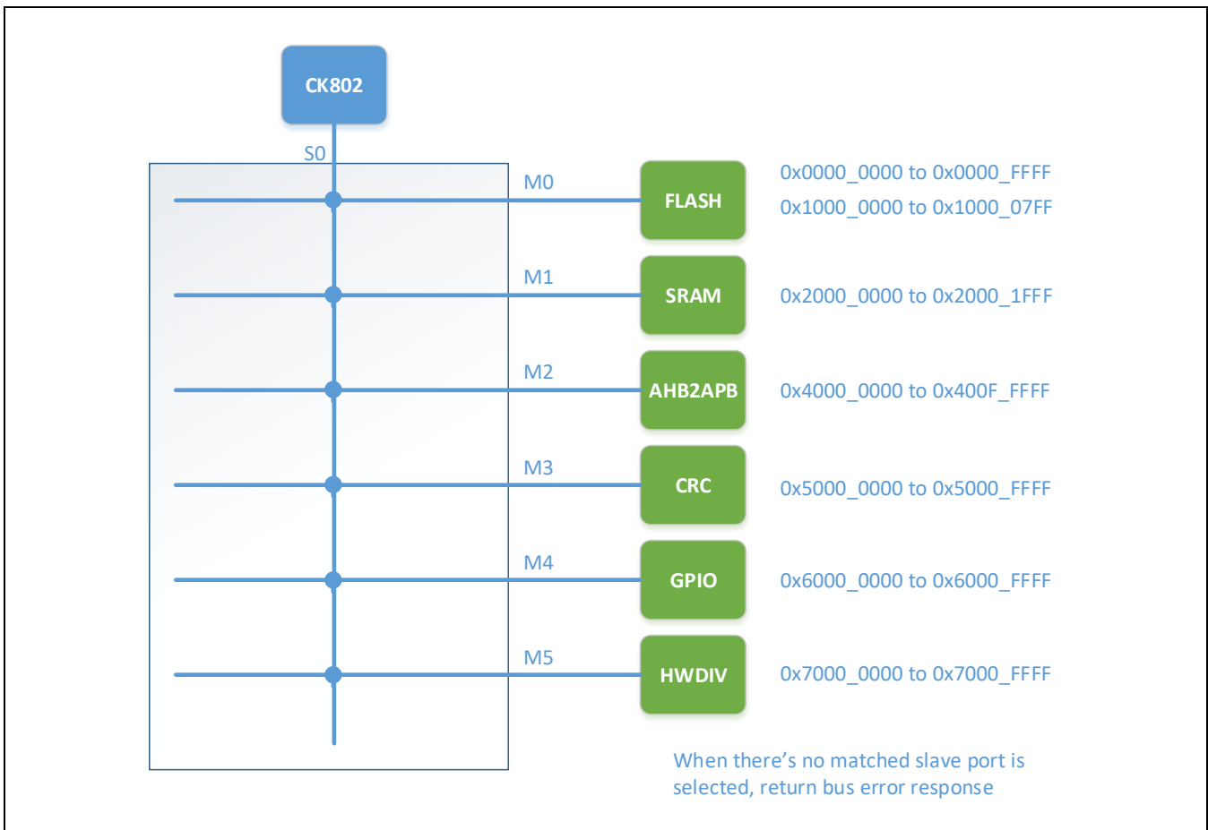
Figure 1-1 系统总线架构
