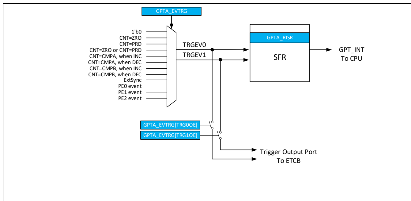
Figure 12-30 事件触发输出
