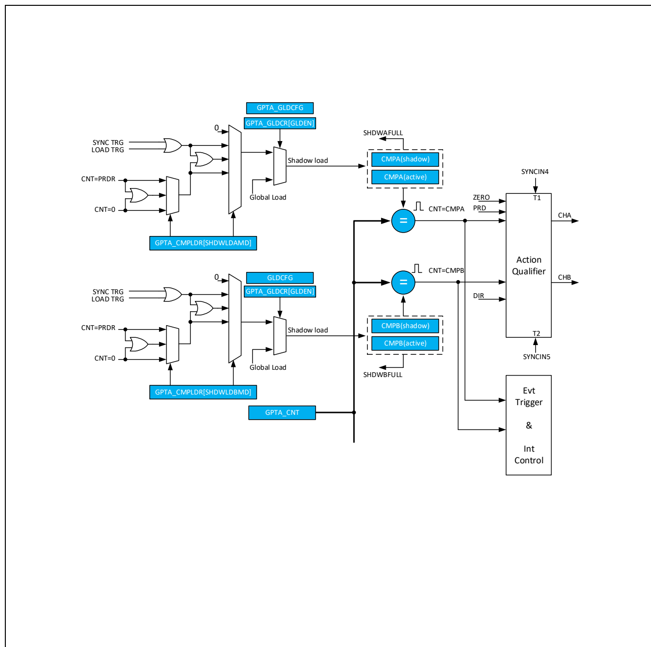
Figure 12-11 计数器值比较控制
