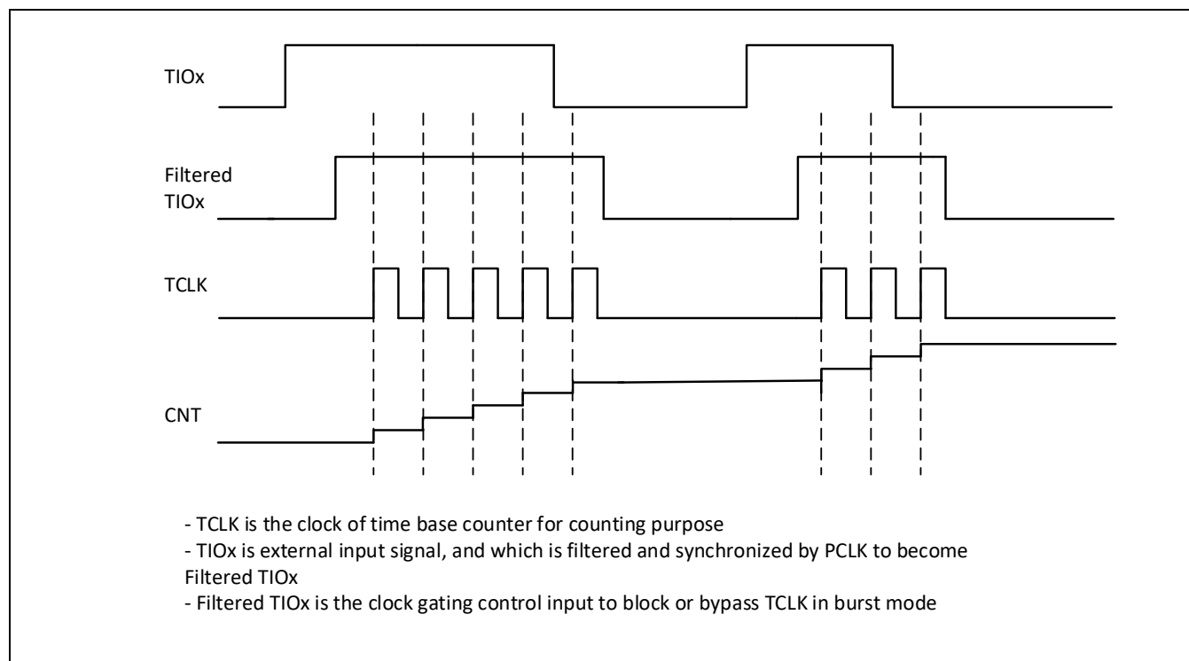
Figure 12-3 群脉冲时钟模式时序
