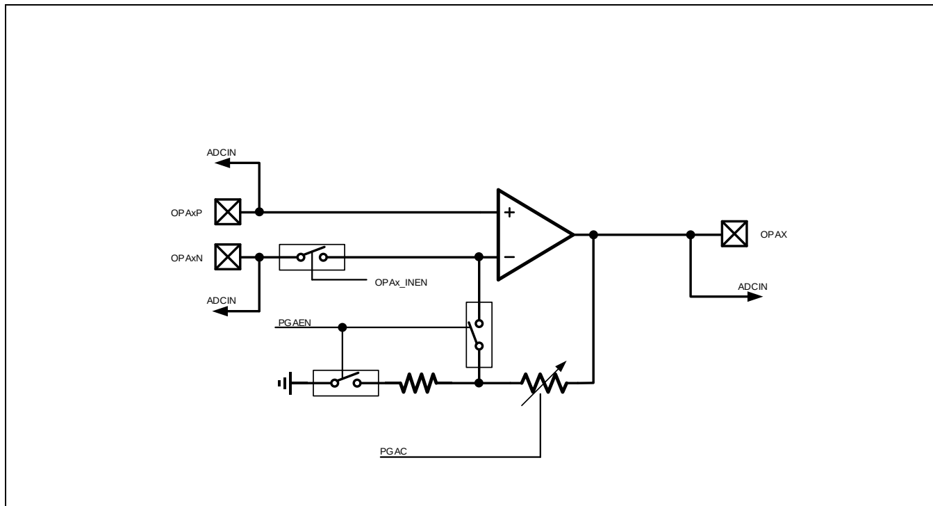
Figure 14-1 运算放大器框图
