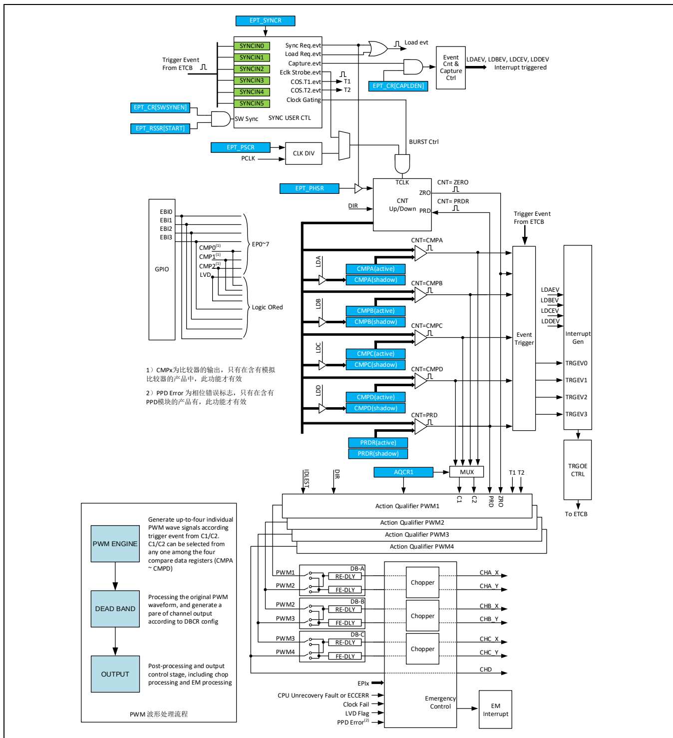
Figure 13-1 模块结构示意图
