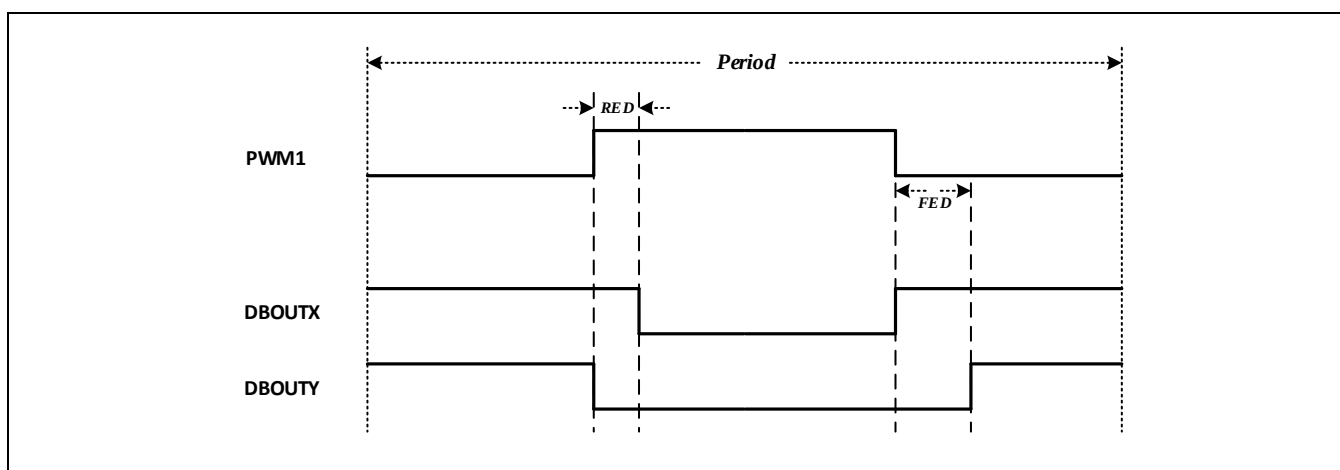
Figure 13-30 模式5: 低高电平有效死区输出举例
