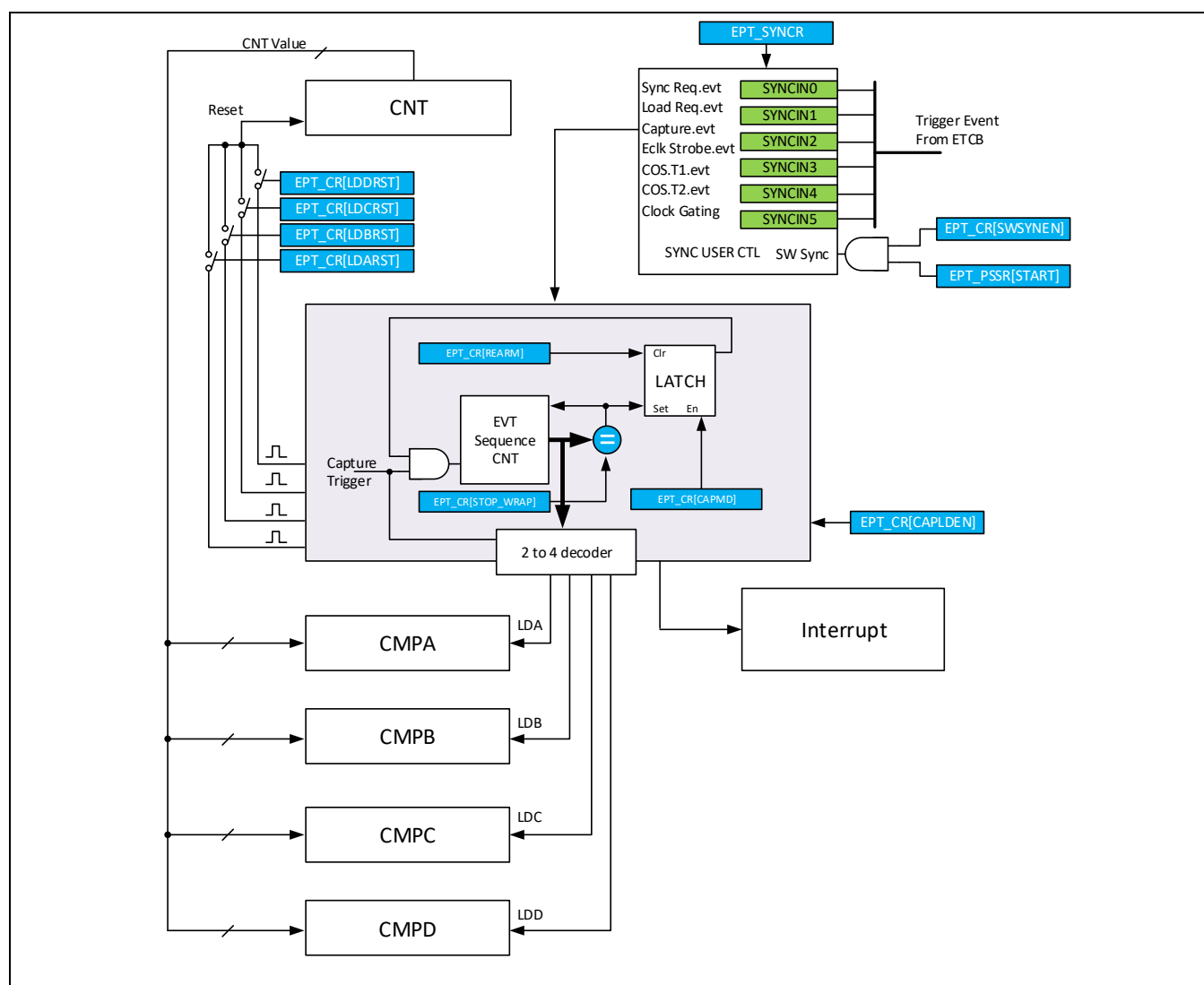
Figure 13-39 捕捉模式结构框图
