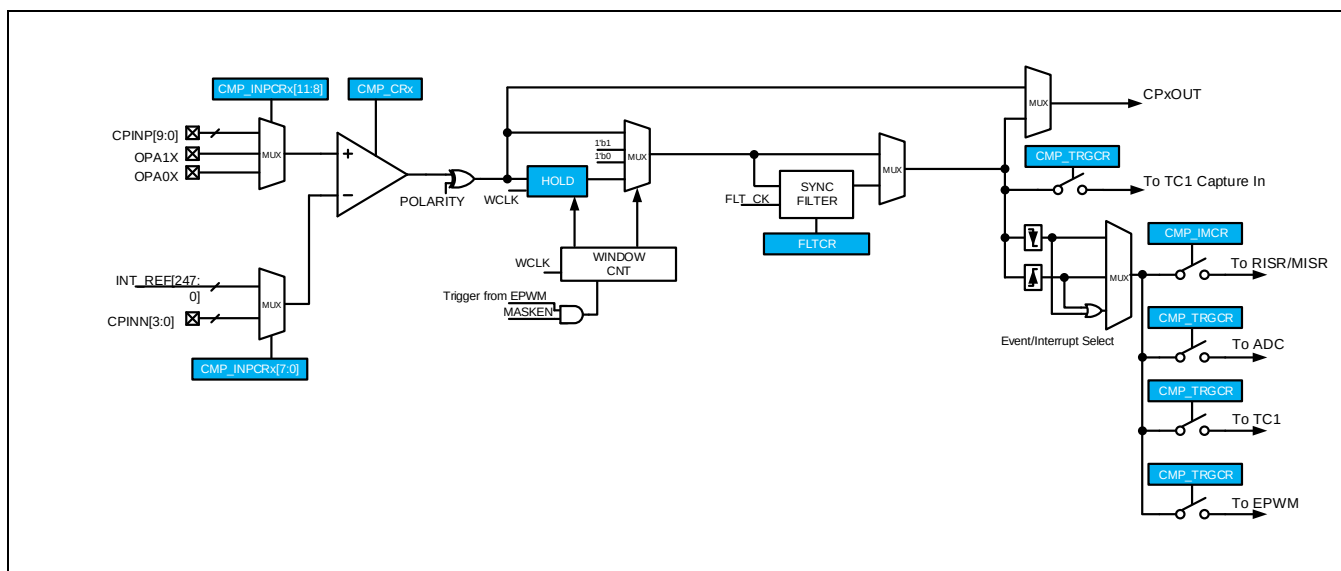
Figure 18-3 CMP2、CMP3、CMP4比较器结构示意图
