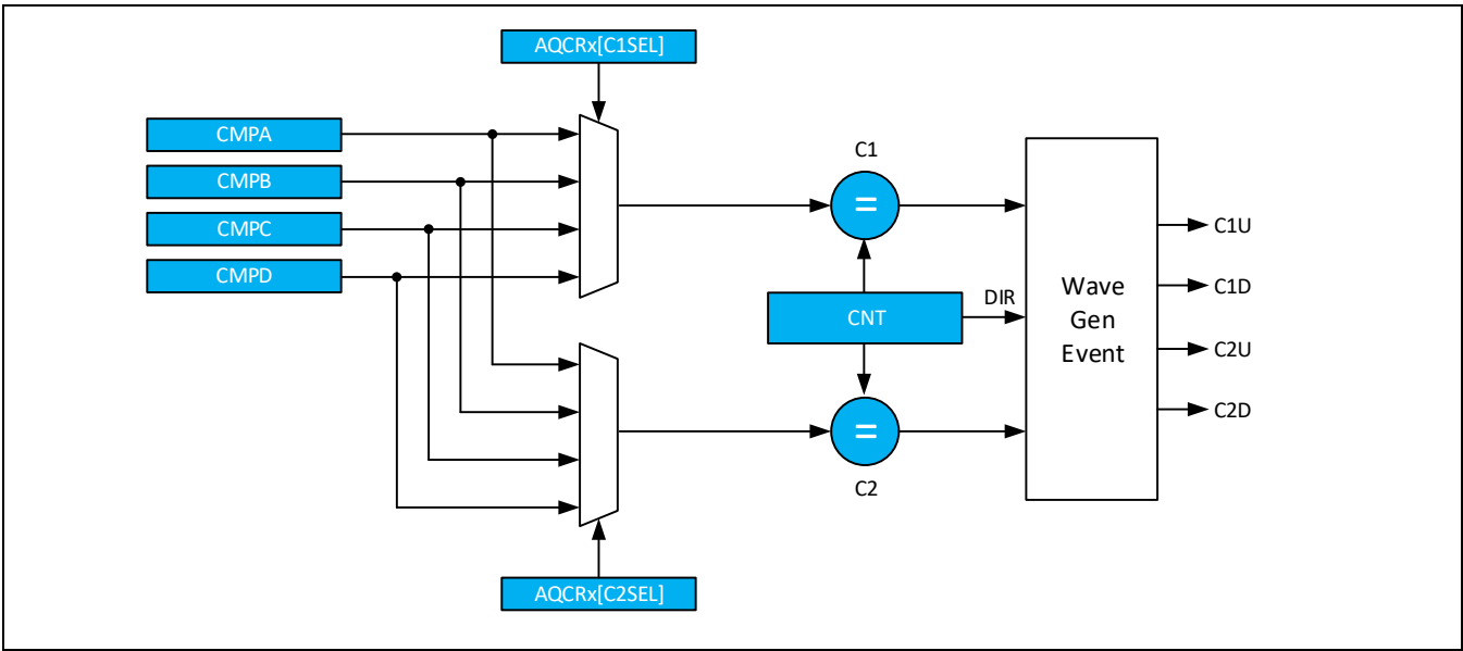
Figure 13-15 C1和C2选择控制
