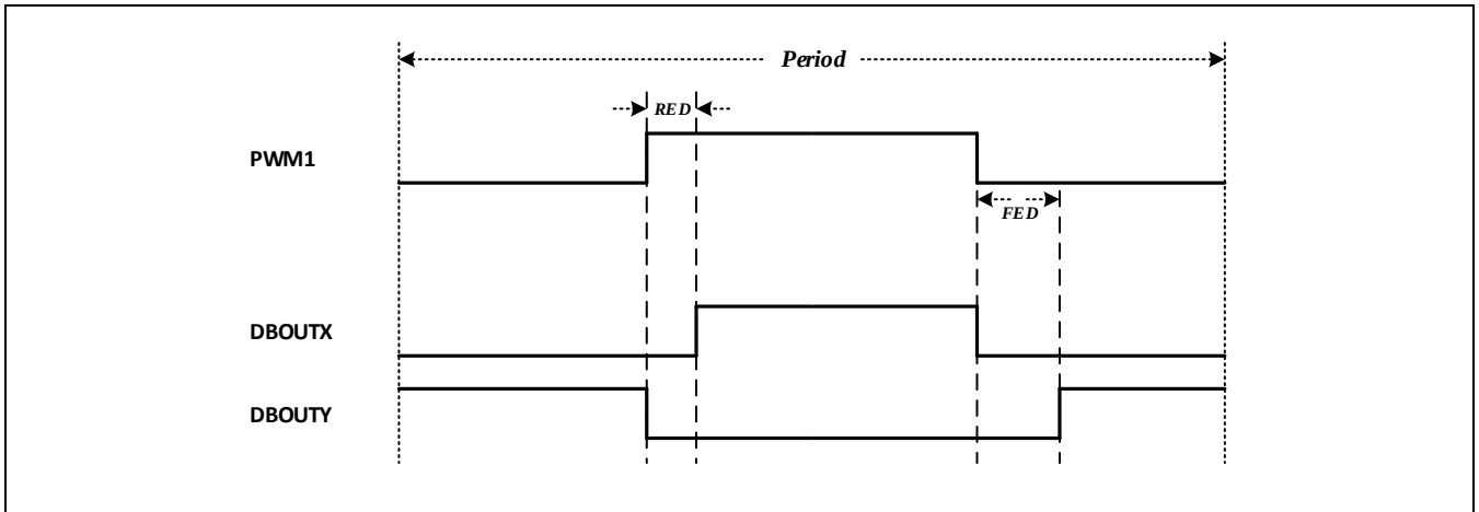
Figure 13-27 模式2：高电平有效的死区互补输出举例
