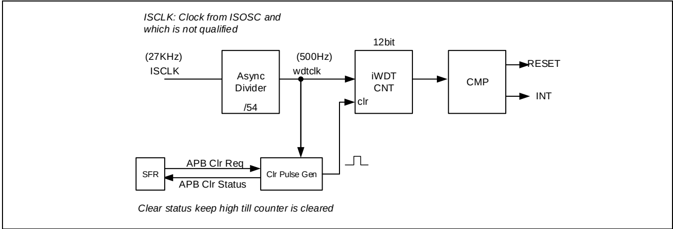
Figure 7-9 IWDT 结构框图
