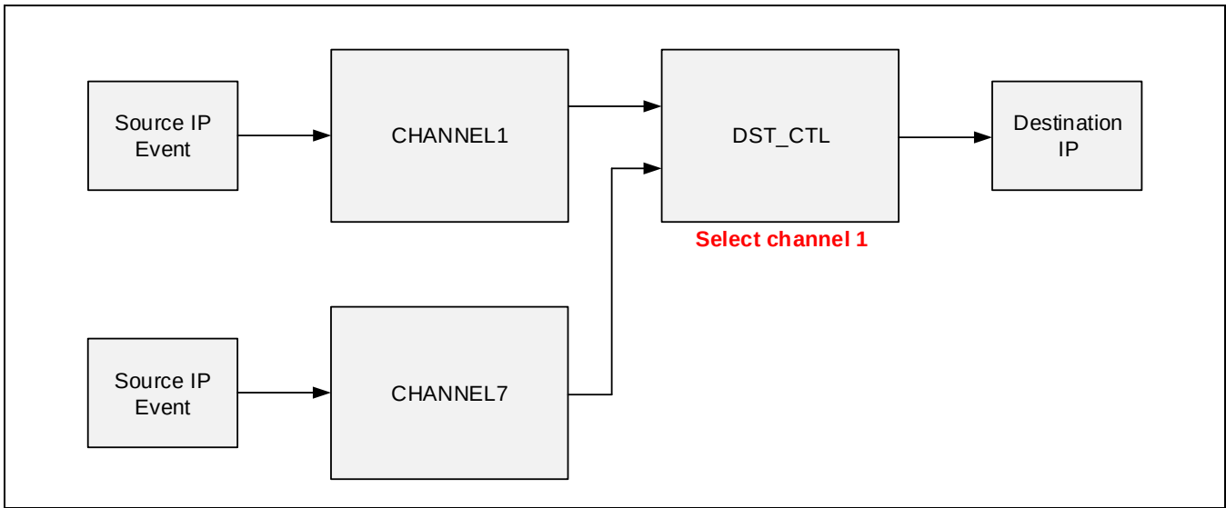
Figure 8-5 2个通道选择了相同的目标
