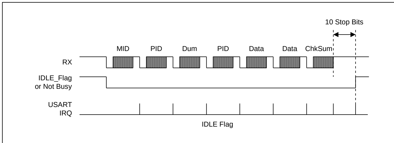
Figure 17-6 空闲标志
