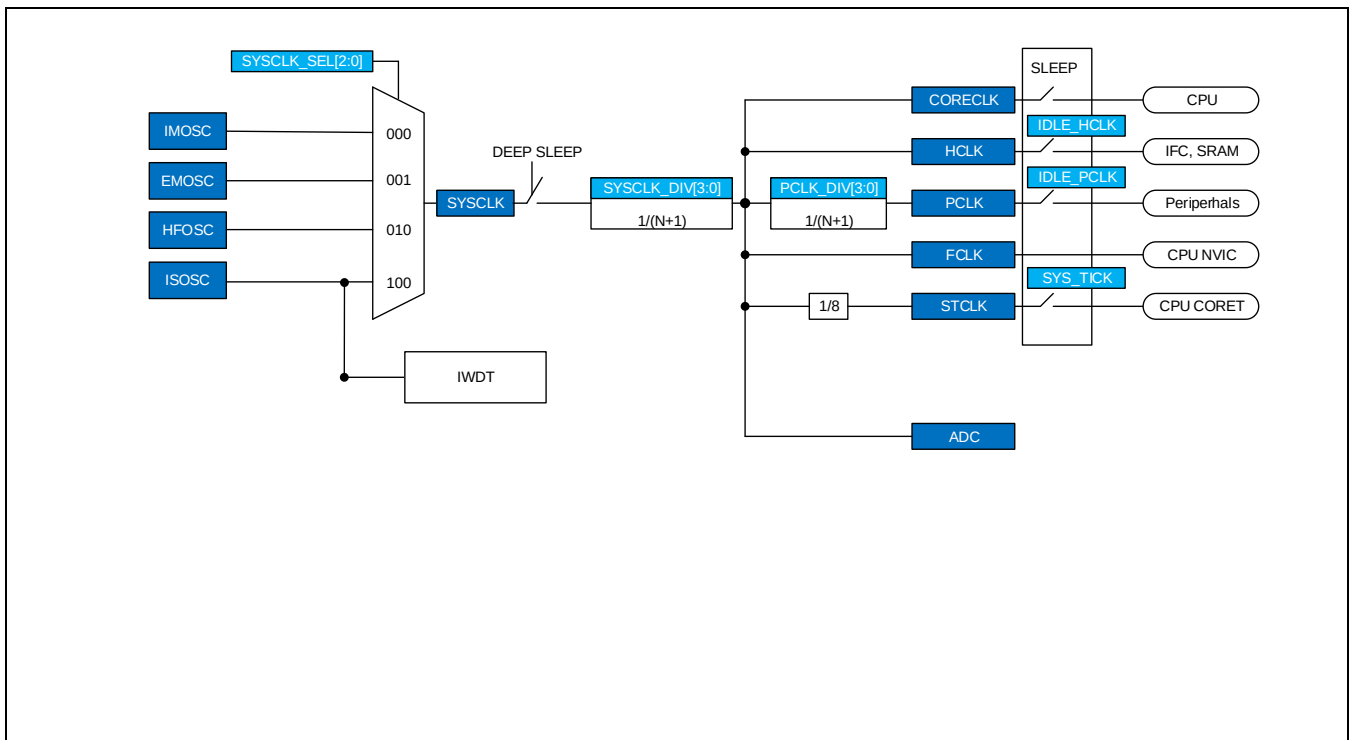
Figure 7-1 时钟结构示意图
