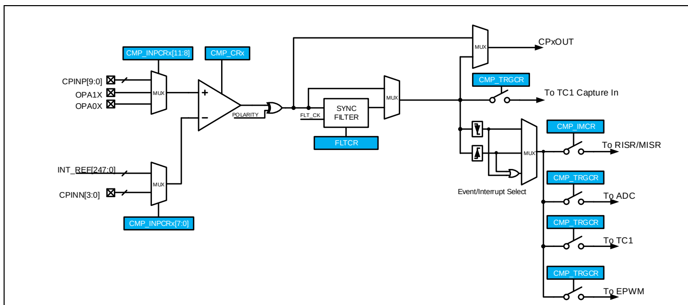
Figure 18-2 CMP0、CMP1比较器结构示意图
