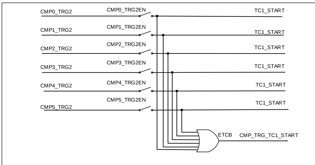
Figure 18-11 CMP 触发 TC1 的启动触发及产生相关 ETCB 触发信号
