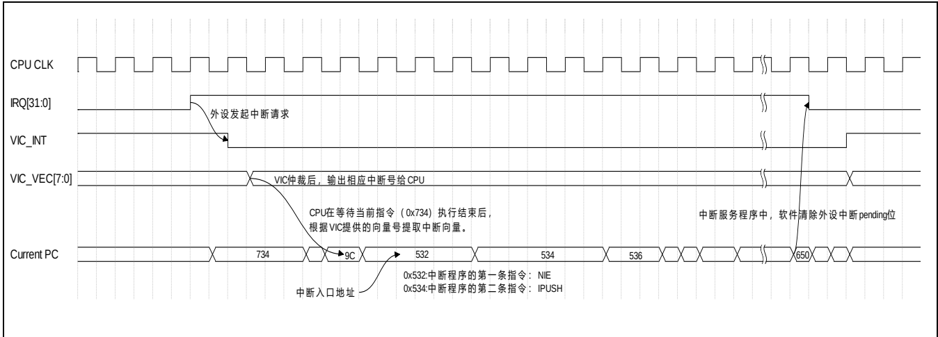
Figure 2-2 中断响应过程
