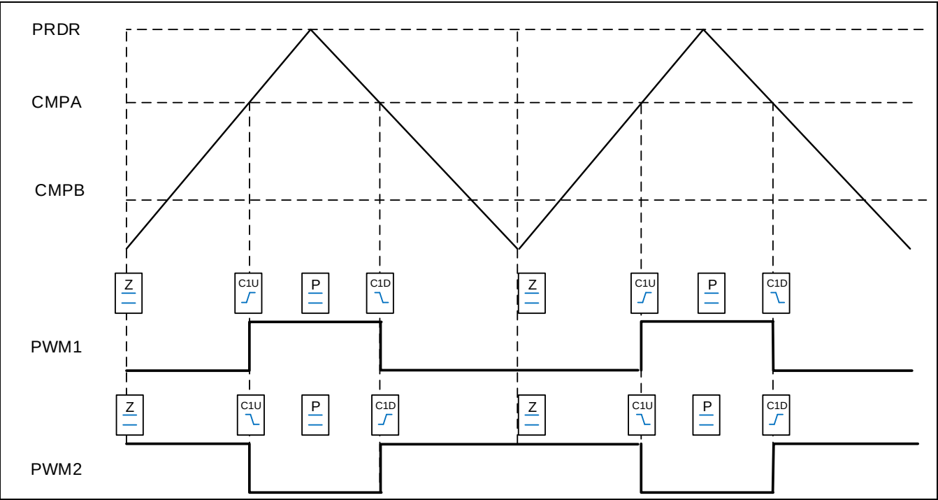
Figure 12-22 递增递减，双沿对称波形输出
