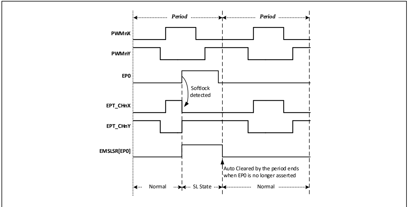
Figure 13-36 软锁止模式
