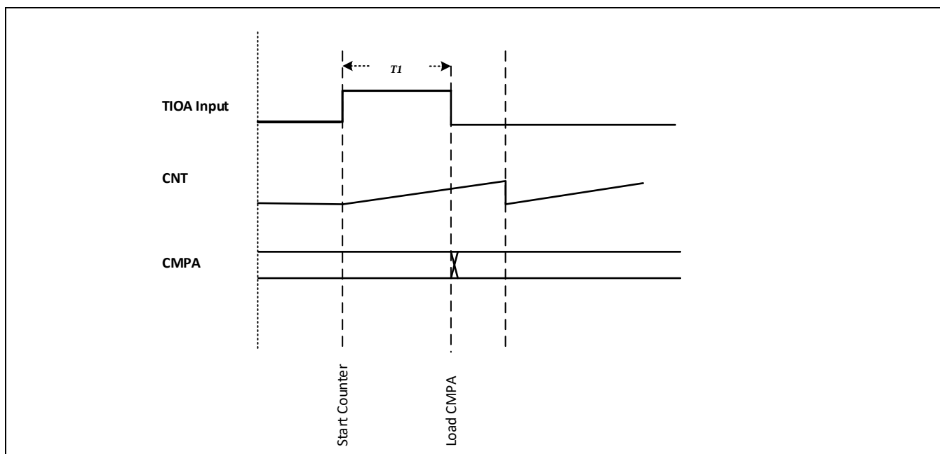
Figure 13-41 测量TIOA的脉冲宽度
