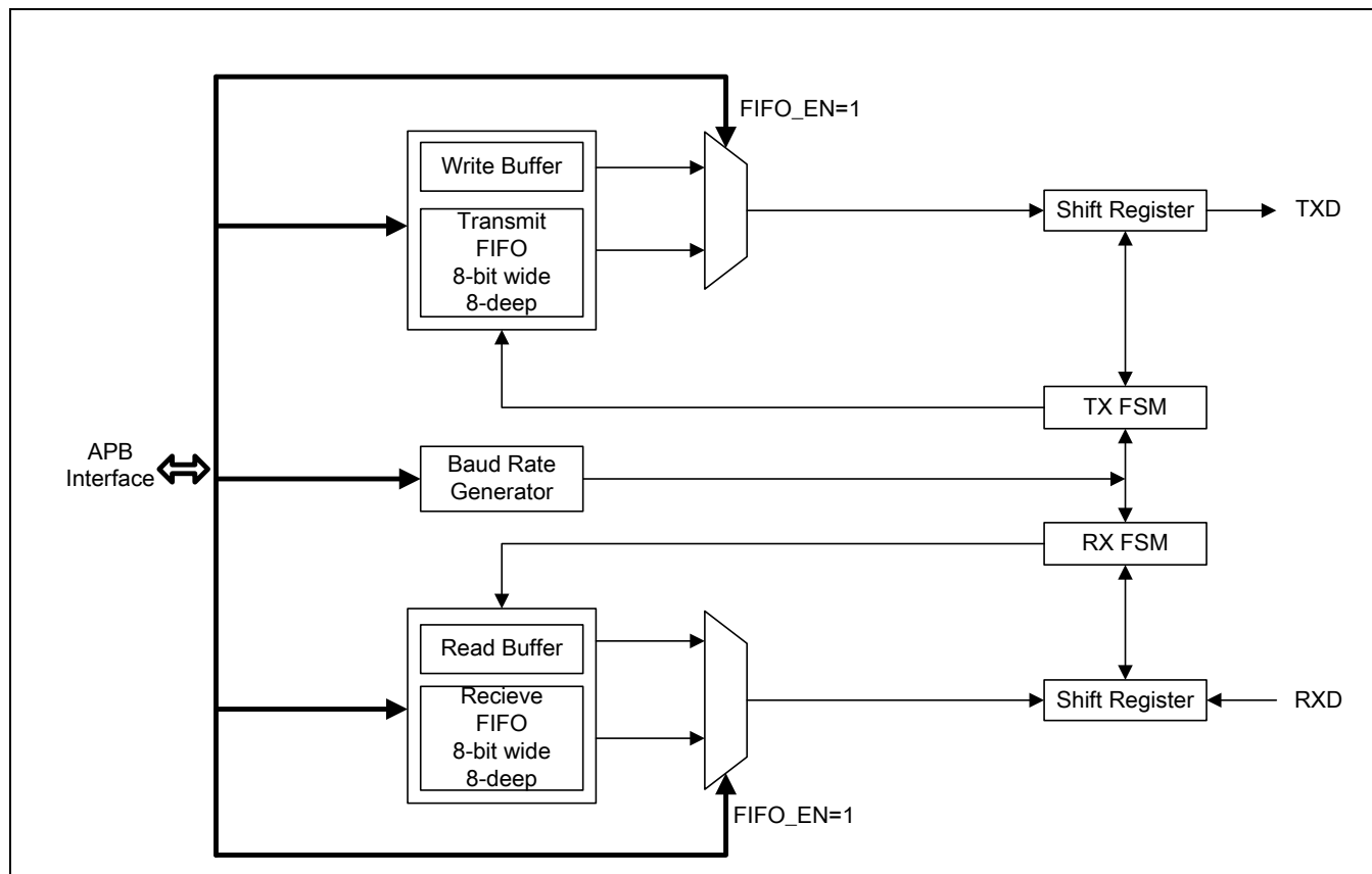
Figure 16-1 UART模块框图
