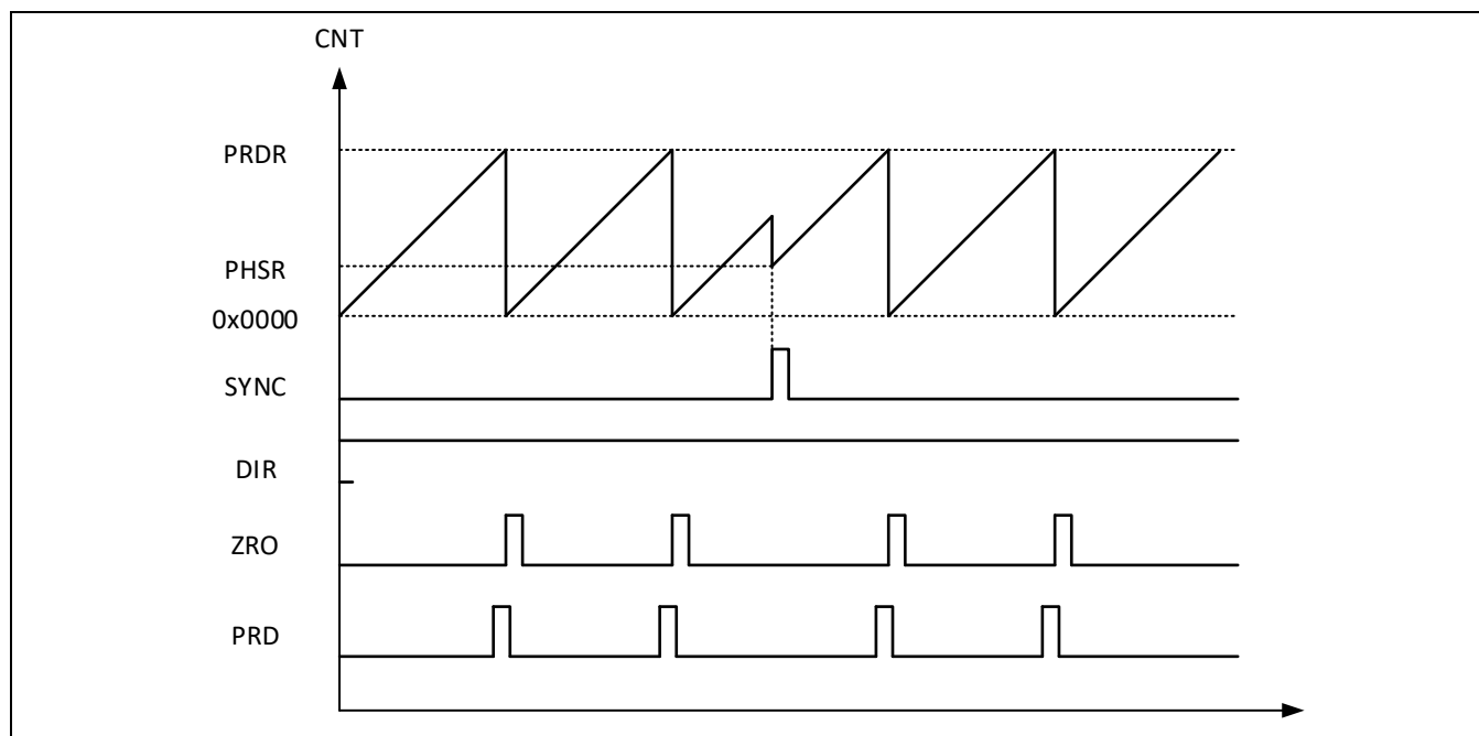
Figure 12-7 递增工作模式
