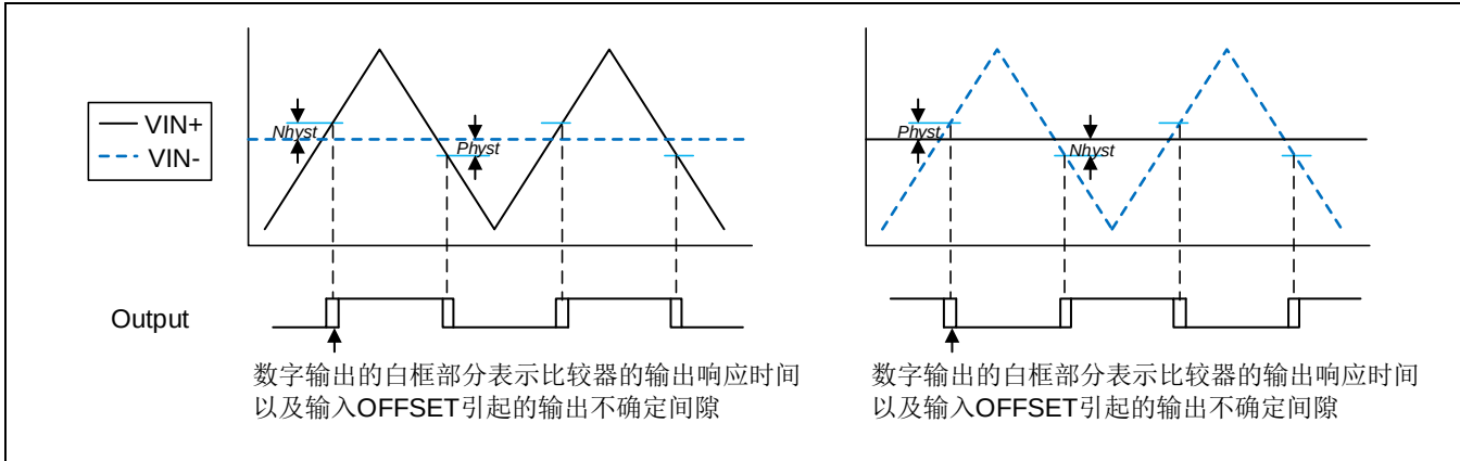
Figure 18-1 单一比较器示意图
