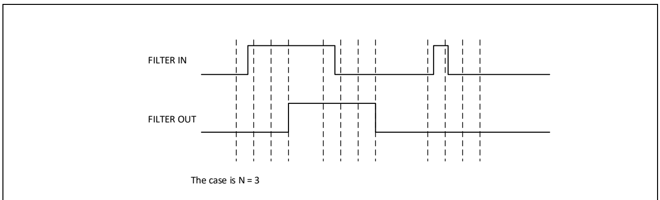
Figure 12-4 CG Filter 数字滤波器的原理
