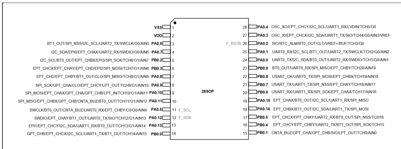
Figure 2-3 管脚定义图(28SOP)
