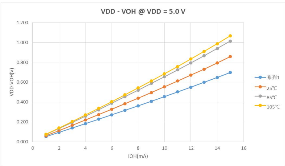
Figure 3-1 ( V_{DD}-V_{OH} ) 温度曲线
