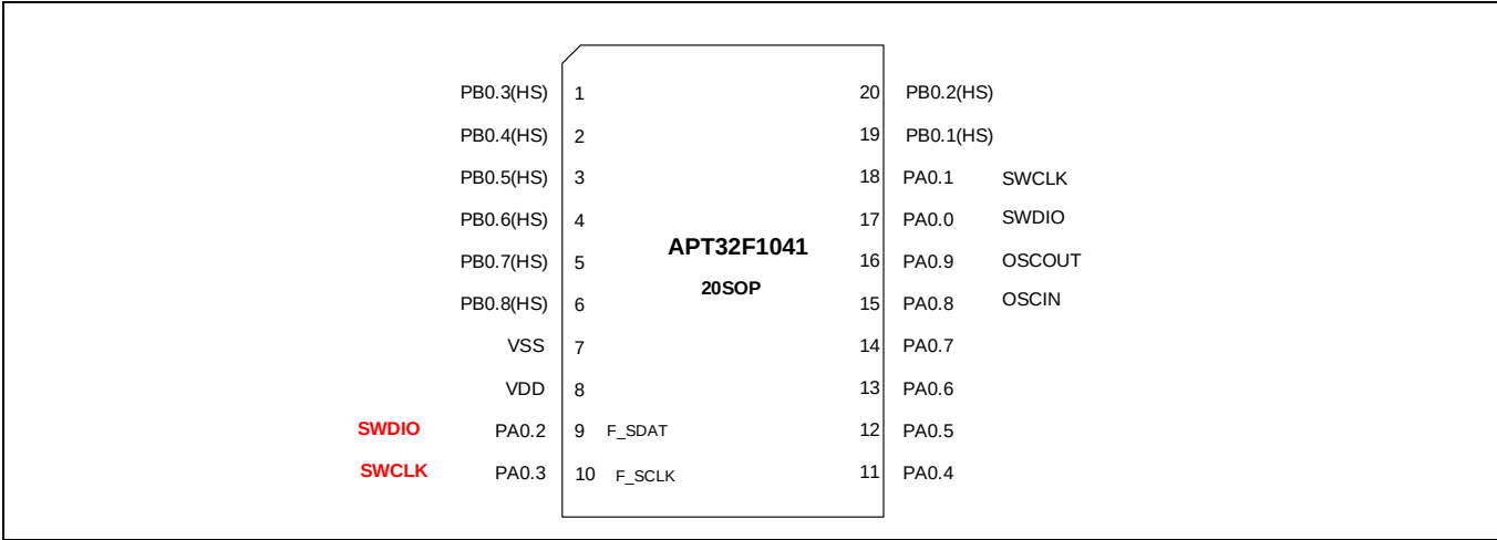
Figure 2-2 管脚定义图(SOP20)
