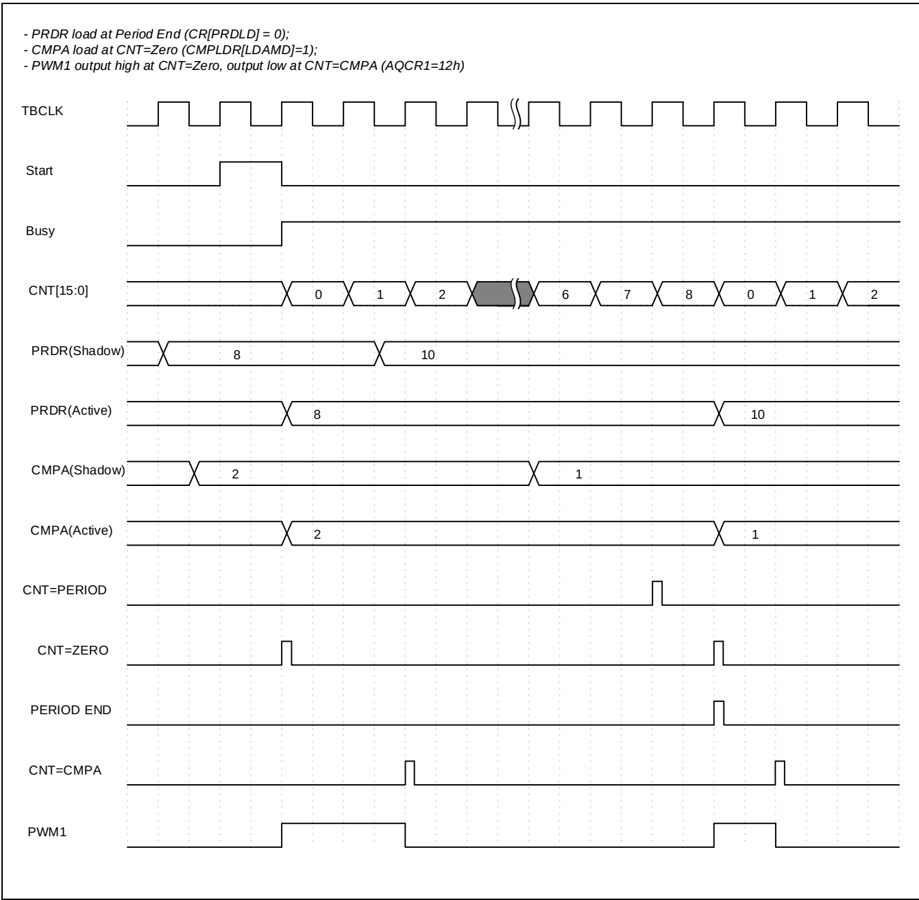
Figure 11-16 递增单比较值时，非对称波形输出
