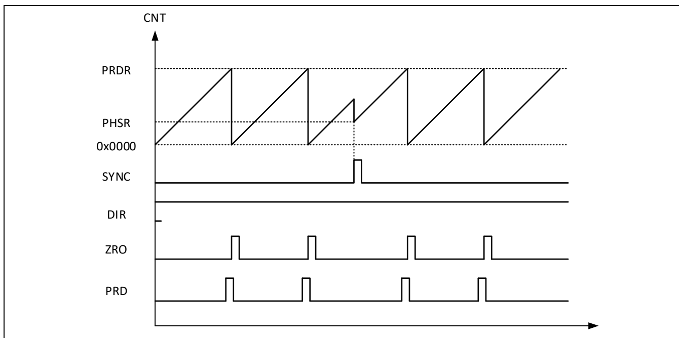
Figure 10-7 递增工作模式
