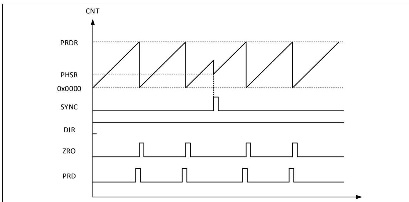
Figure 11-7 递增工作模式
