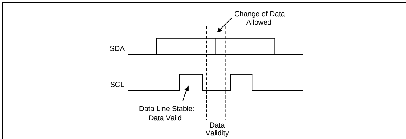
Figure 13-2 数据有效性
