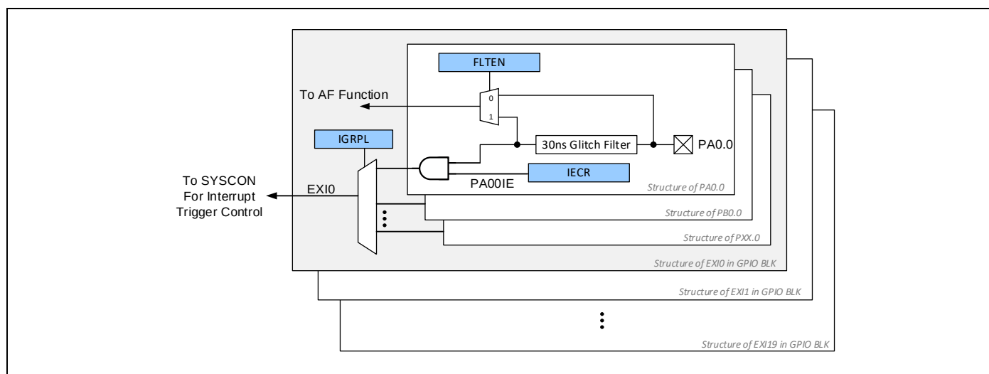
Figure 6-2 GPIO外部中断原理图
