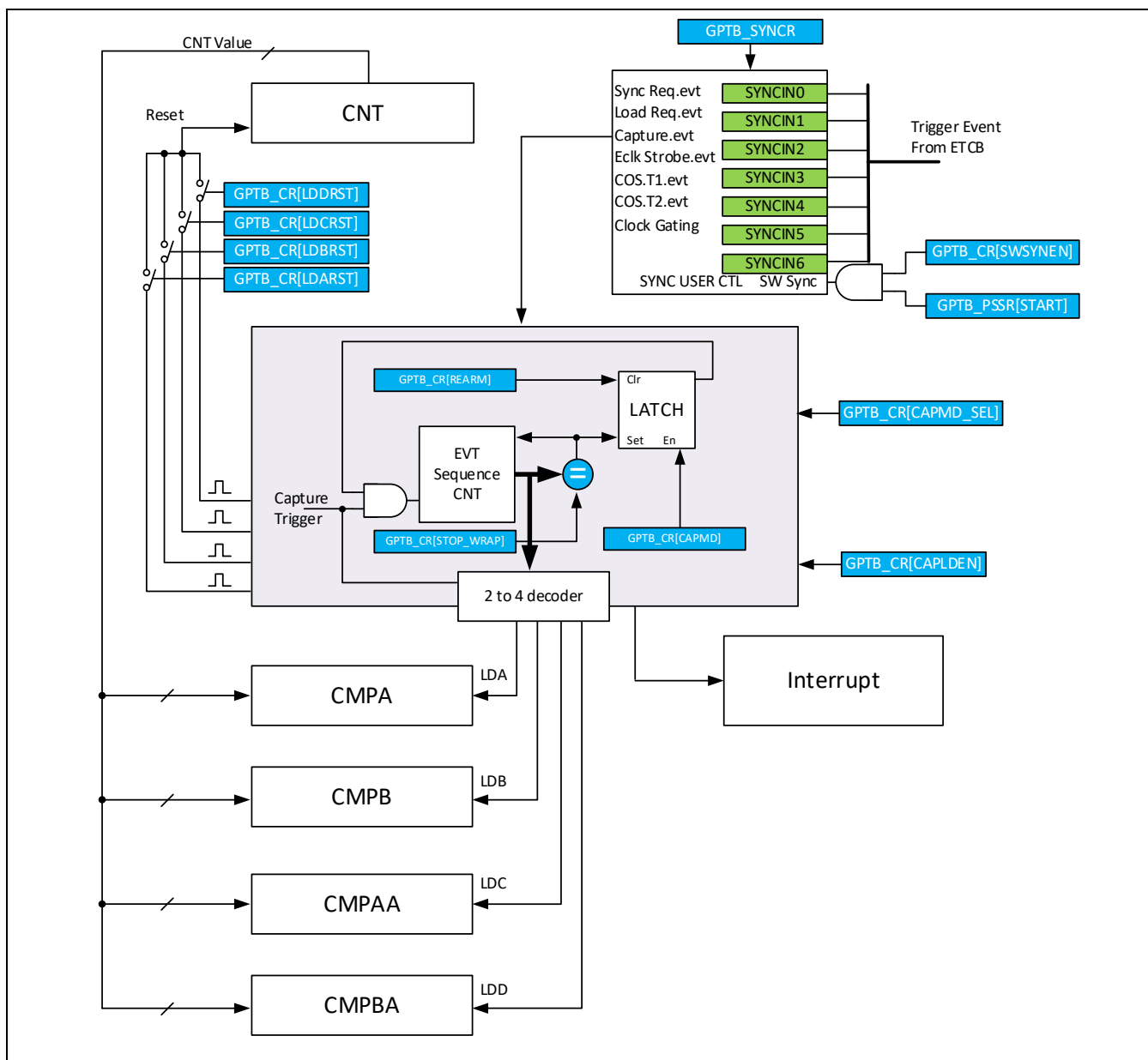
Figure 11-26 捕获模式结构框图
