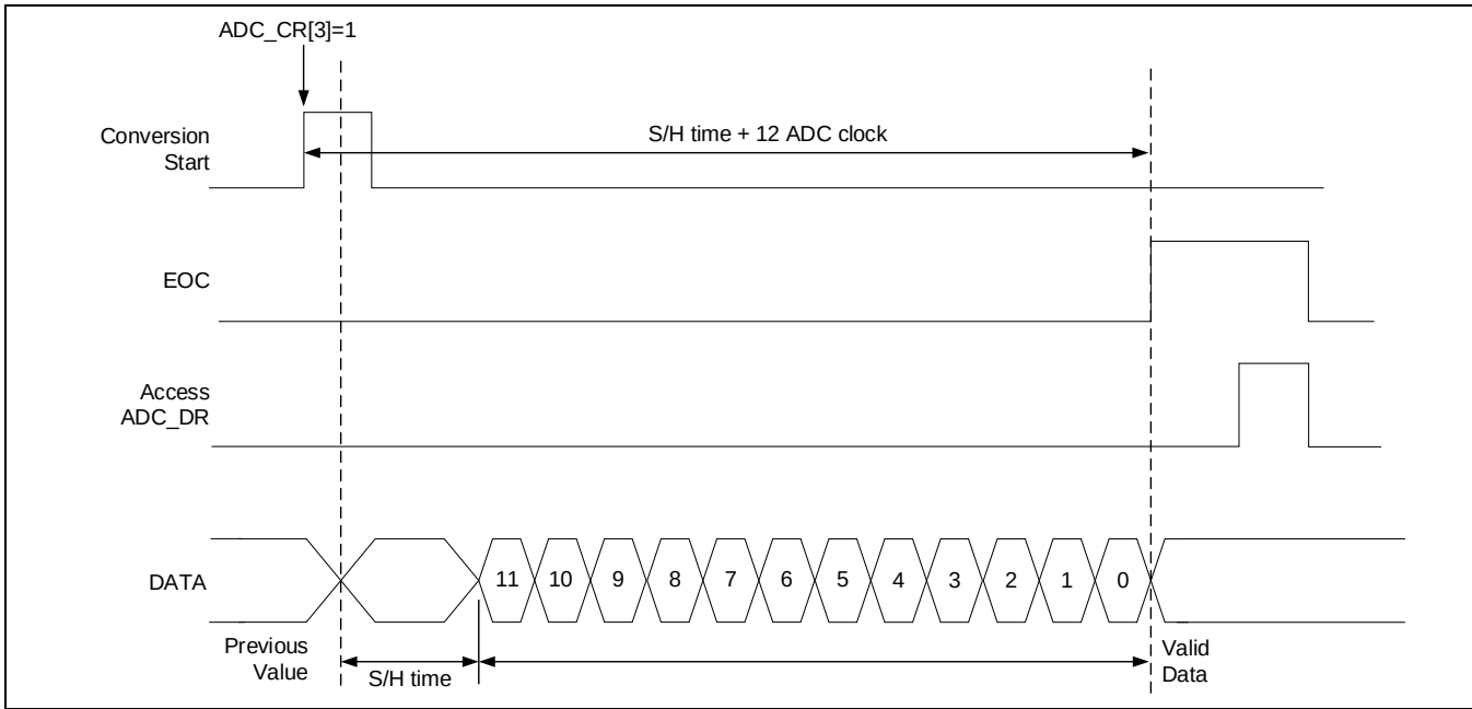
Figure 16-4 ADC工作时序图
