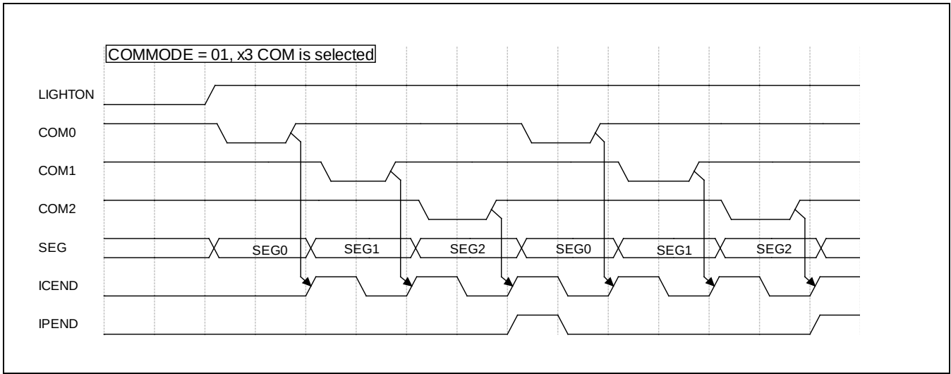
Figure 17-16 中断产生示意图
