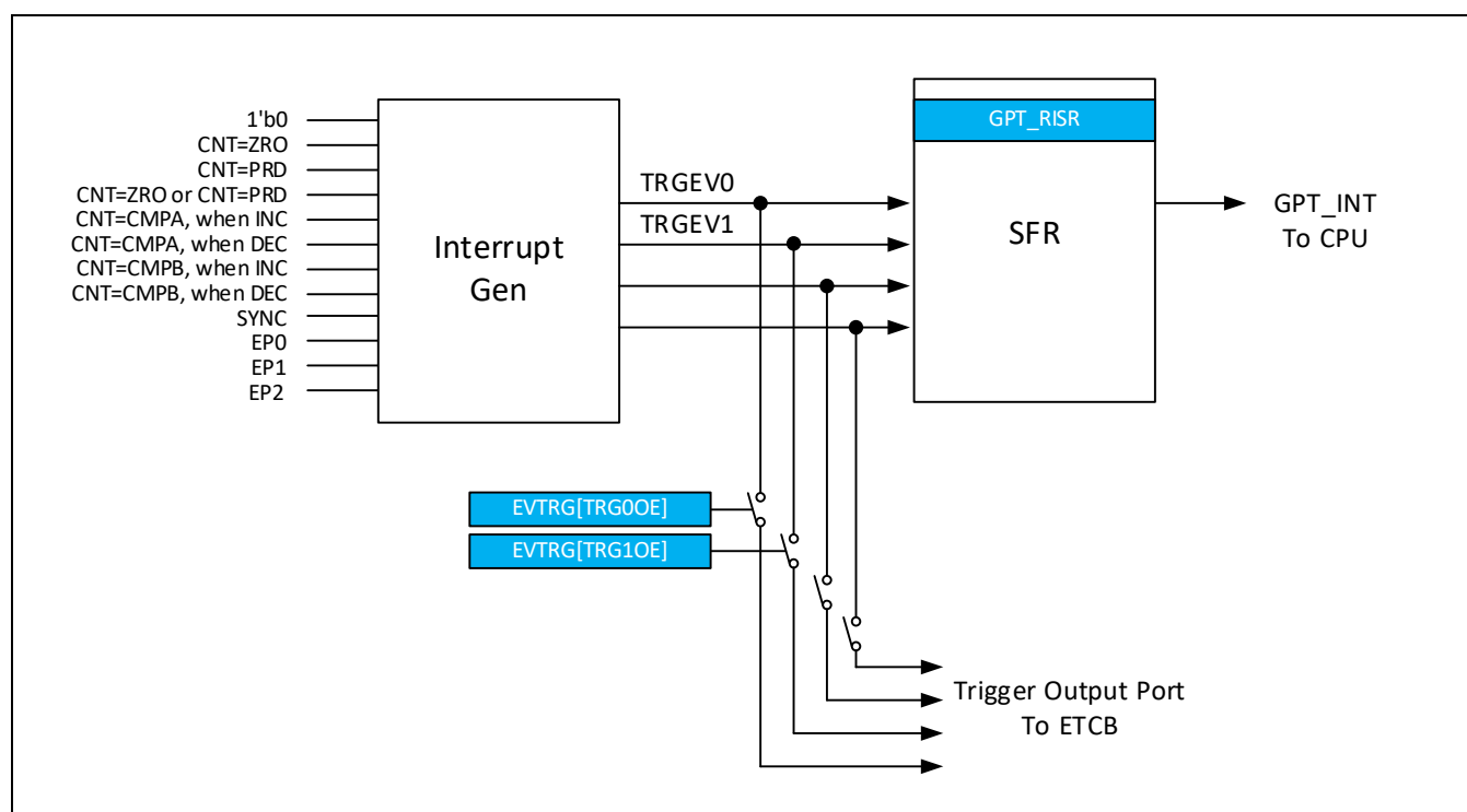
Figure 11-33 同步触发输出
