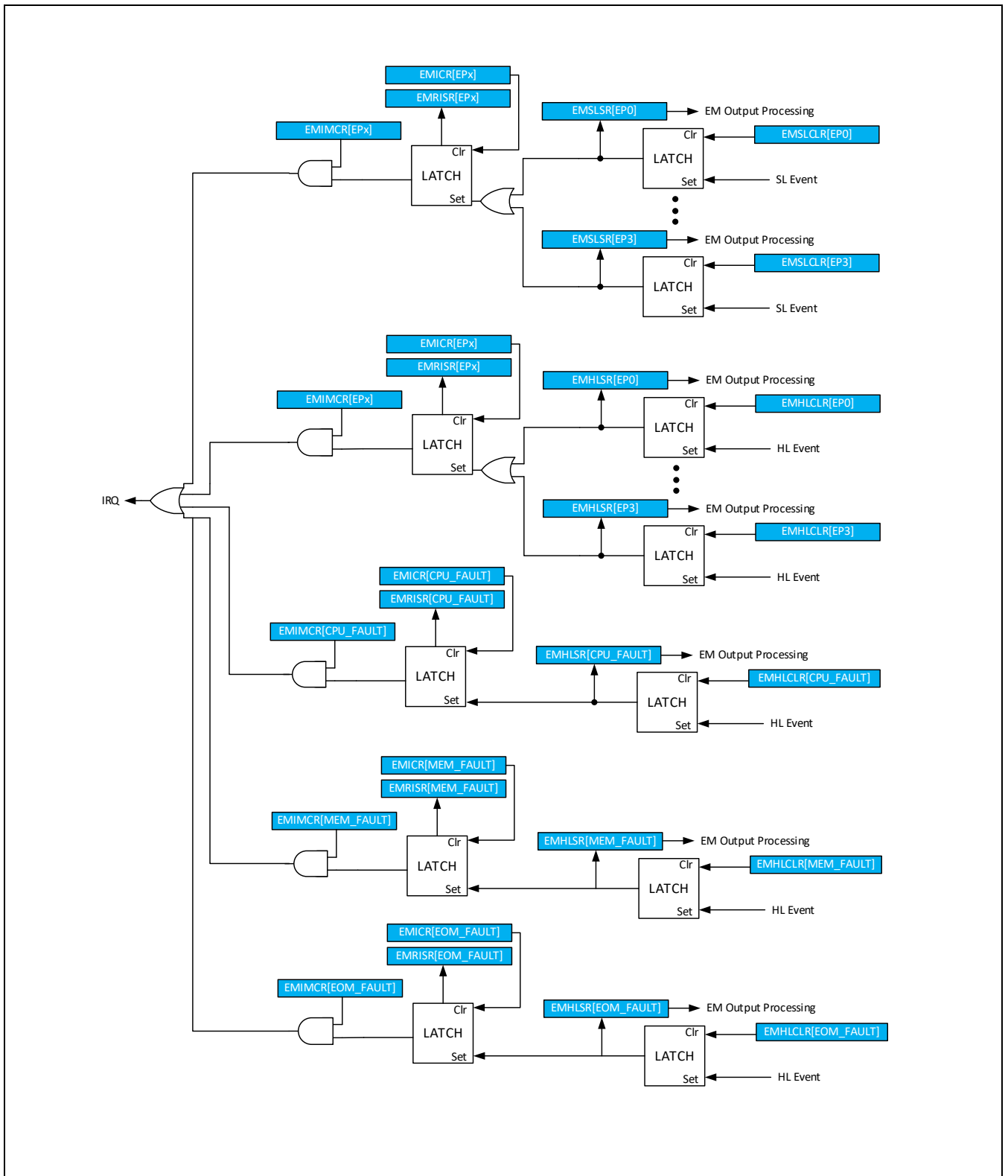
Figure 11-25 紧急模式中断
