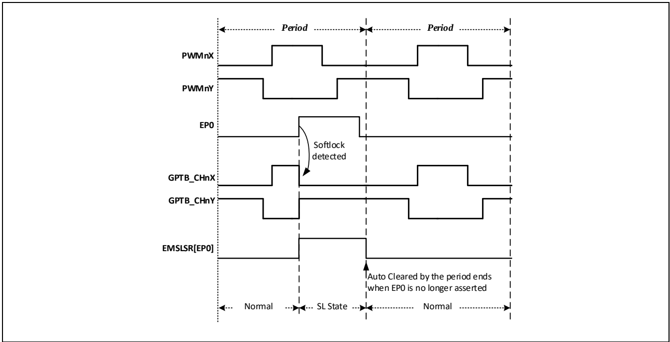
Figure 11-23 软锁止模式
