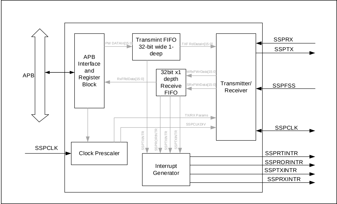
Figure 14-1 SPI 模块框图
