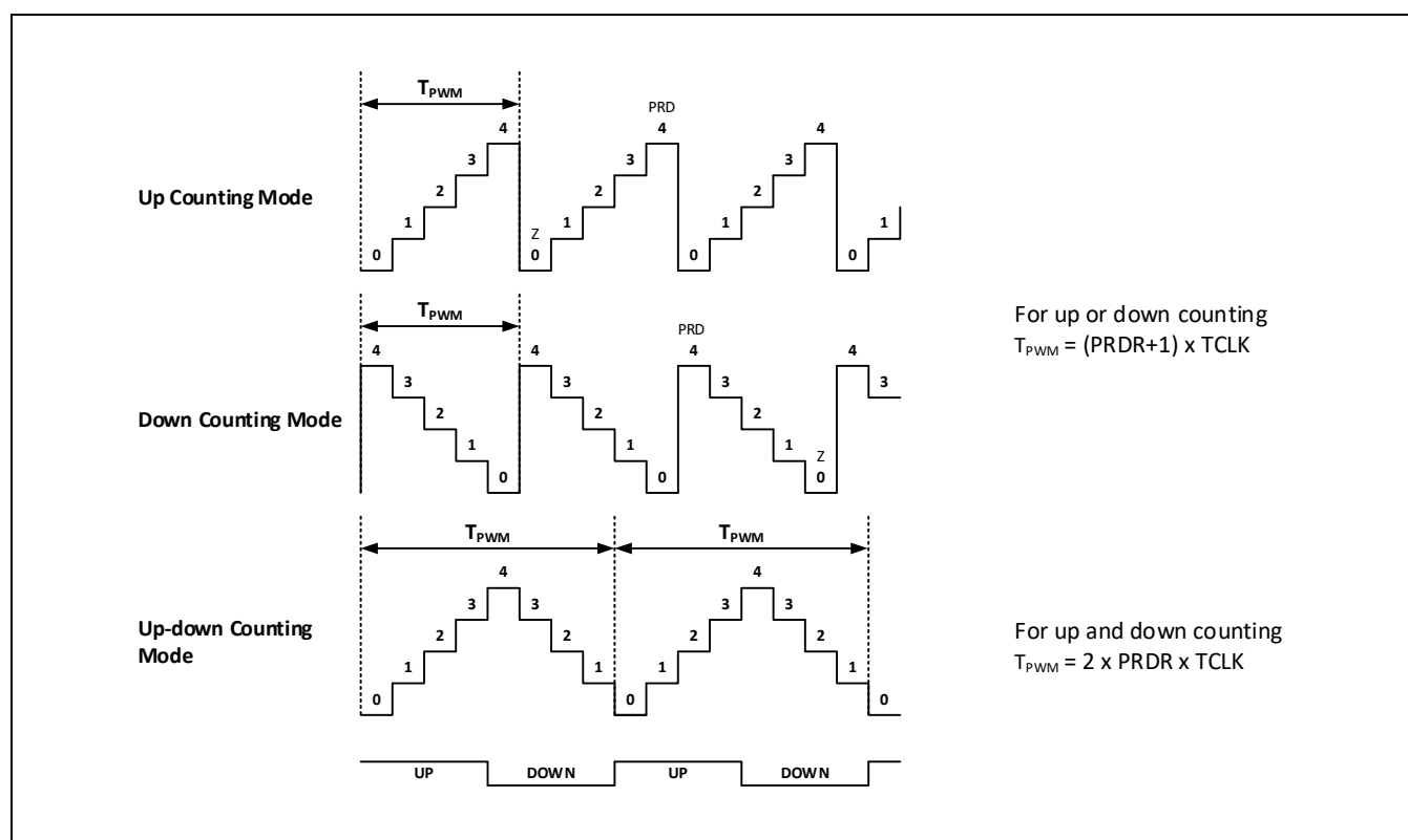
Figure 11-6 计数器工作模式
