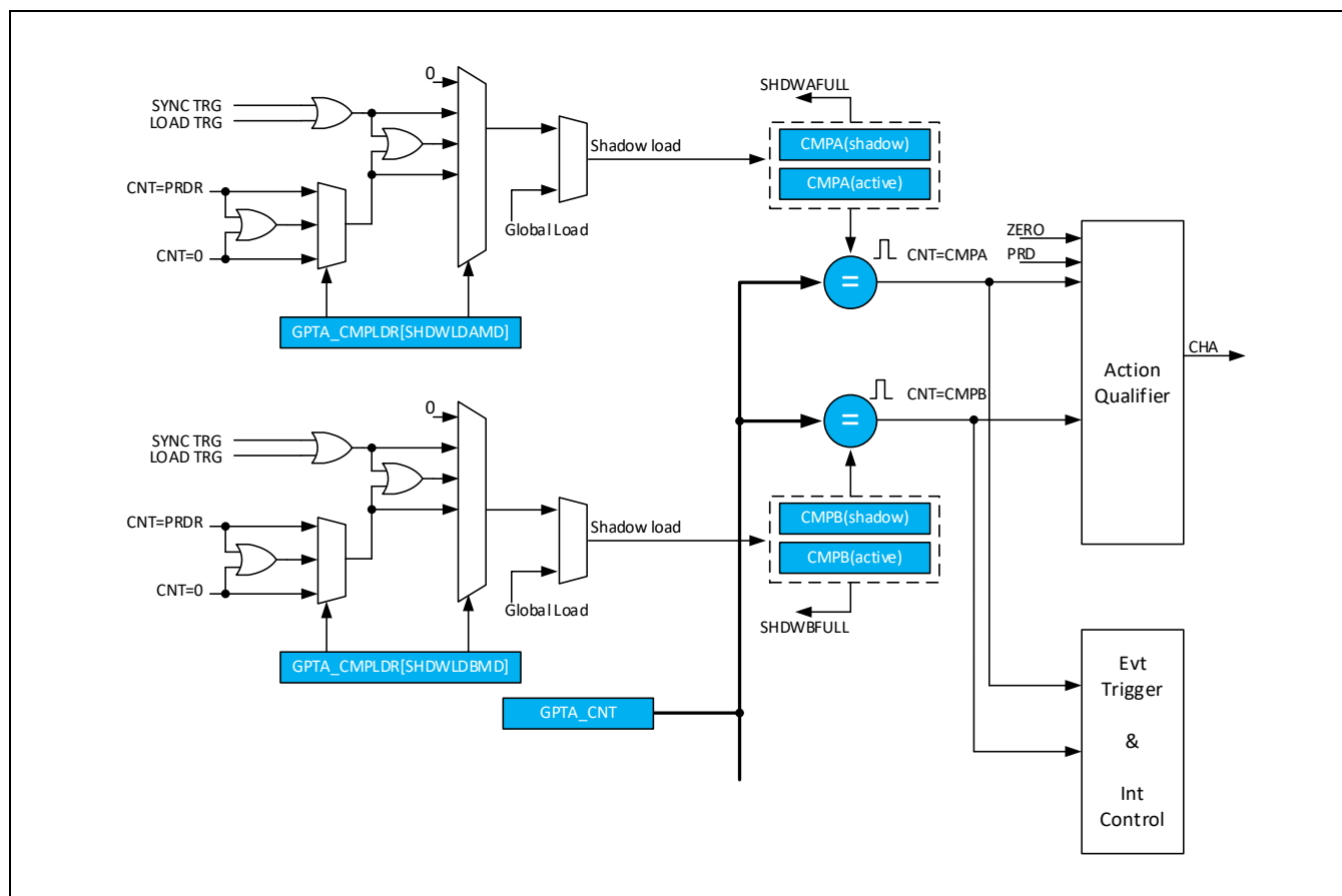
Figure 10-8 计数器值比较控制
