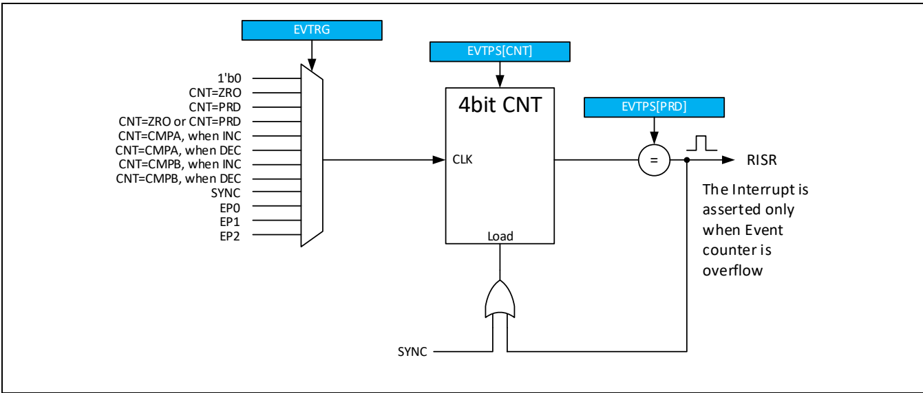
Figure 11-34 事件计数器
