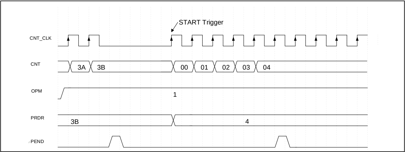
Figure 8-3 BT One Pulse 计数模式
