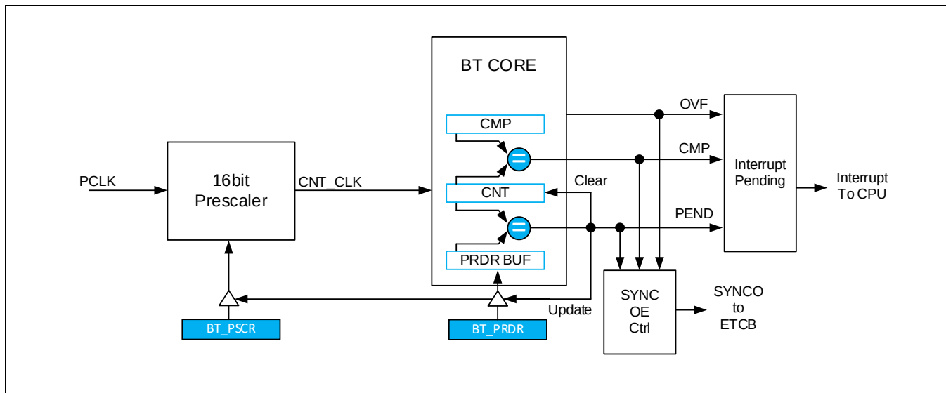
Figure 8-1 模块结构示意图
