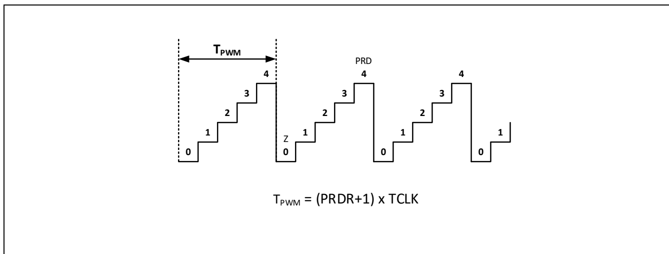
Figure 10-6 计数器工作模式
