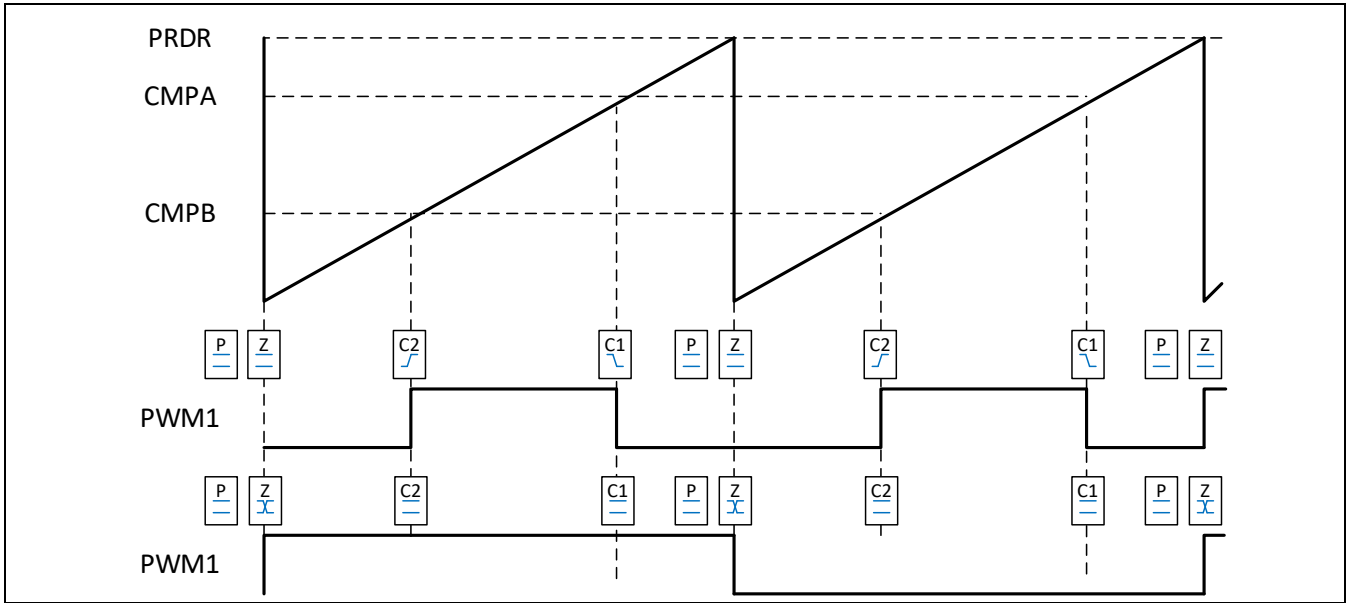
Figure 10-20 递增，脉冲定位非对称波形输出
