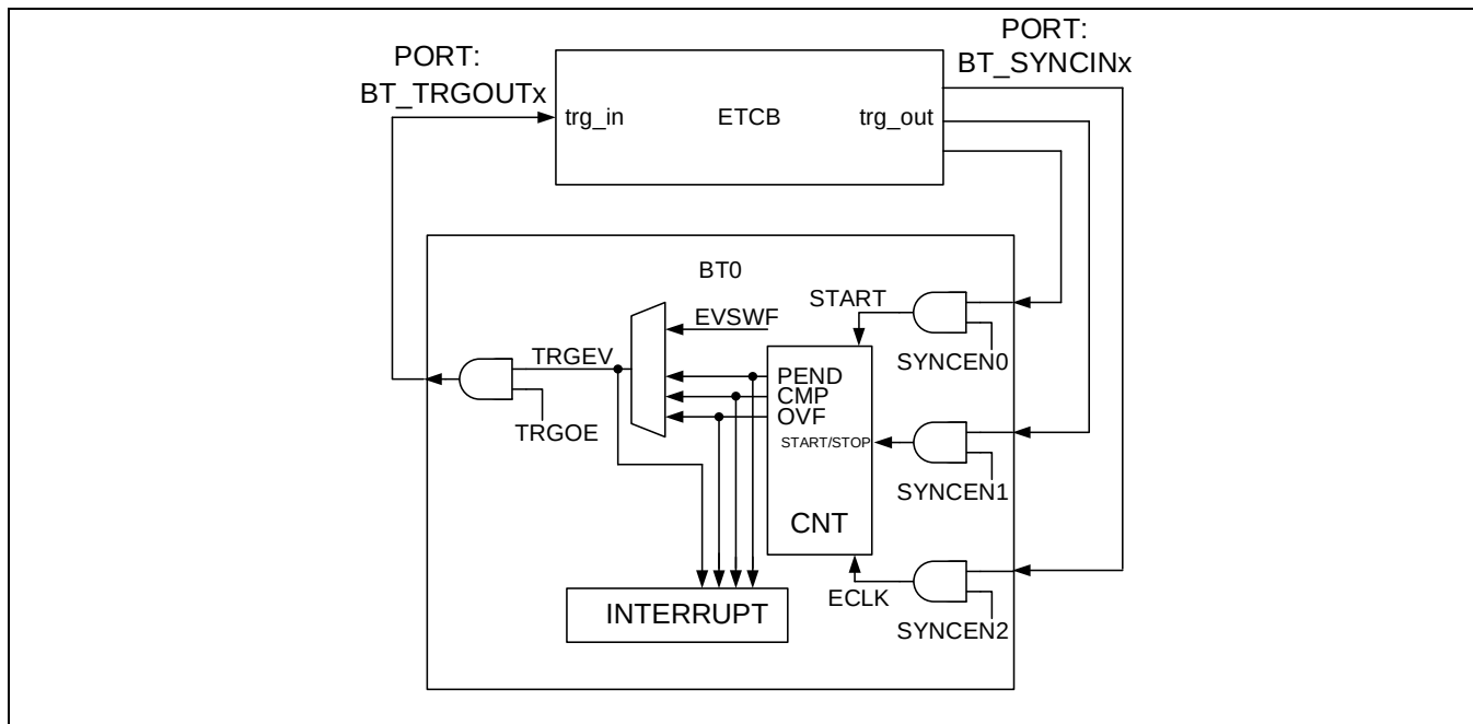
Figure 8-4 同步触发原理
