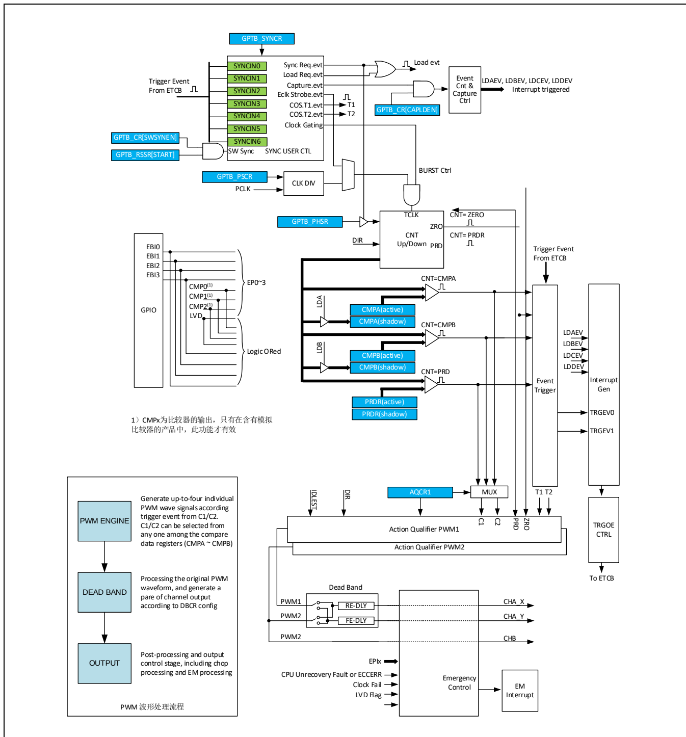
Figure 11-1 模块结构示意图
