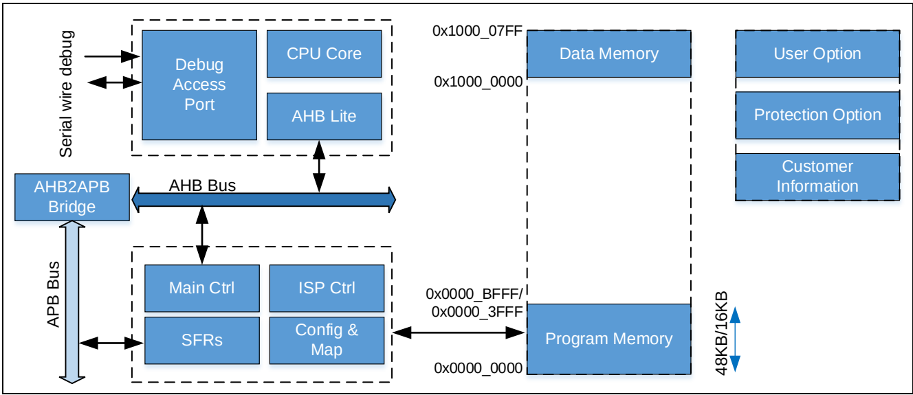
Figure 4-1 IFC模块框图
