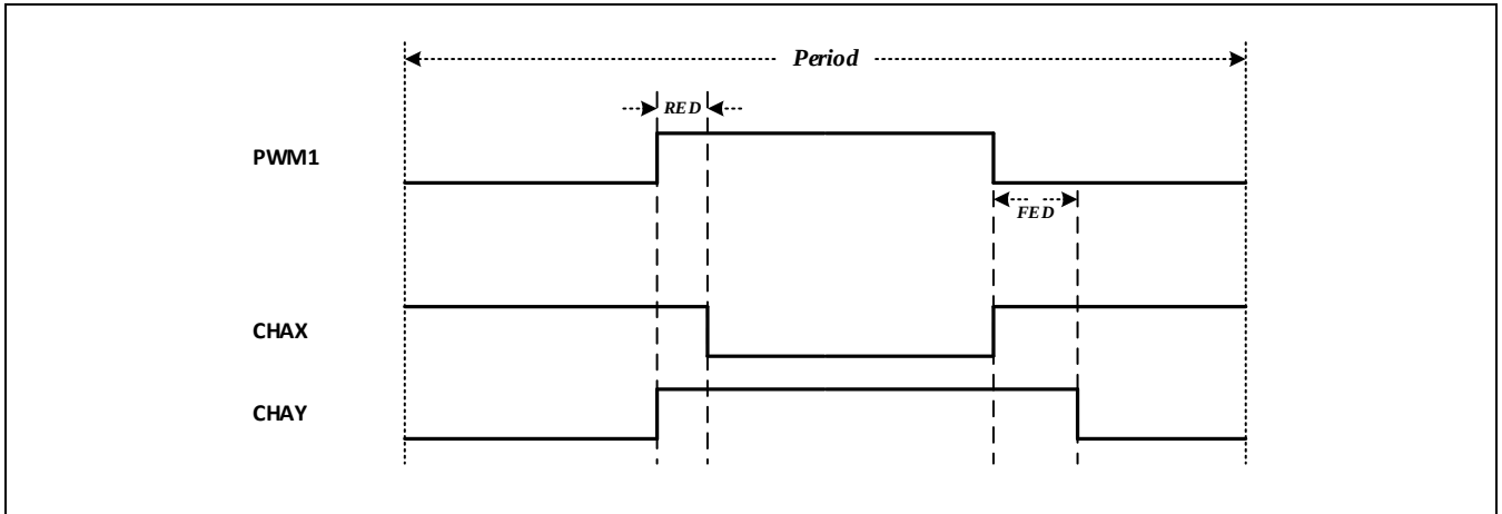
Figure 11-18 模式2：高电平有效的死区互补输出举例
