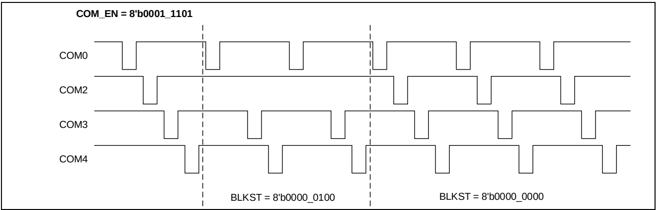
Figure 17-15 LED 闪烁的工作模式
