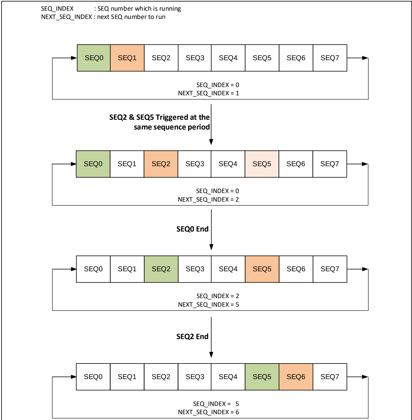
Figure 16-7 同时触发示意图
