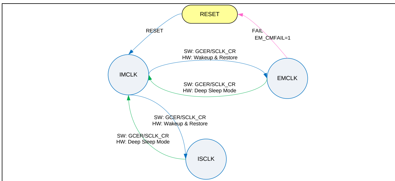
Figure 5-3 时钟切换状态机
