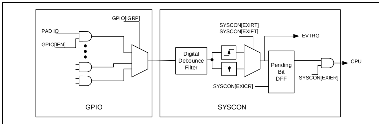
Figure 5-9 外部中断结构示意图
