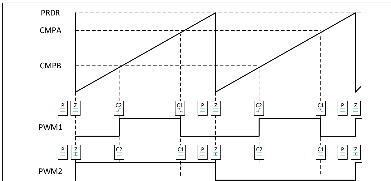
Figure 11-13 递增，脉冲定位非对称波形输出
