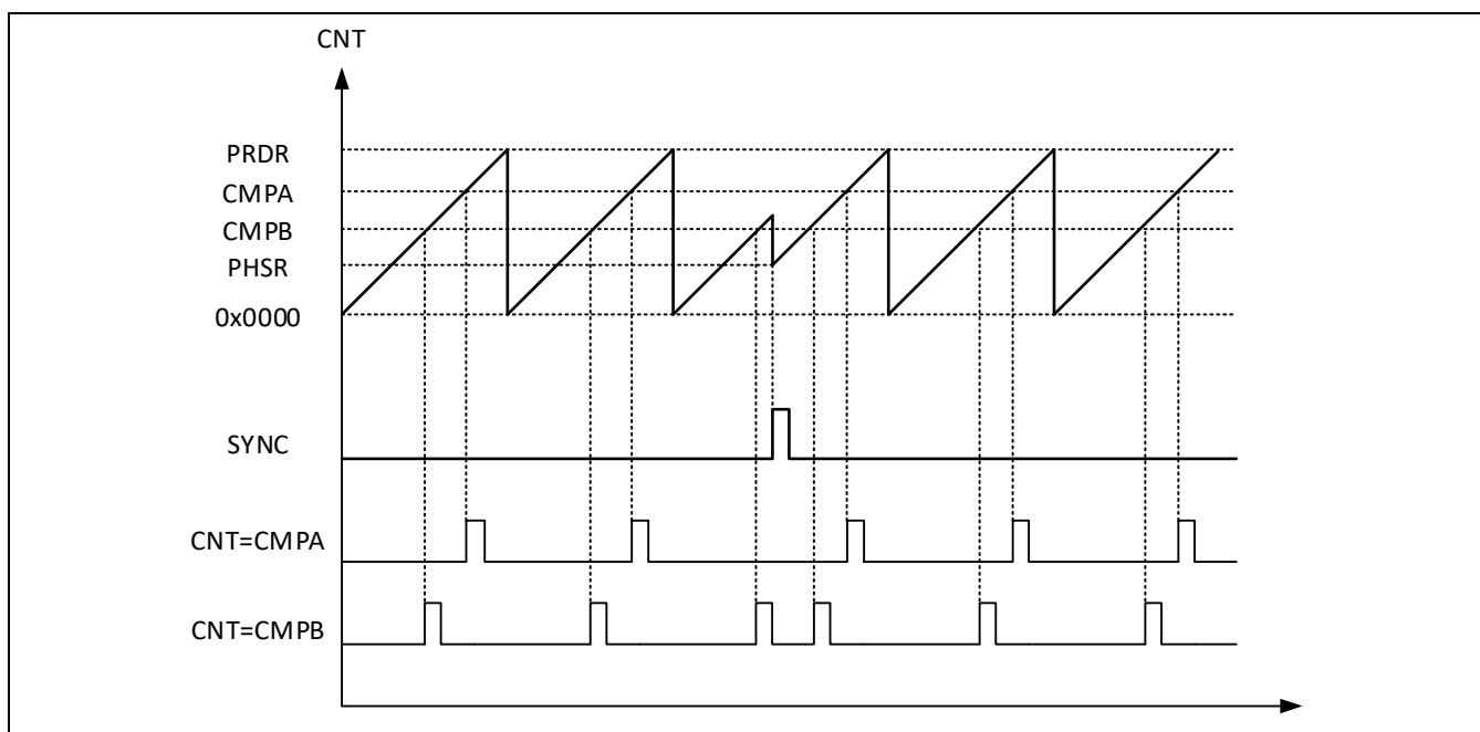
Figure 10-9 递增模式下比较事件产生时序
