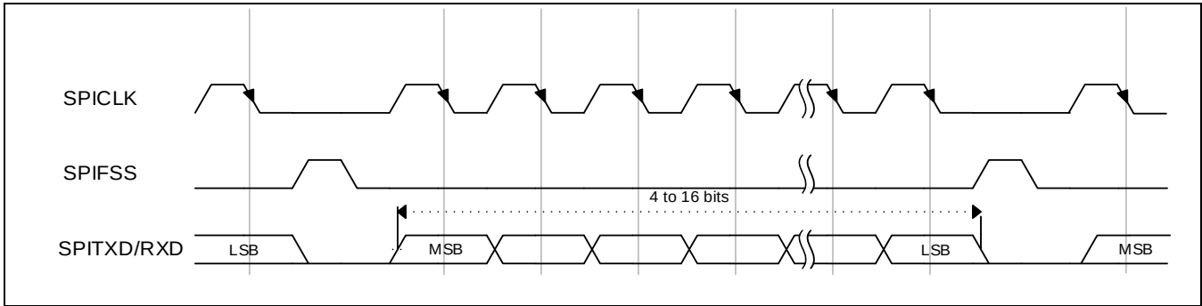
Figure 14-8 Motorola SPI 帧格式（连续传输）， SPO = 0 和 SPH = 1
