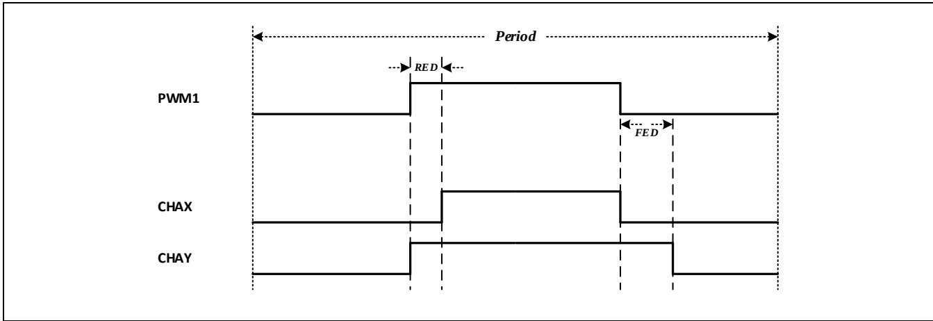
Figure 11-20 模式4：高低电平有效死区输出举例
