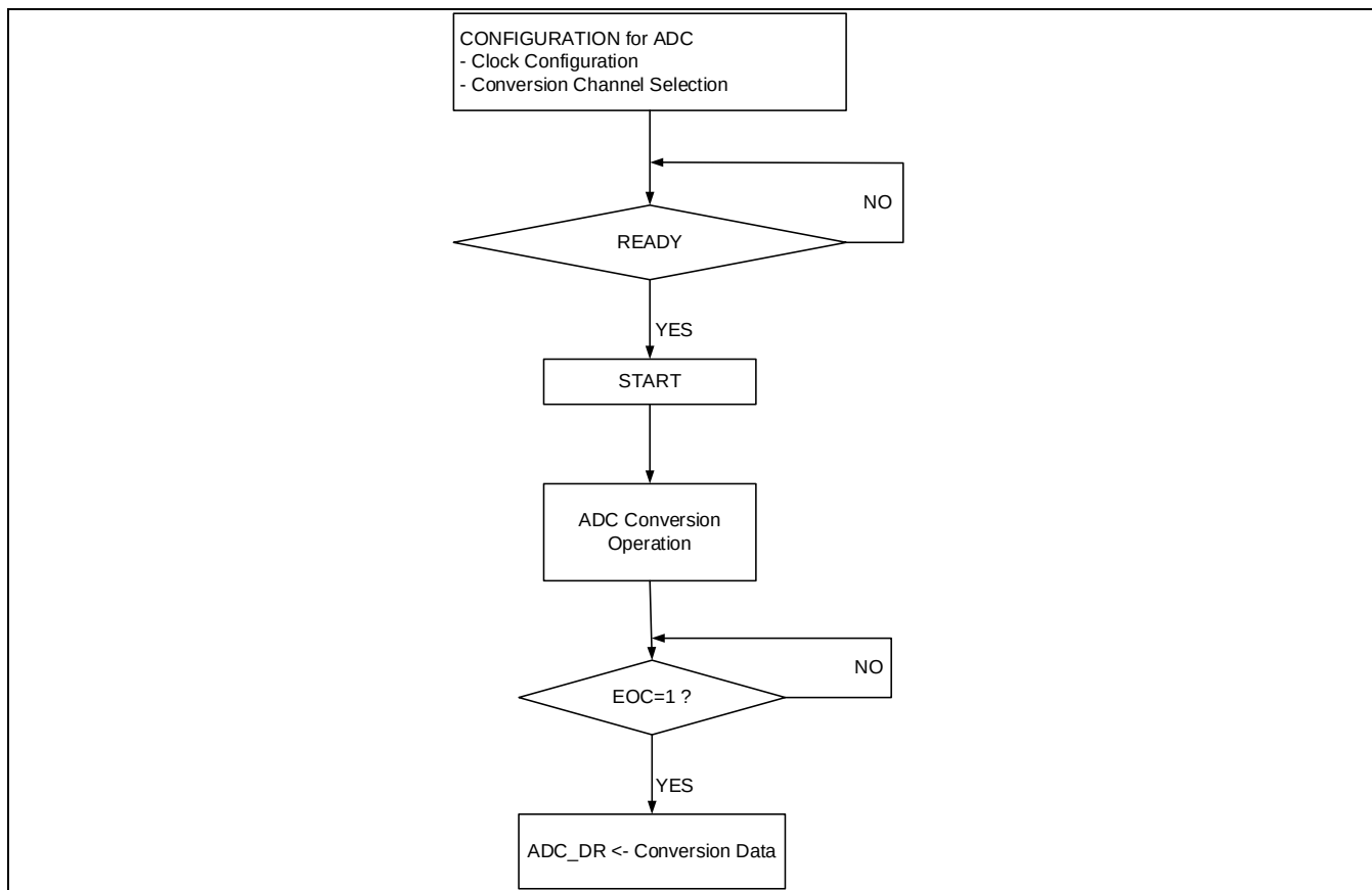
Figure 16-9 ADC工作流程图
