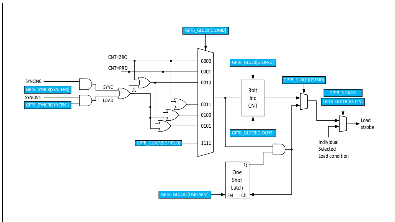
Figure 11-8 全局载入控制
