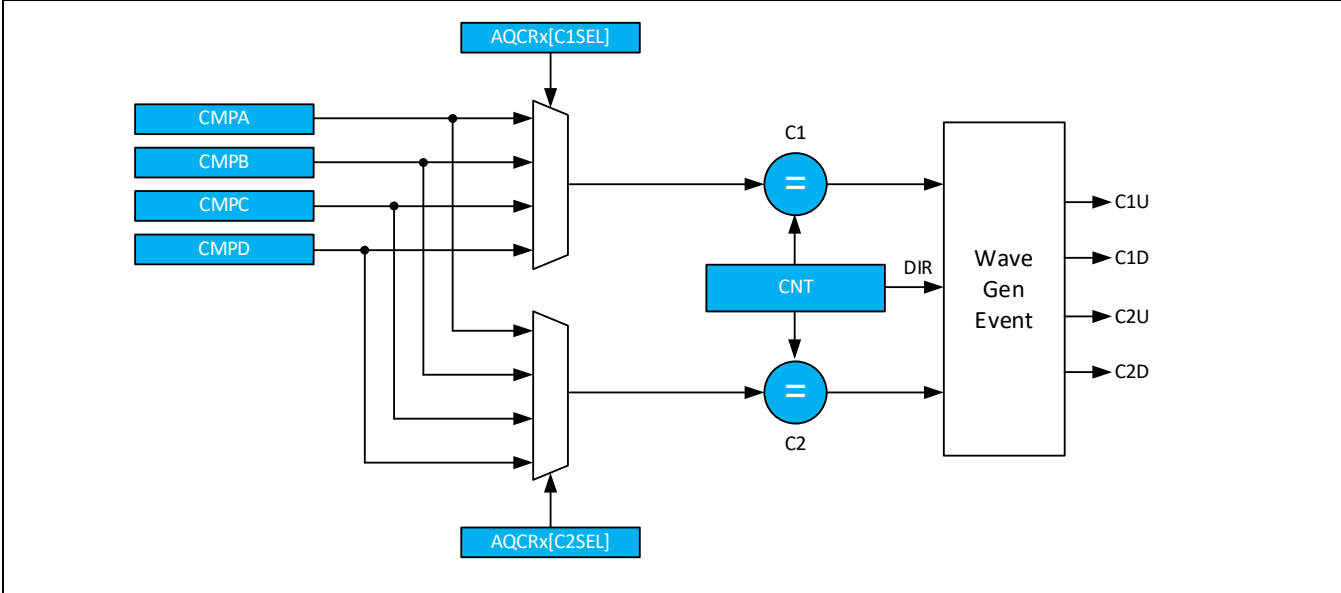
Figure 11-11 C1和C2选择控制
