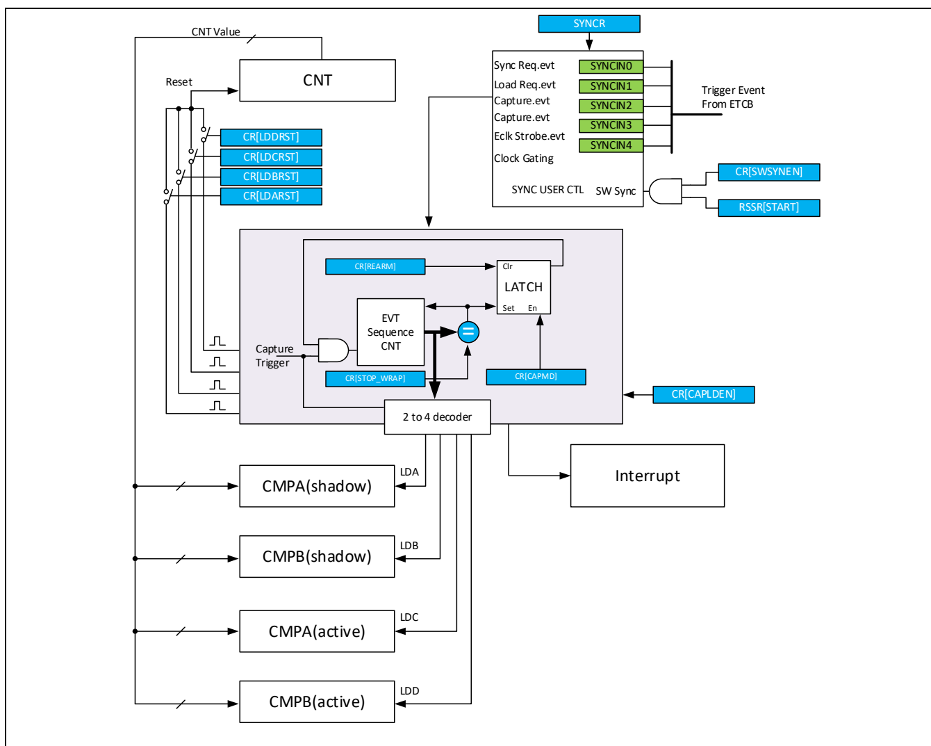
Figure 10-12 捕捉模式结构框图
