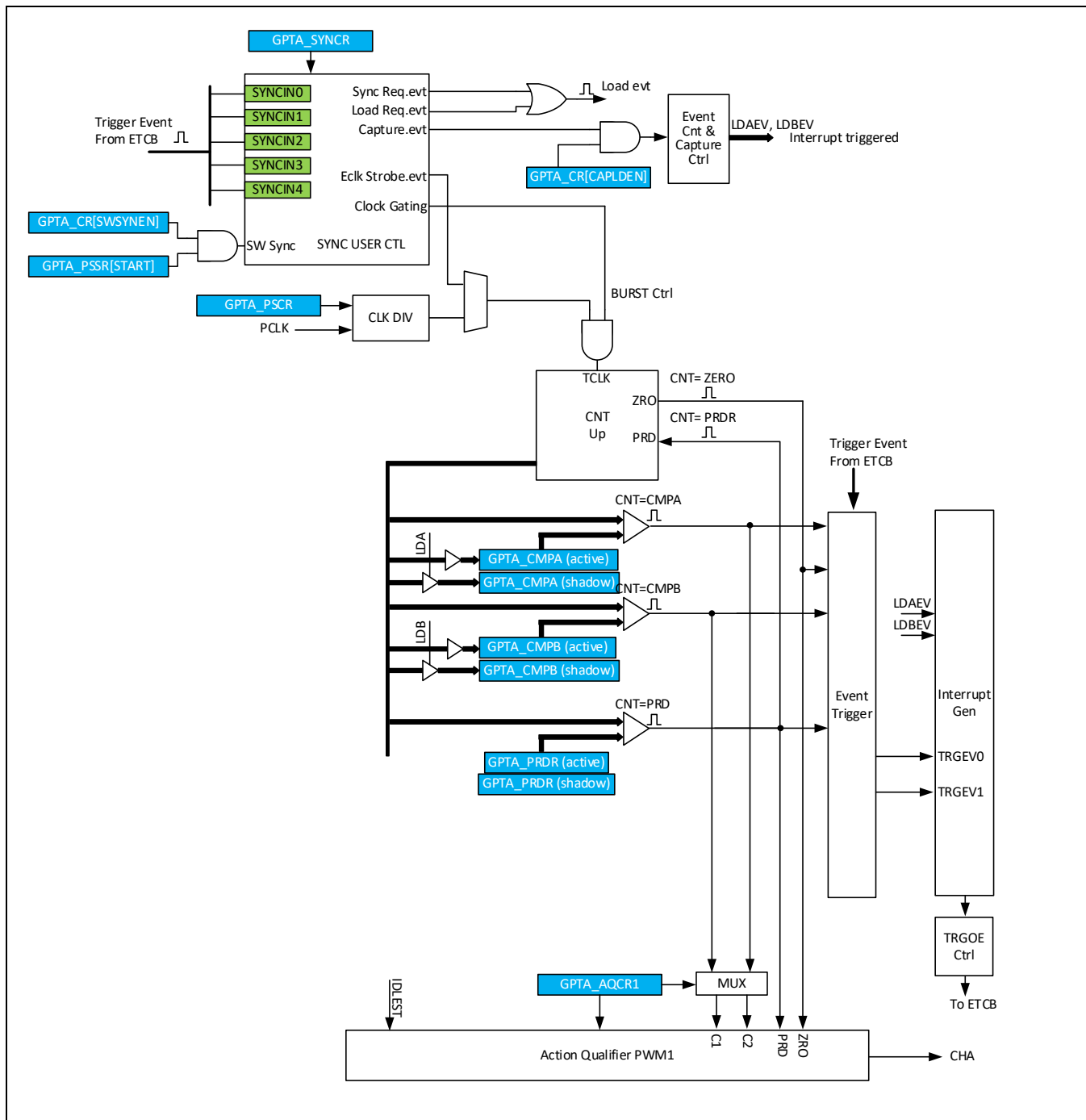
Figure 10-1 模块结构示意图
