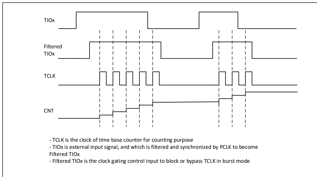
Figure 10-3 群脉冲时钟模式时序
