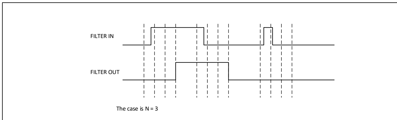
Figure 10-4 CG Filter 数字滤波器的原理
