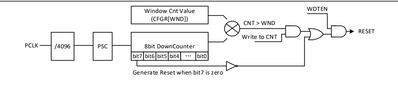
Figure 12-1 模块结构示意图
