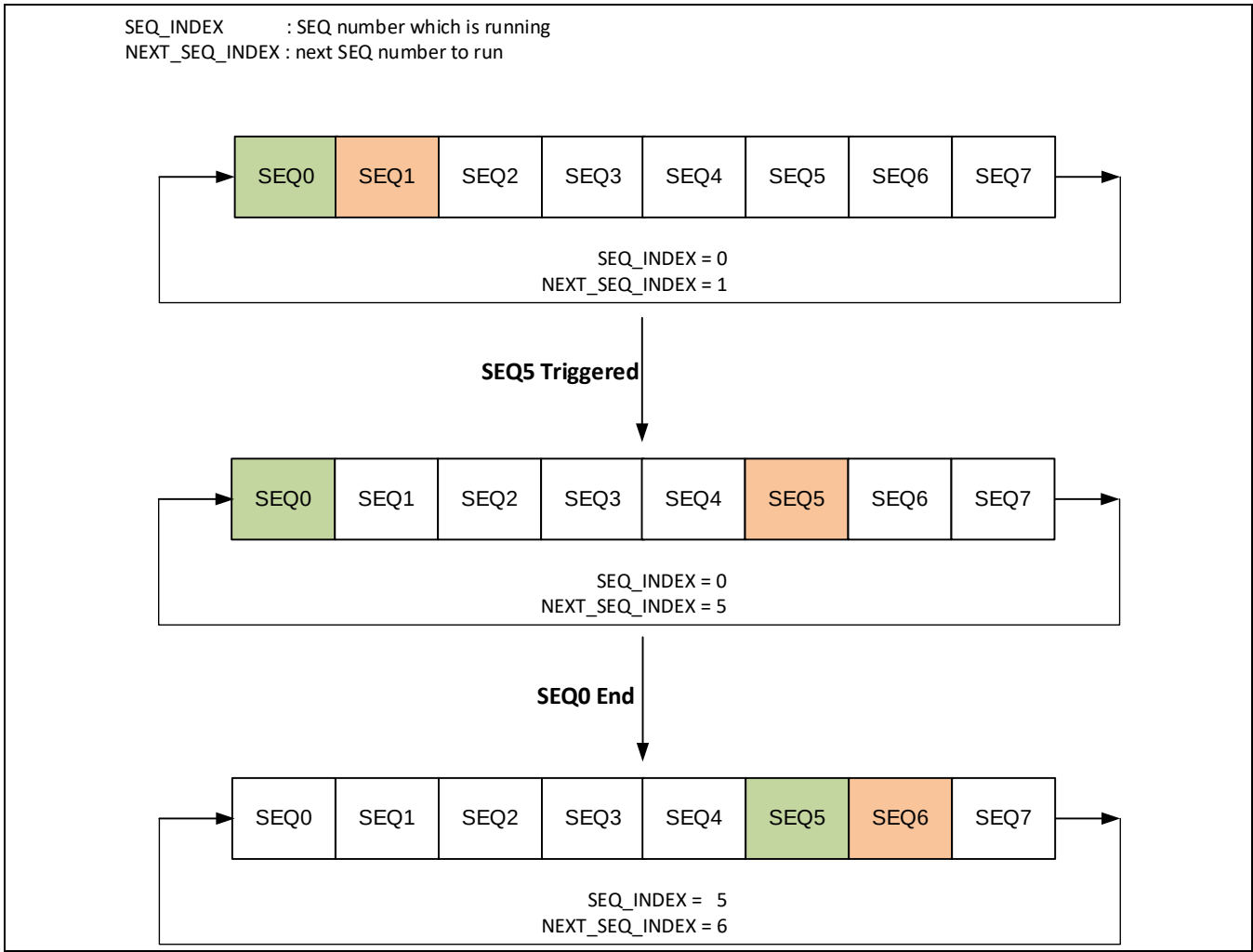
Figure 16-6 触发原理示意图
