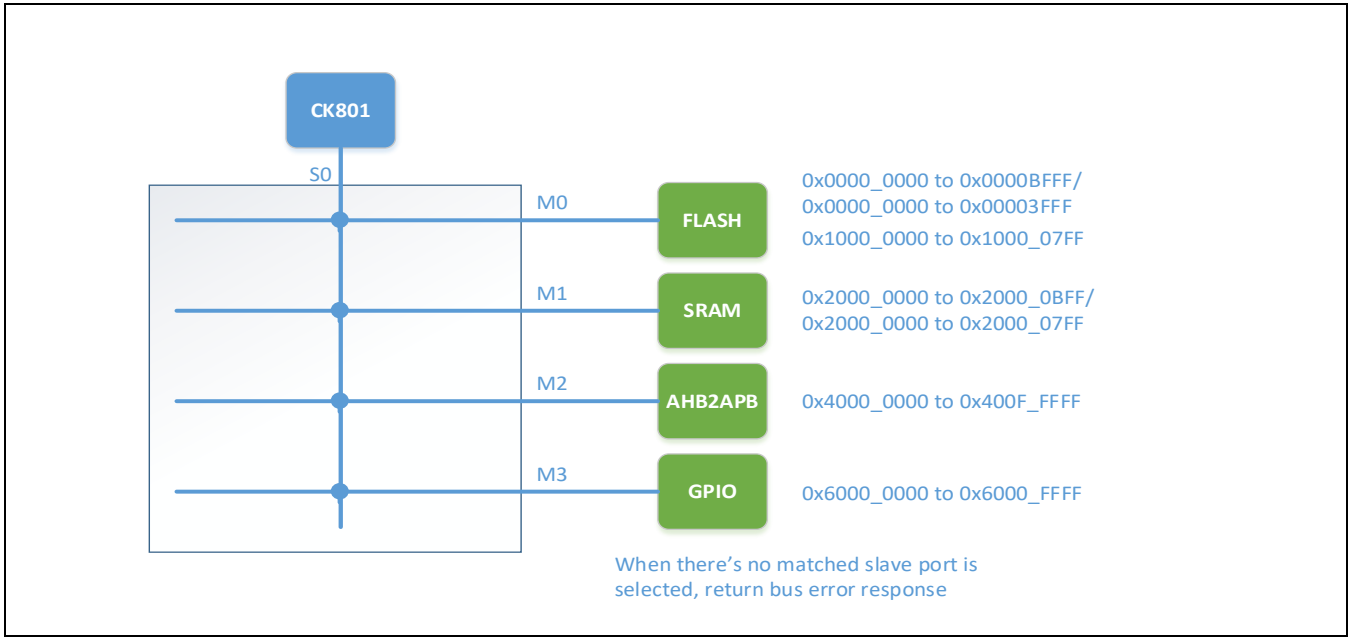
Figure 1-1 系统总线架构
