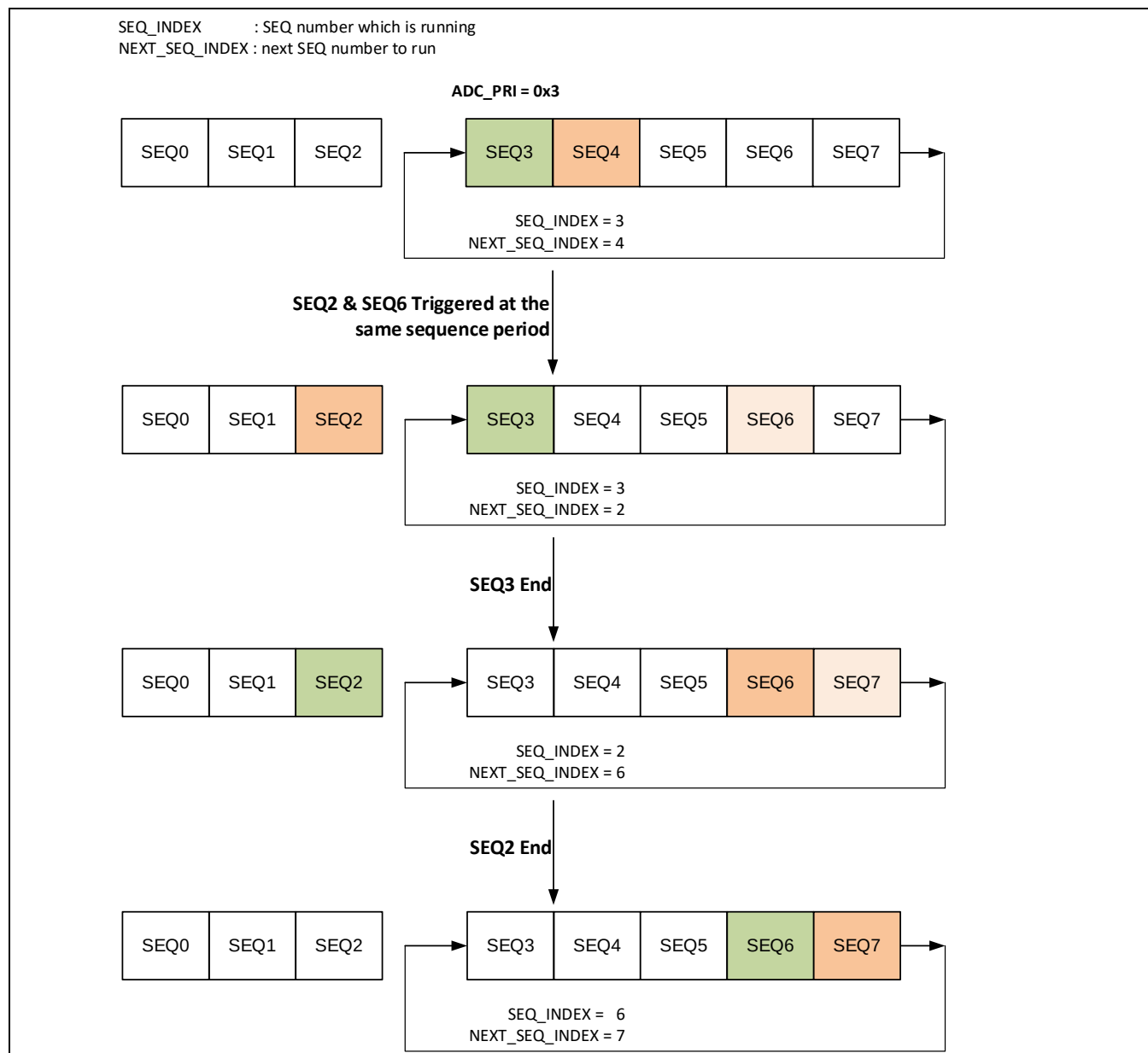
Figure 16-8 触发优先级示意图
