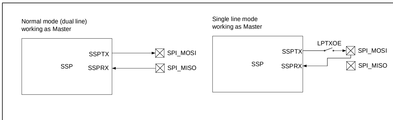
Figure 14-2 SPI 单线通讯模式
