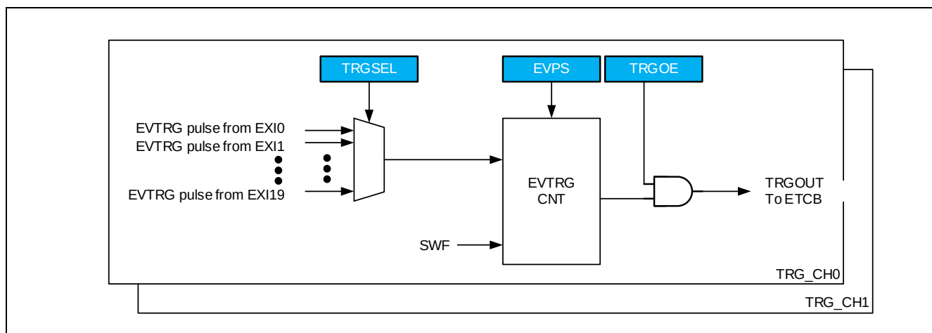
Figure 5-14 SYSCON 外部事件触发控制逻辑
