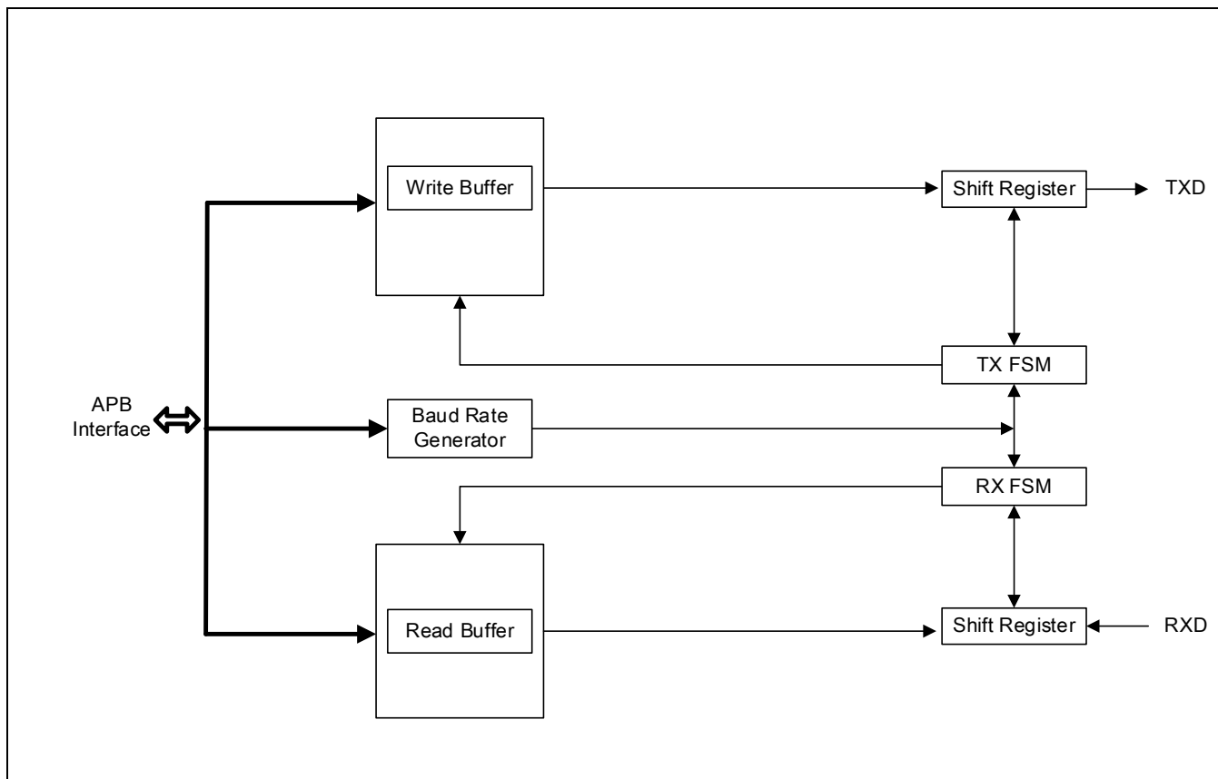
Figure 15-1 UART模块框图
