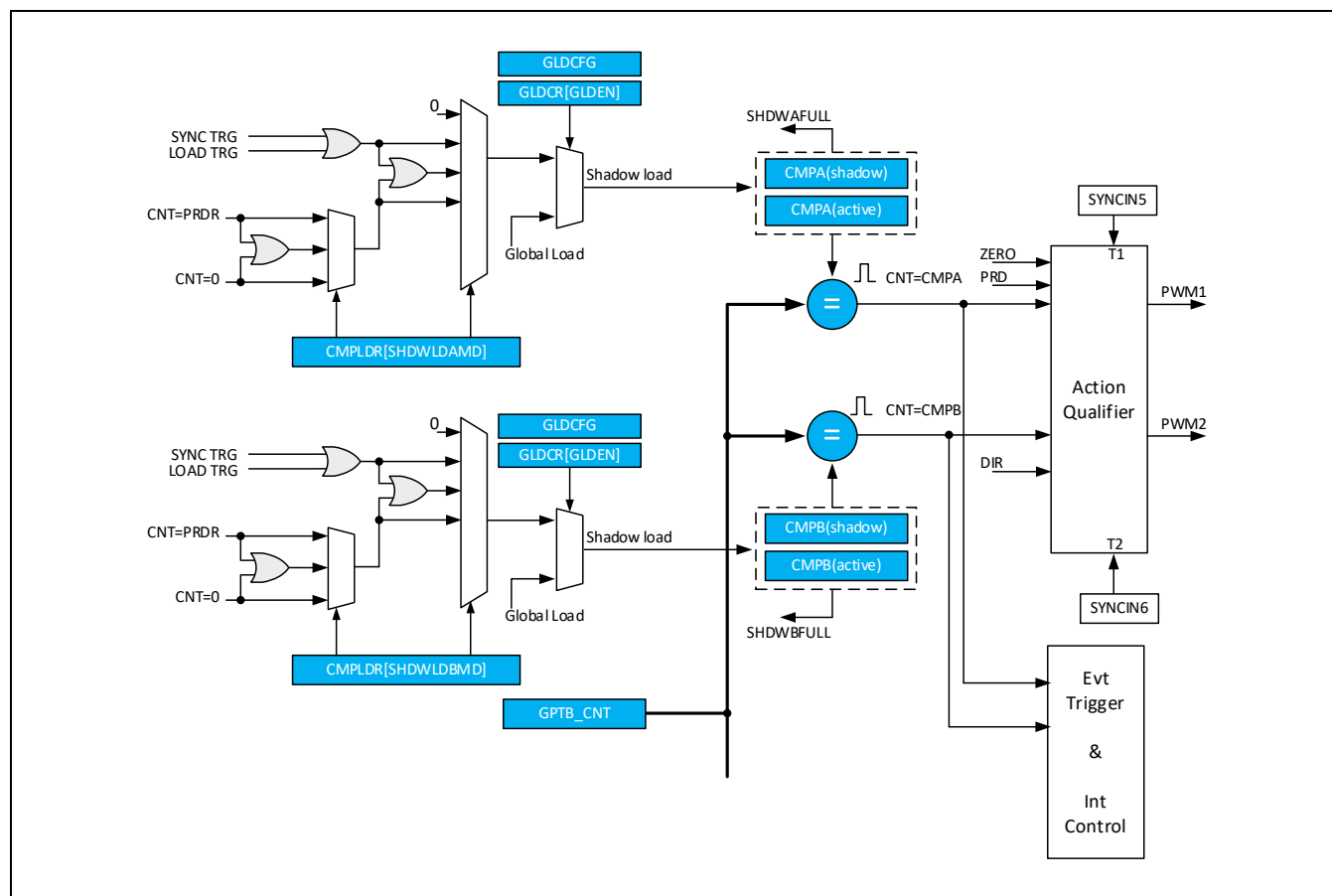
Figure 11-9 计数器值比较控制
