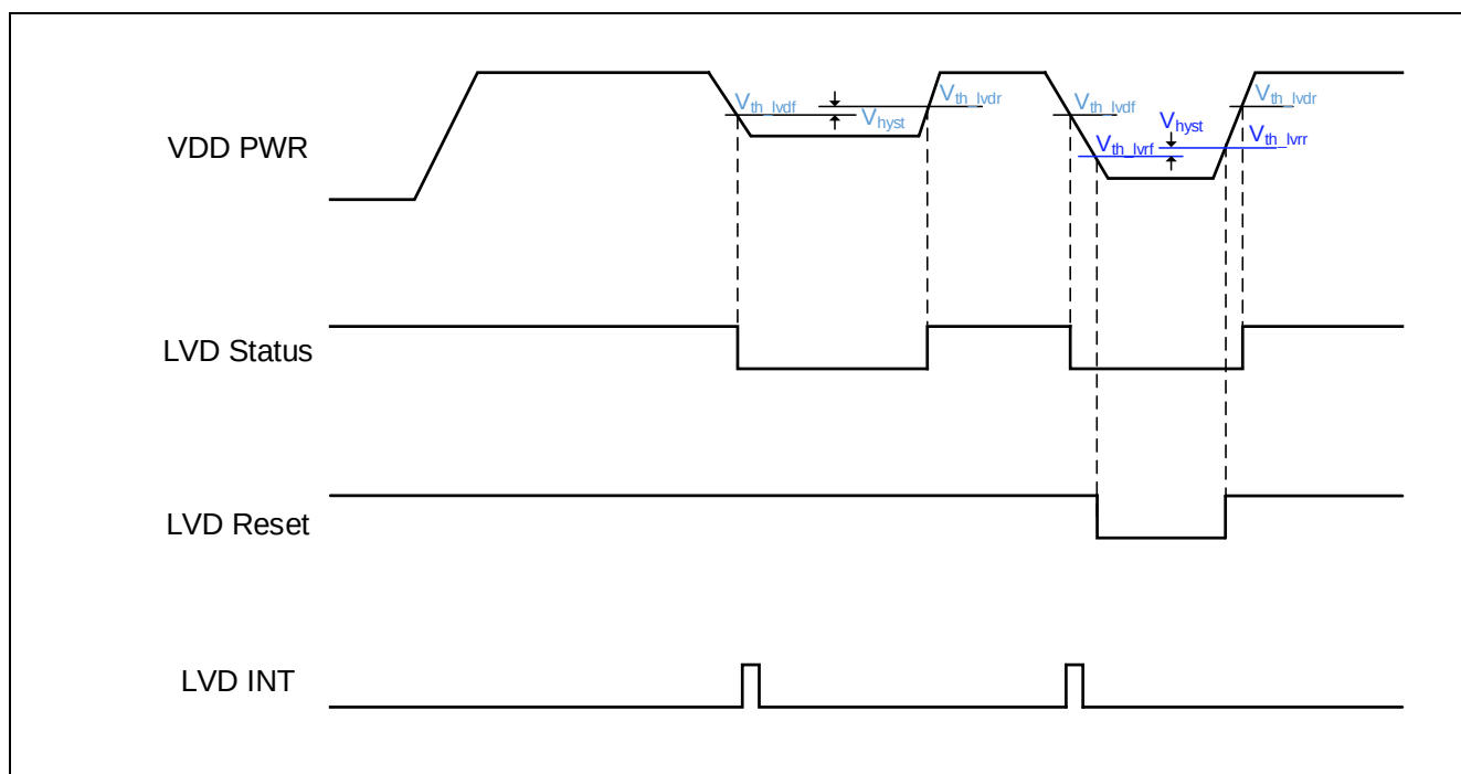
Figure 5-7 LVD 工作时序图
