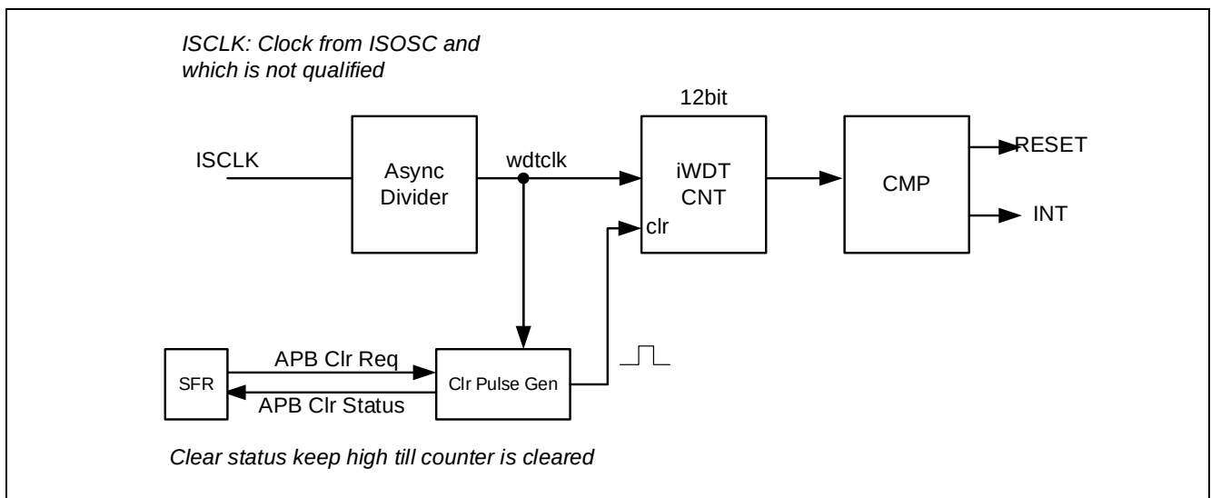
Figure 5-10 IWDT 结构框图
