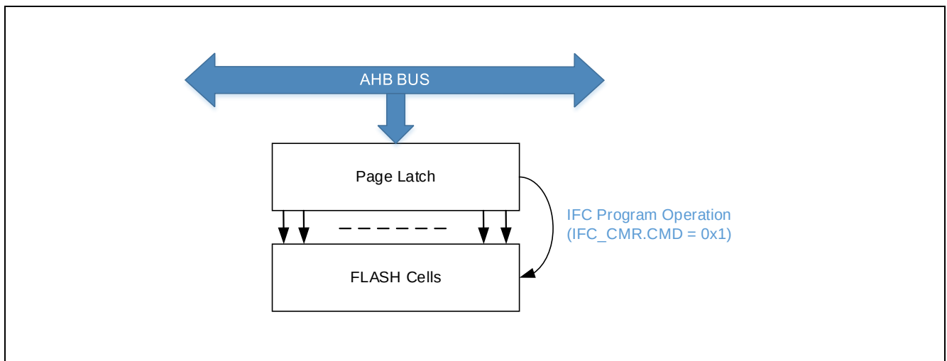
Figure 4-4 将页缓存数据写入闪存中
