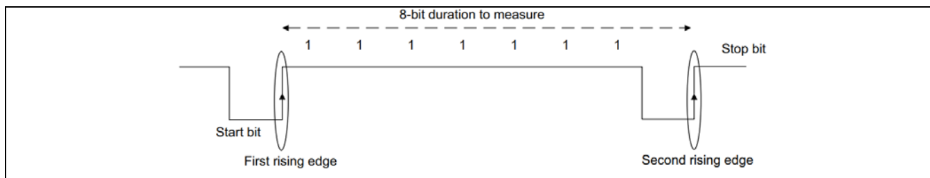
Figure 15-2 自动波特率原理
