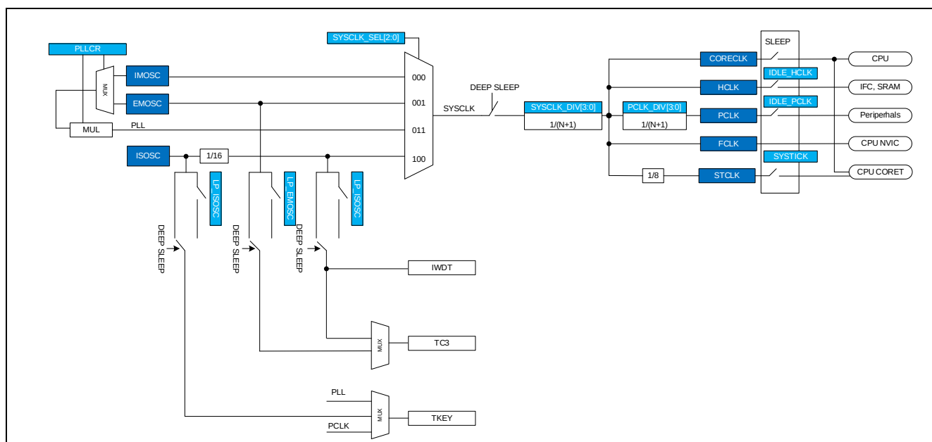
Figure 5-1 时钟结构示意图
