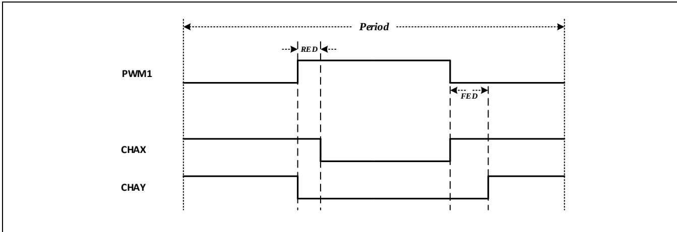
Figure 11-21 模式5：低高电平有效死区输出举例
