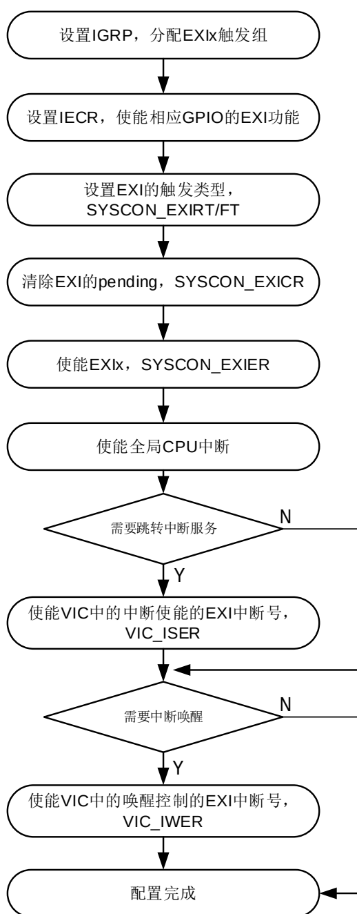
Figure 6-3 GPIO外部中断配置流程
