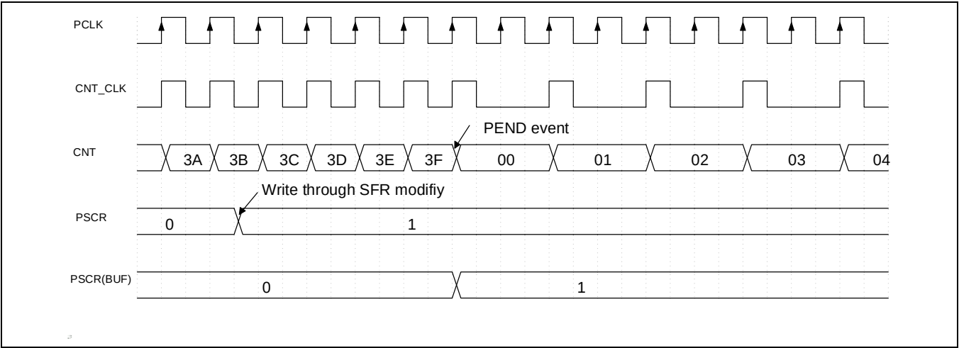
Figure 8-2 BT 周期计数模式
