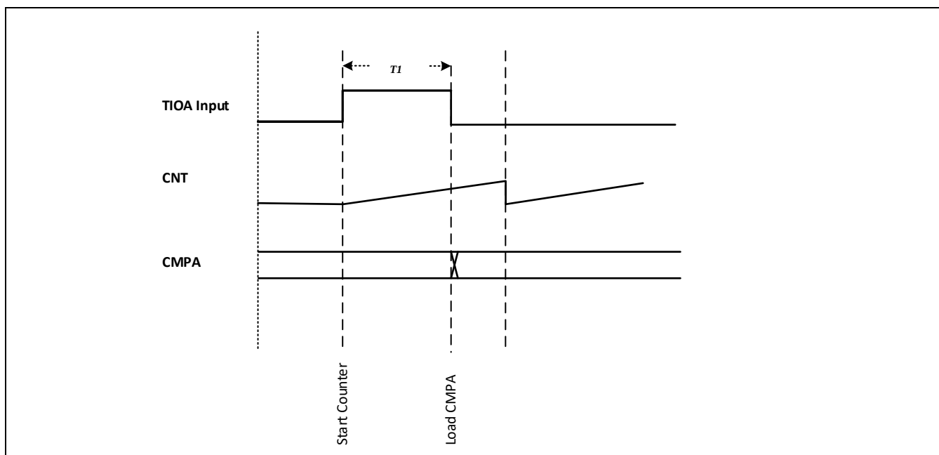
Figure 10-14 测量TIOA的脉冲宽度
