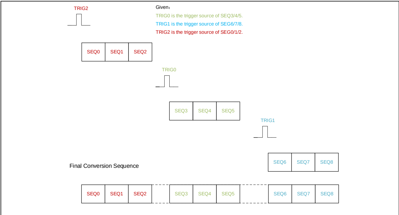
Figure 16-5 等待模式 ADC 工作时序图
