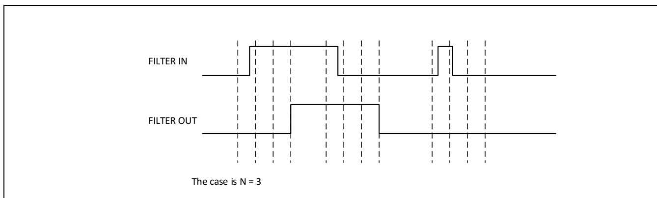
Figure 11-4 CG Filter 数字滤波器的原理
