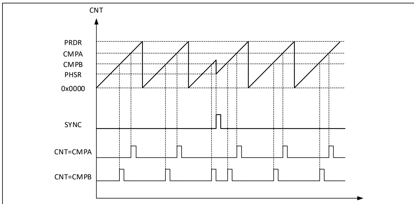
Figure 11-10 递增模式下比较事件产生时序
