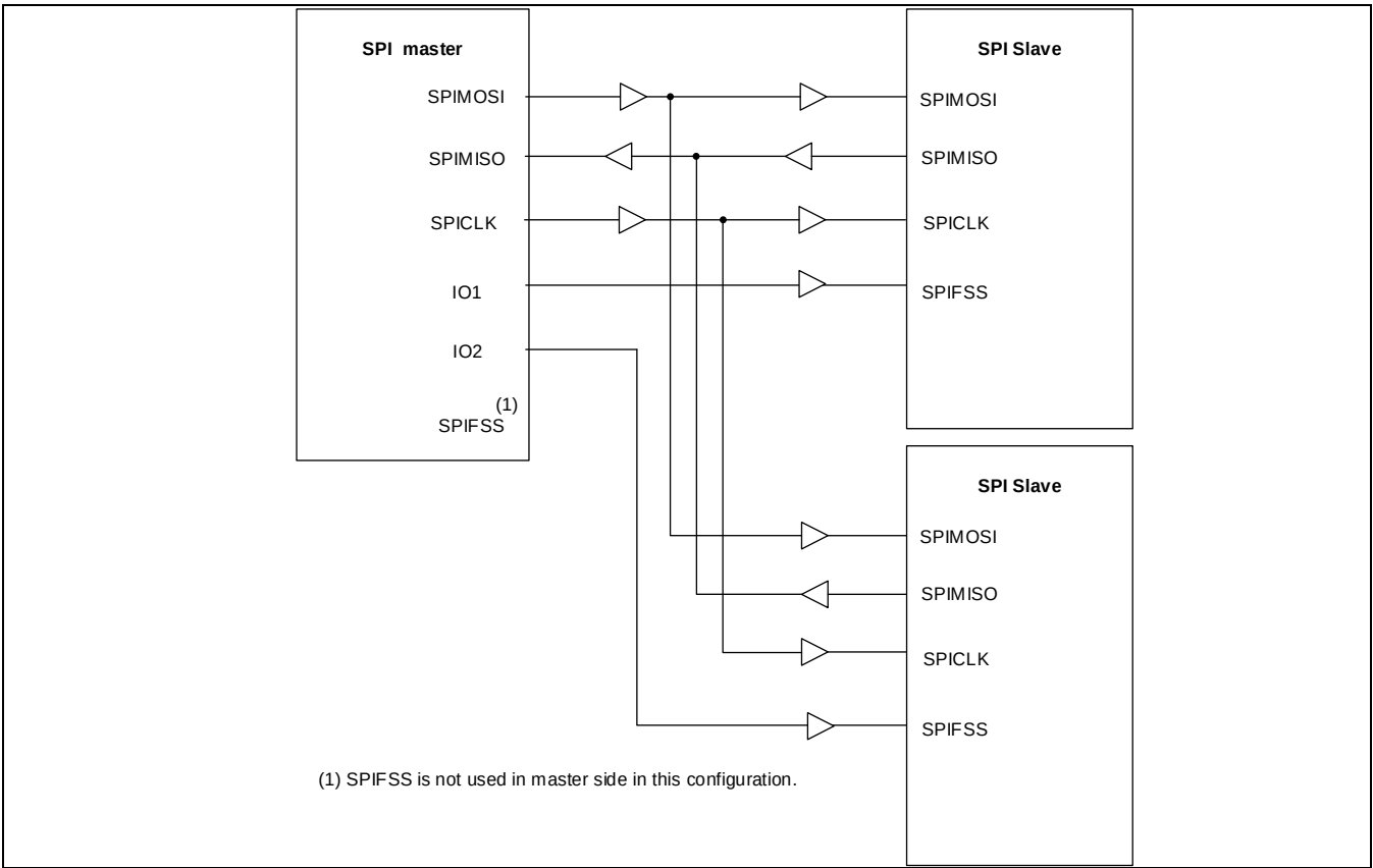
Figure 14-4 SPI 主机连接到两个SPI从机
