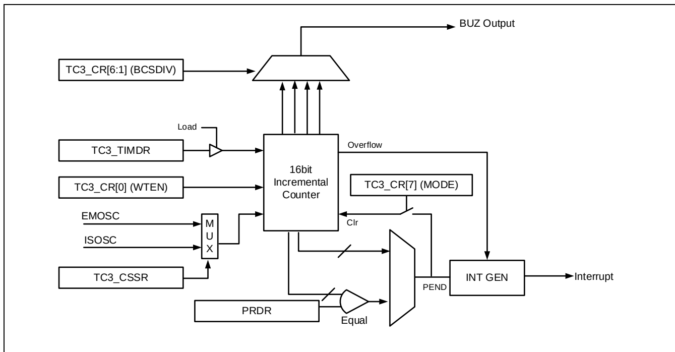
Figure 9-1 时钟定时器模块框图
