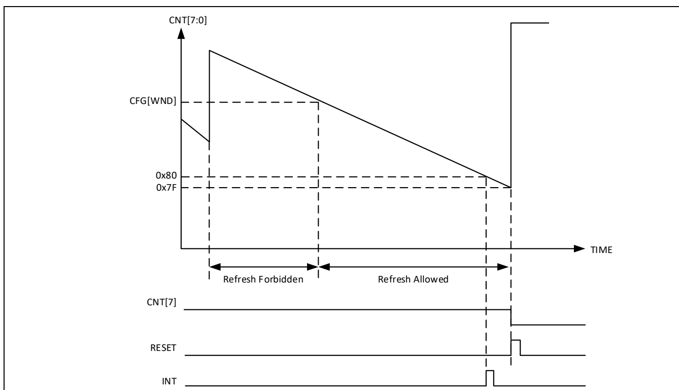
Figure 12-2 计数器工作示例
