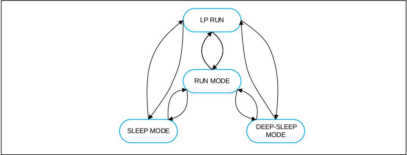
Figure 5-8 模式切换示意图
