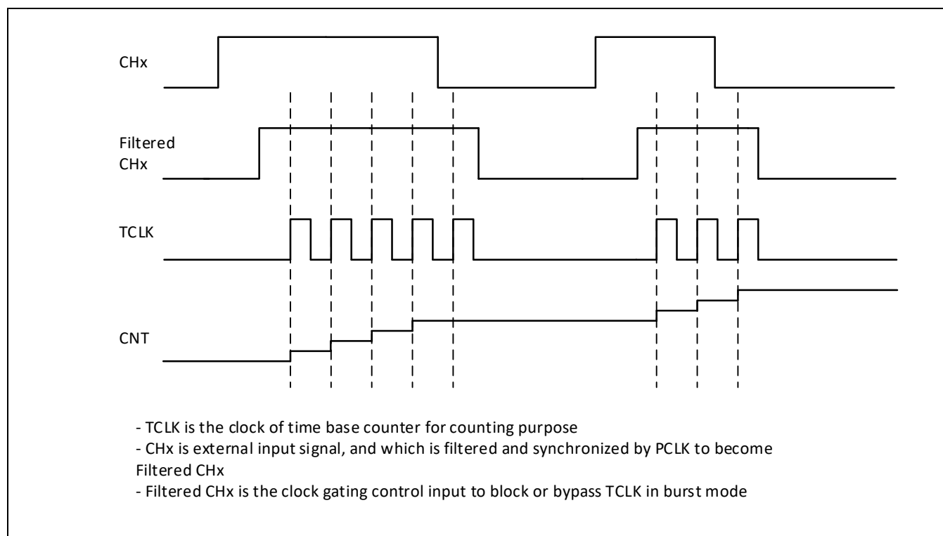
Figure 11-3 群脉冲时钟模式时序
