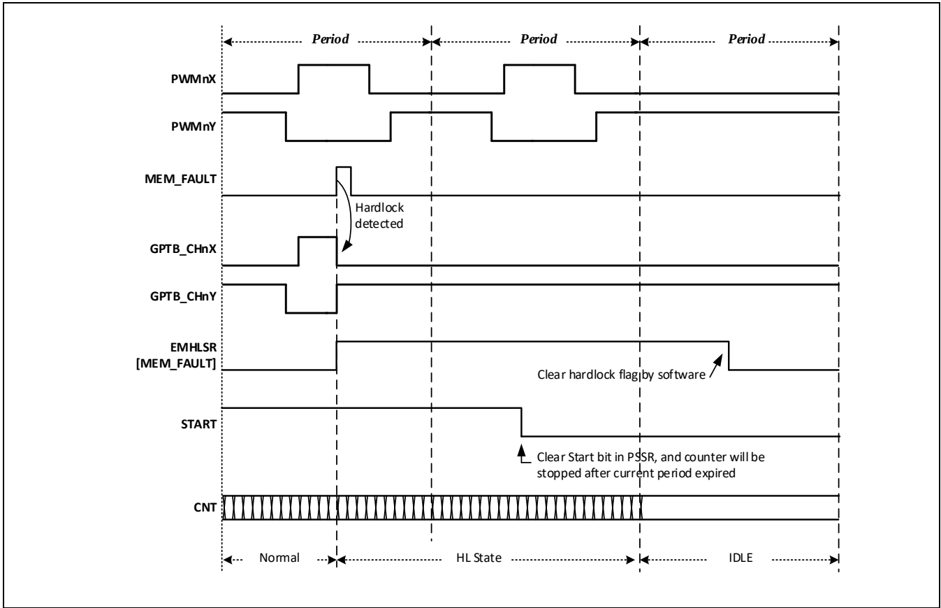
Figure 11-24 硬锁止模式
