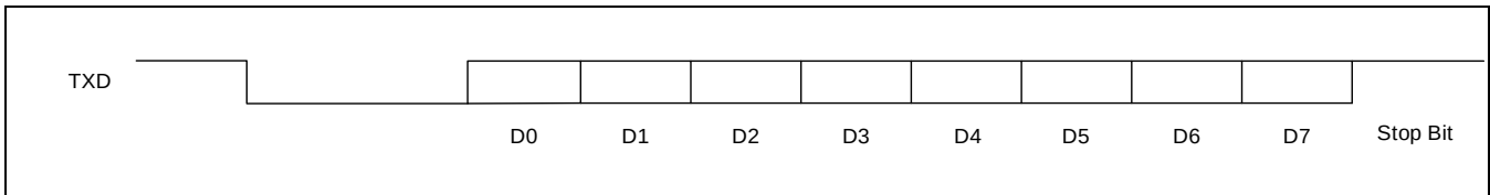
Figure 15-5 数据发送
