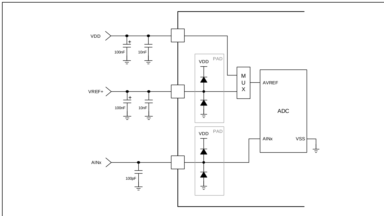
Figure 16-2 参考电路
