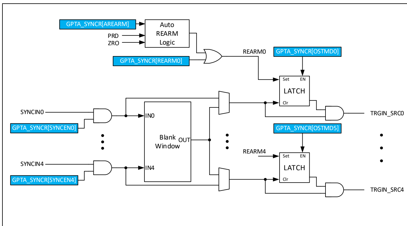
Figure 10-16 同步触发输入
