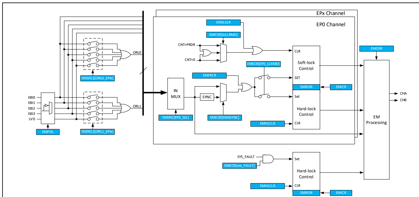
Figure 11-22 紧急模式控制模块
