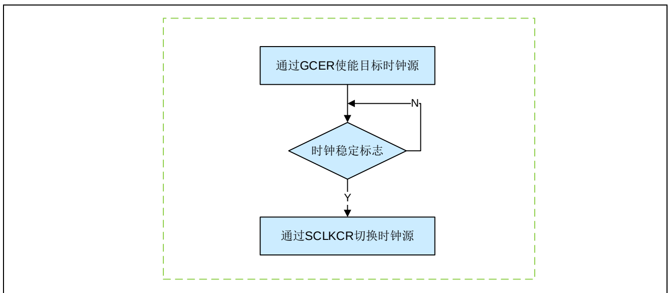
Figure 5-2 时钟源切换示意图
