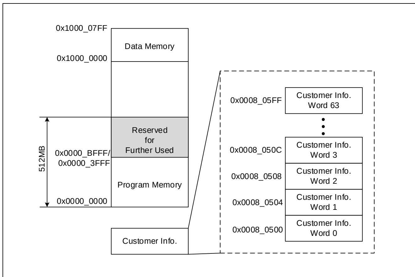
Figure 4-2 闪存地址空间结构
