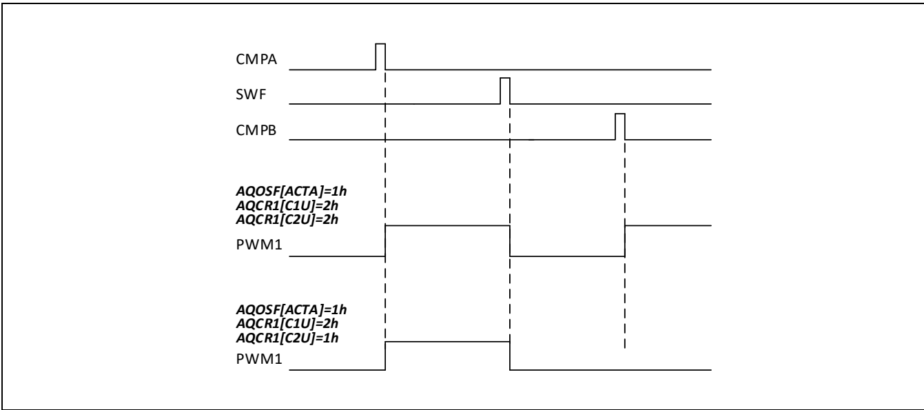
Figure 11-14 一次性软件强制输出
