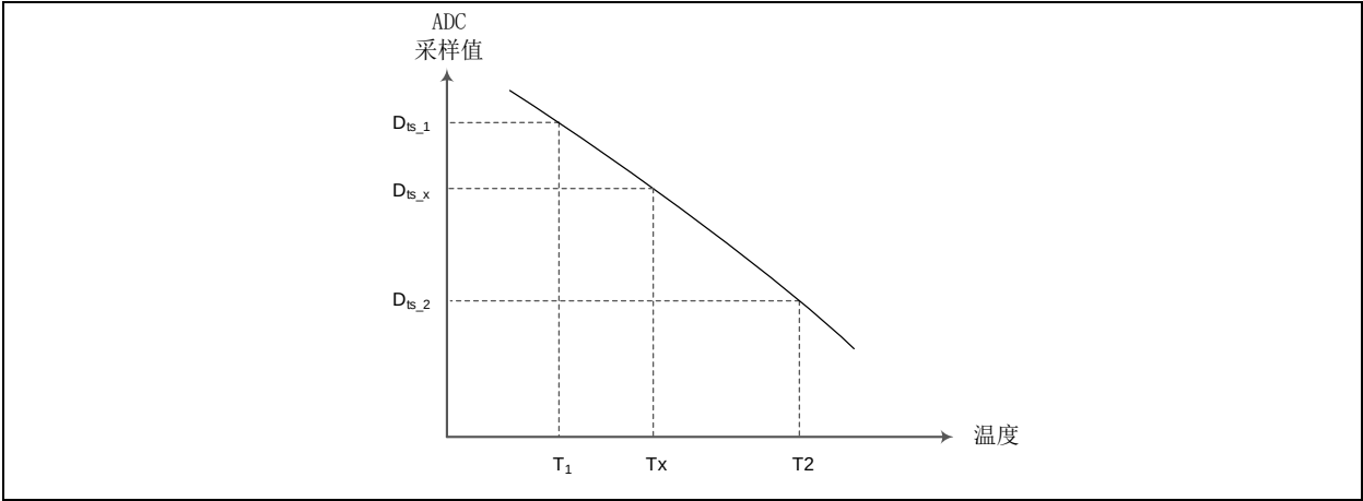
Figure 16-10 ADC采样内部温度传感器
