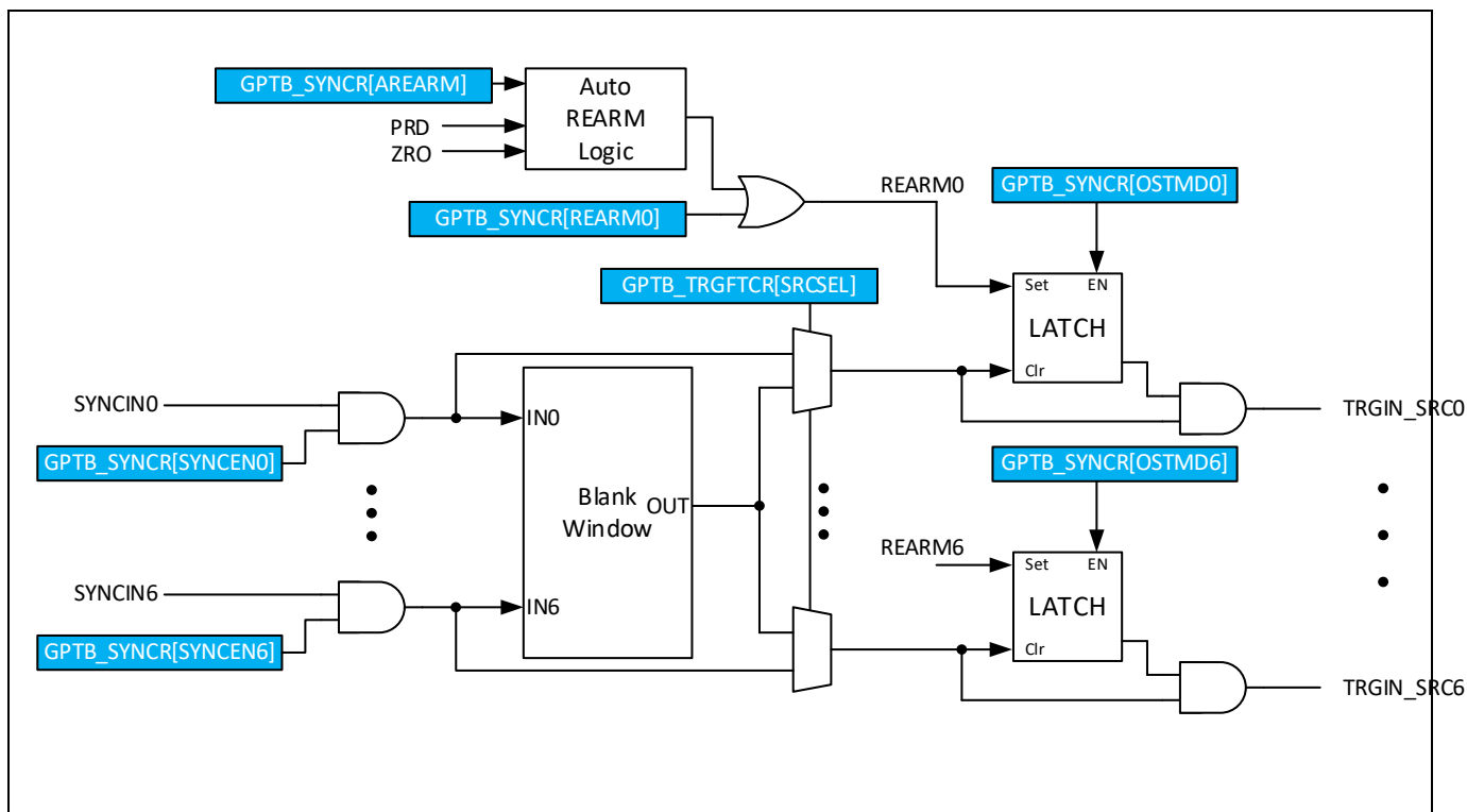
Figure 11-30 同步触发输入
